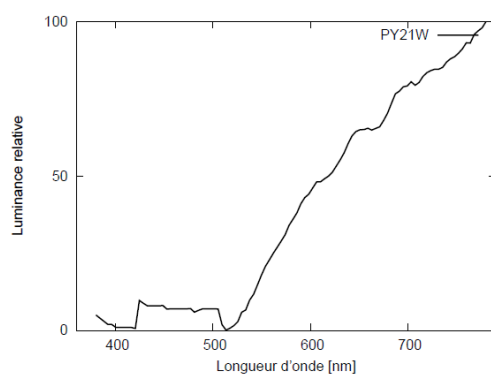
(a) Lampe à incandescence teintée - extrait de [Alb04]
