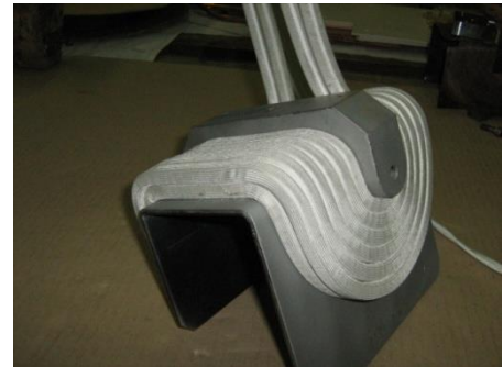
Figure 1.7: Inducteur enveloppant en cours de fabrication (Fives Celes)
