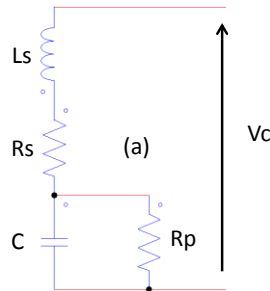
Figure 1.51: Modélisation des condensateurs pour le calcul des pertes
