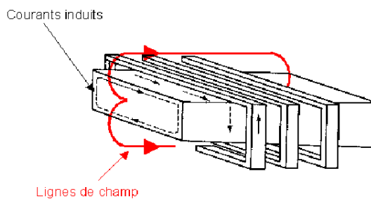
Inducteur à flux longitudinal
