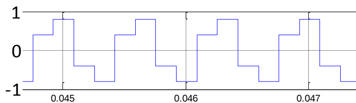
Figure 3.11: Forme générale des signaux de commande U , modulés en amplitude
