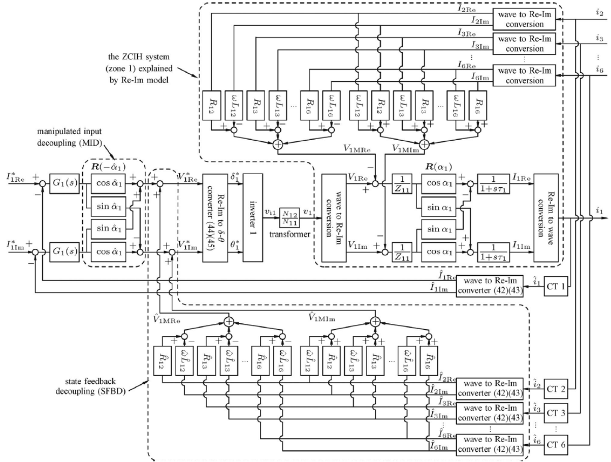
Figure 2.33: Schéma général de la commande des courants en valeurs réelles et imaginaires [33]
