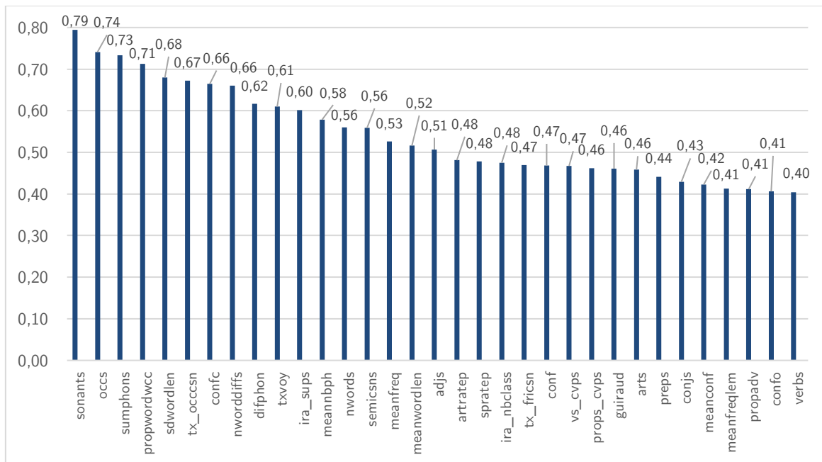
Figure 30 - Analyses bivariées entre le score holistique de communication et les paramètres automatiques dont les coefficients de corrélation de Spearman sont significatifs au seuil de 5 %.
