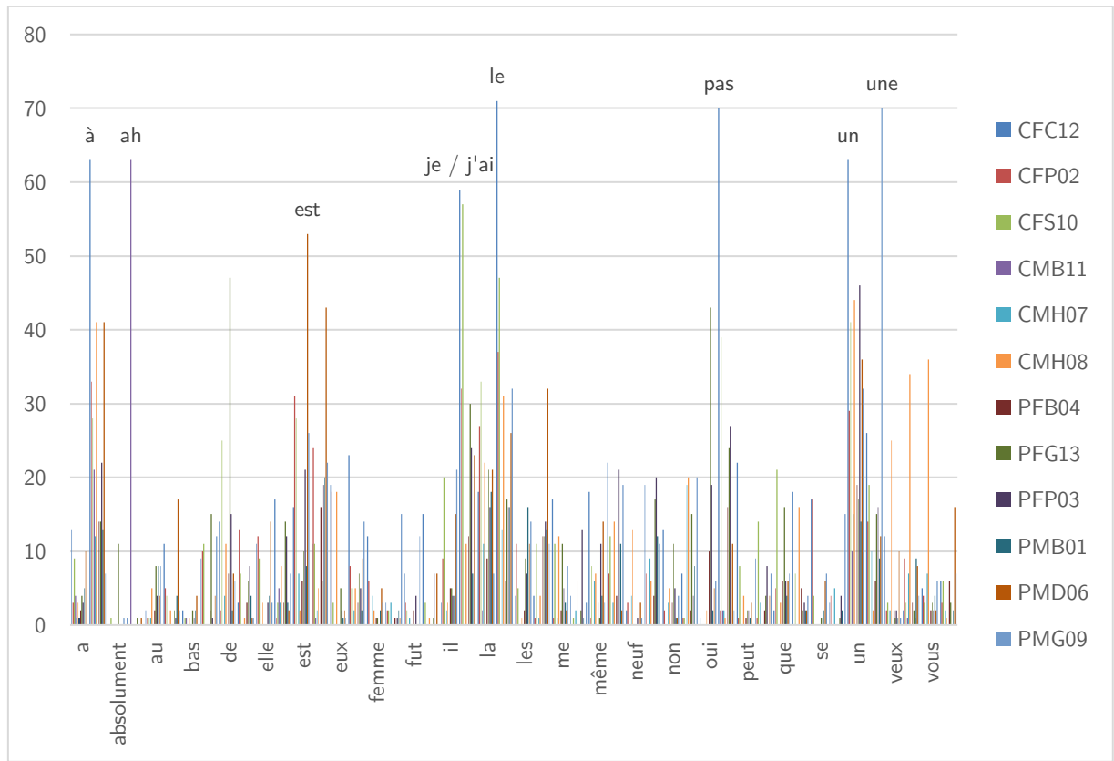
Figure 21 - Représentation des mots ayant au moins dix occurrences chez au moins un des sujets (les mots ayant au moins 50 occurrences ont été étiquetés)
