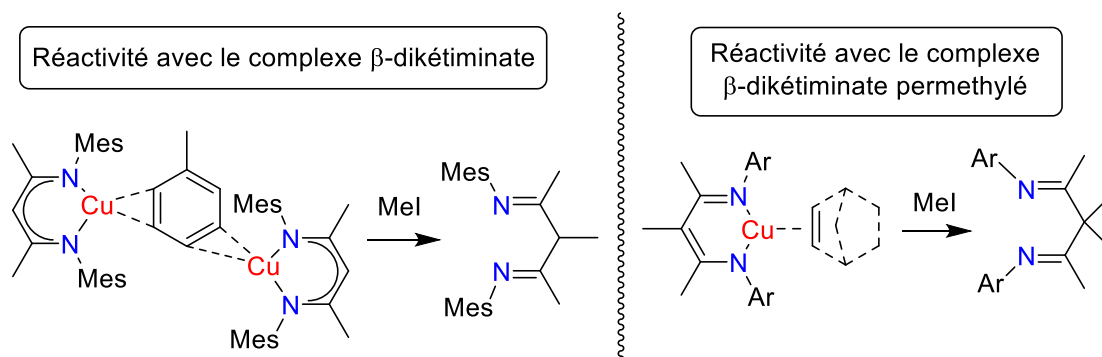
Schéma 5 : Réactivités observées des complexes \beta -dikétiminates de cuivre(I) et \beta -dikétiminates protégés de cuivre(I).
