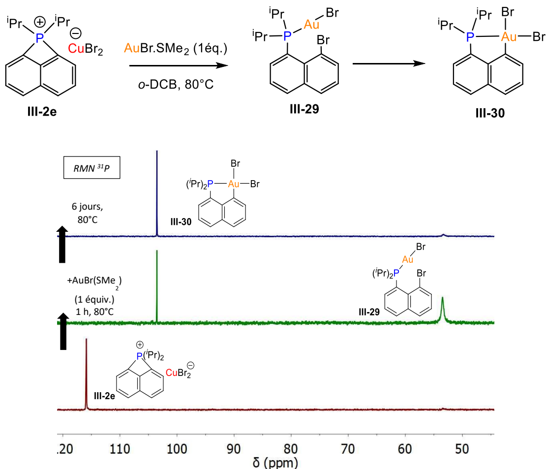
Schéma 23 : Réactivité du phosphonium III-2e avec \text{AuBr} \cdot \text{SMe}_2 (au-dessus). Spectres montrant la formation de l'intermédiaire III-29 (en-dessous).
