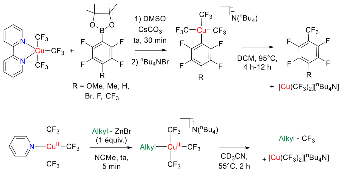
Schéma 39 : Synthèse des espèces \text{Ar-Cu}^{\text{III}} et élimination réductrice (réaction du dessus). Formation des espèces \text{Alk-Cu}^{\text{III}} et élimination réductrice (réaction du dessous)
