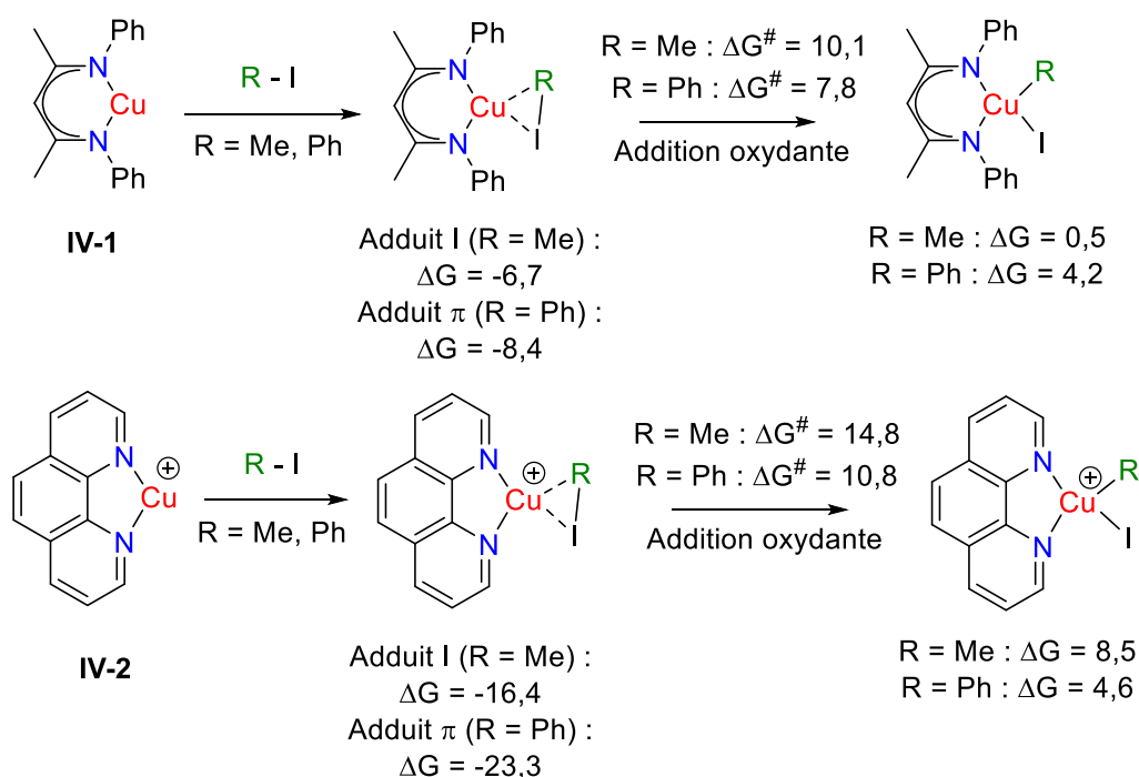
Schéma 4 : Calculs DFT au niveau de théorie (B97D/SDD+f(Cu),6-31G**(autres atomes)) pour l'addition oxydante de l'iodométhane et de l'iodobenzène sur les complexes dicoordinés de Cu(I) ( \Delta G en kcal/mol).
