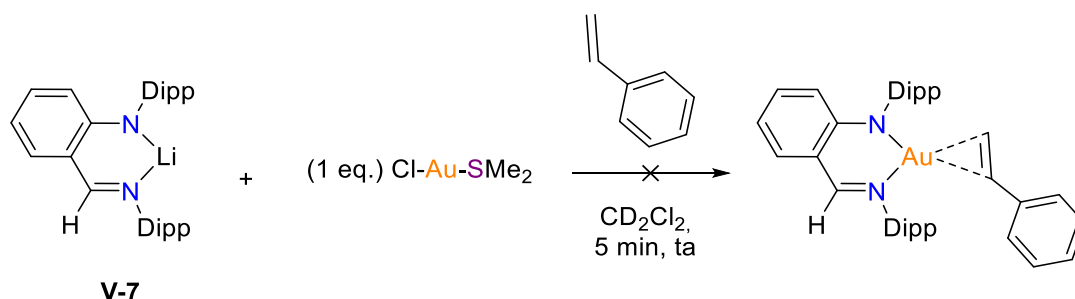
Schéma 20 : Complexation du lithien V-7 sur le \text{ClAuSMe}_2 en présence de styrène pour former un \pi -complexe d'or(I).
