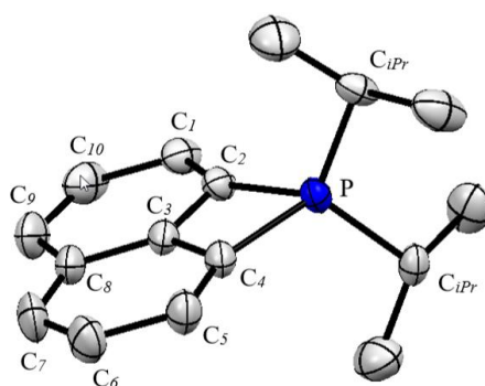
Schéma 6 : Structure cristallographique du phosphonium cyclique péri -ponté.
