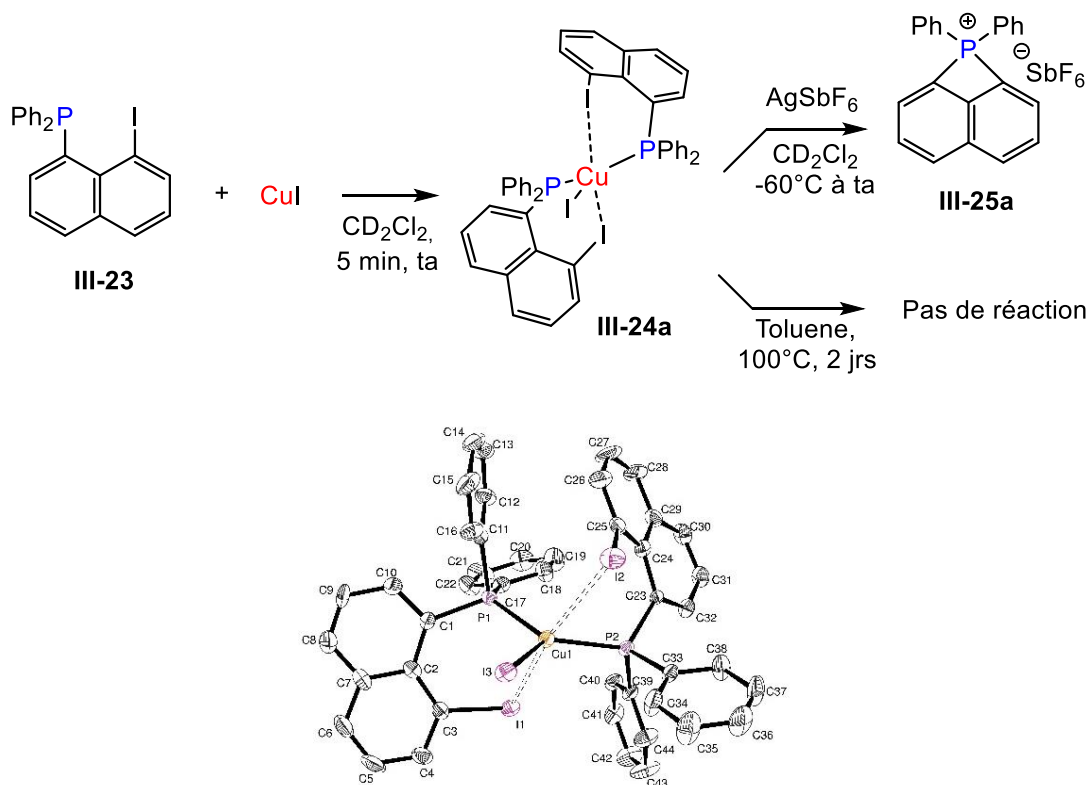
Schéma 15 : Réactivité de la phosphine III-23 avec le précurseur CuI (en haut). Structure cristallographique du composé III-24a (en bas).
