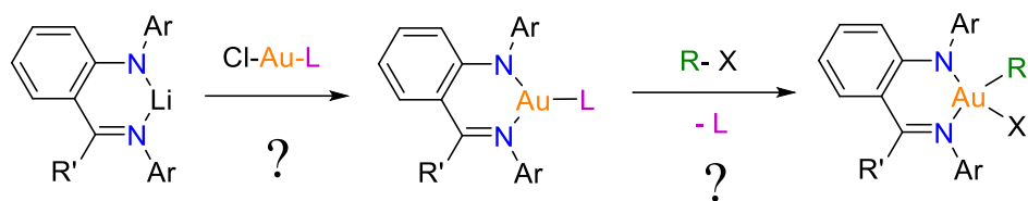
Schéma 15 : Stratégie envisagée et développée dans le chapitre V pour stabiliser des complexes d'or(I) et d'or(III).
