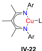
Complexe \beta -dikétiminate de cuivre(I) protection méthyle
