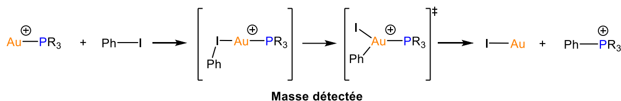
Schéma 8 : Couplage P-C aryle passant par l'intermédiaire d'un complexe d'or(III).
