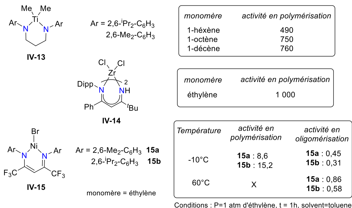
Schéma 9 : Exemples de pré-catalyseurs à ligands BDI (ou analogue) actifs en polymérisation/oligomérisation de \alpha -oléfines (activité en kg.mol[catalyseur] -1 .h -1 ).
