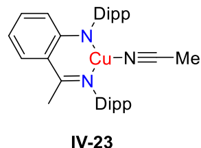
Schéma 13 : Complexes de cuivre(I) envisagés et possédant une protection du carbone en position \alpha .
