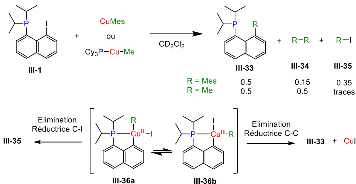
Schéma 27 : Mécanisme postulé pour la formation des produits de couplages entre le ligand péri-iodonaphthyl-phosphine III-1 et les organocuvires.
