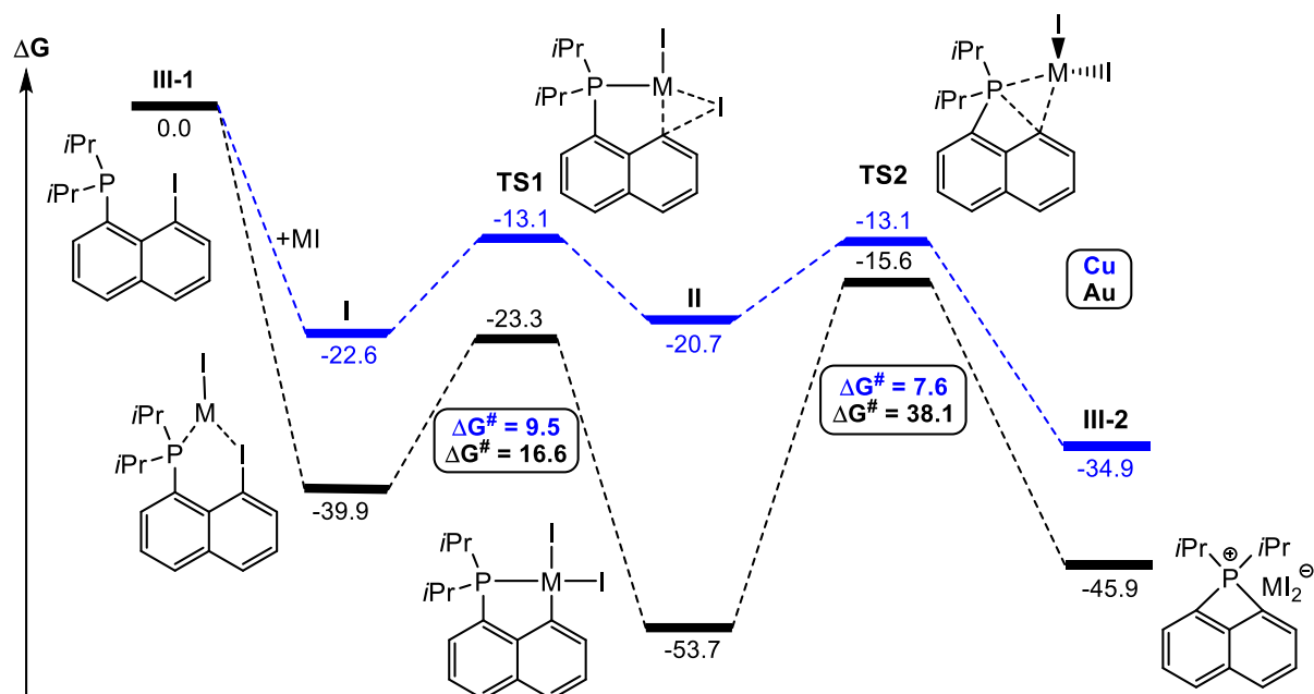
Schéma 11 : Profils énergétiques calculés au niveau de théorie SMD(dichlorométhane) B3PW91/SDD+f(M), SDD(I), 6-31G** (autres atomes) pour les réactions entre la 8-iodonaphtyl-1-phosphine III-1 avec CuI et AuI. (Energie libre en kcal/mol.).
