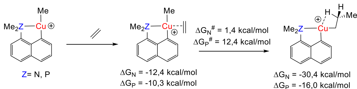
Schéma 12 : Calculs DFT au niveau de théorie (B97D/SDD+f(Cu),6-31G**(autres atomes)) pour l'insertion migratoire de l'éthylène dans la liaison Cu^{III} -Me avec les ligands (P,C) et (N,C) ( \Delta G en kcal/mol) – site de coordination en trans de l'hétéroatome.
