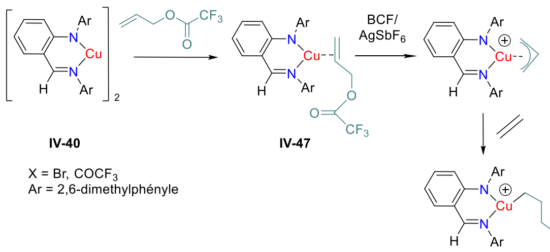
Schéma 32 : Stratégie envisagée pour obtenir un complexe \pi -allyle de cuivre(III) à partir du complexe IV-47 .
