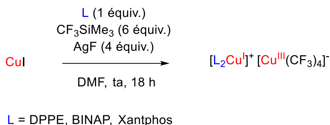
Schéma 38 : Synthèse des paires ioniques avec les ligands (P,P).
