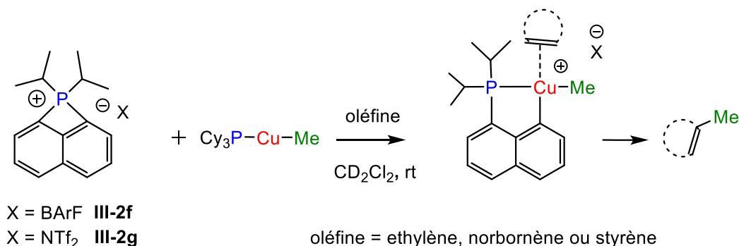
Schéma 31 : Réactivité des phosphoniums III-2f et III-2g avec le \text{Cy}_3\text{P}-\text{Cu}-\text{Me} .
