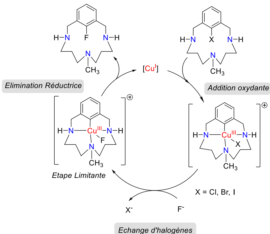
Schéma 21 : Cycle catalytique pour l'échange d'halogène.
