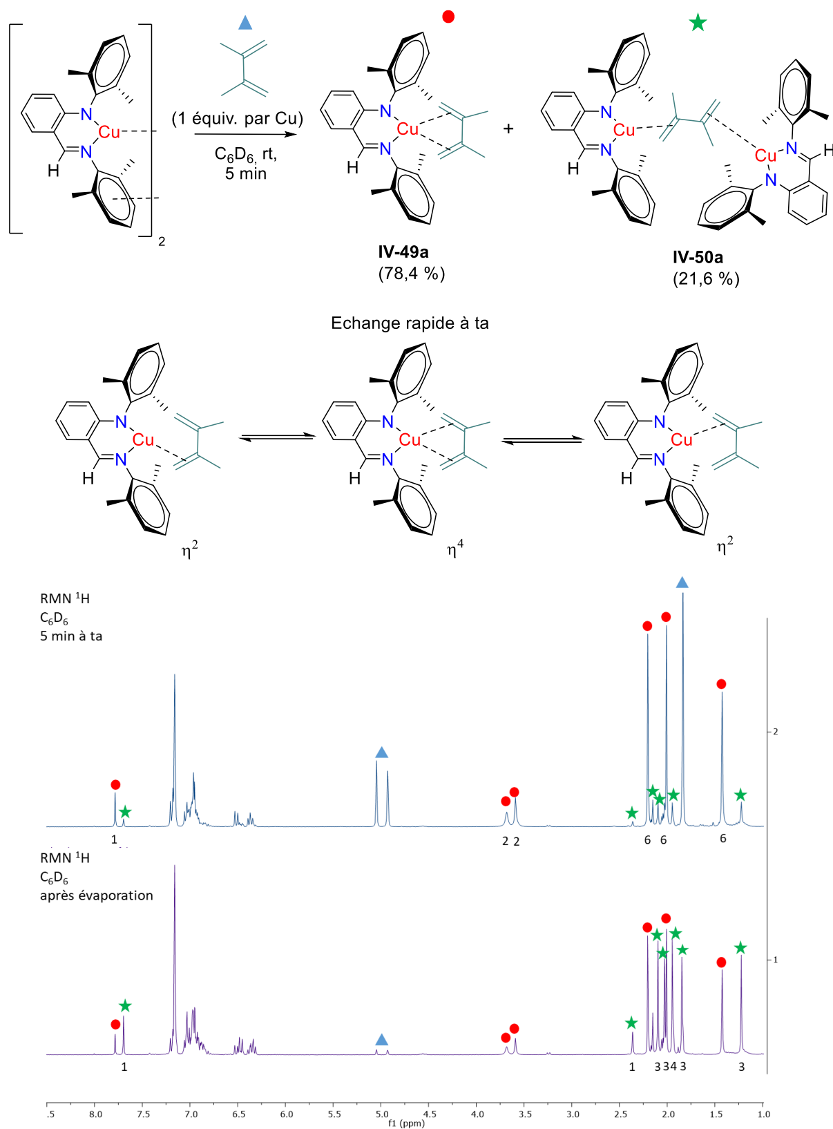
Schéma 34 : Réaction entre le complexe de cuivre(I) IV-40 et la 2,3-diméthylbutadiène dans le benzène- \text{d}_6 . Spectres RMN ^1\text{H} de la réaction montrant l'évolution des deux espèces.
