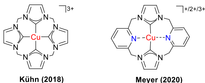
Schéma 26 : Exemples d'organocuivres(III) stabilisés par des NHC.
