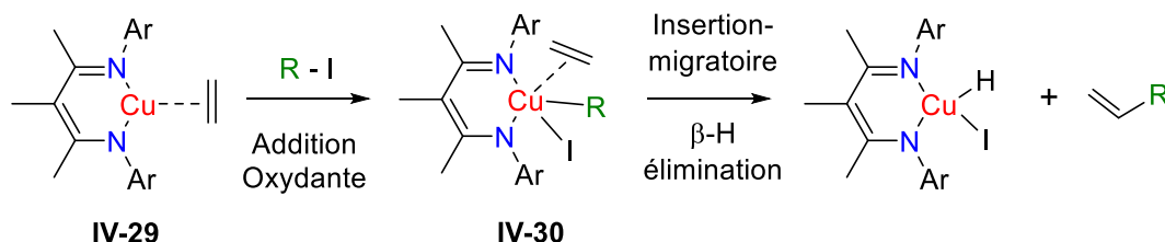
Schéma 16 : Réactivité d'addition oxydante envisagée avec les complexes \beta -dikétiminates de \text{Cu(I)} stabilisés par une oléfine.
