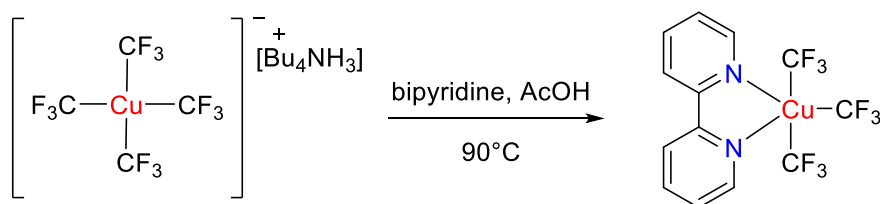
Schéma 32 : Synthèse du complexe [(\text{bpy})\text{Cu}^{\text{III}}(\text{CF}_3)_3] .
