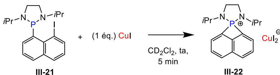
Schéma 14 : Réactivité de la phosphine III-21 avec CuI .
