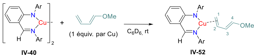
Schéma 37 : Formation du complexe de cuivre(I) IV-52 obtenu à partir du dimère de cuivre(I) IV-40 .
