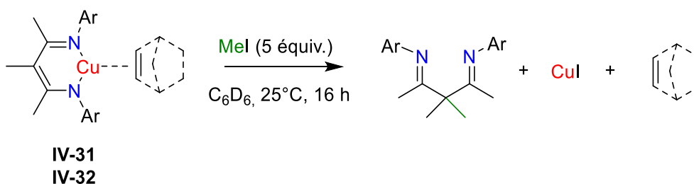
Schéma 18 : Réactivité des complexes IV-31 et IV-32 vis à vis de MeI.
