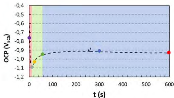
Figure 85 : Potentiel à circuit ouvert de l'alliage d'aluminium 2024-T3 A_{poli} dans la solution de conversion TCS et position sur la courbe des zones de potentiel étudiées
