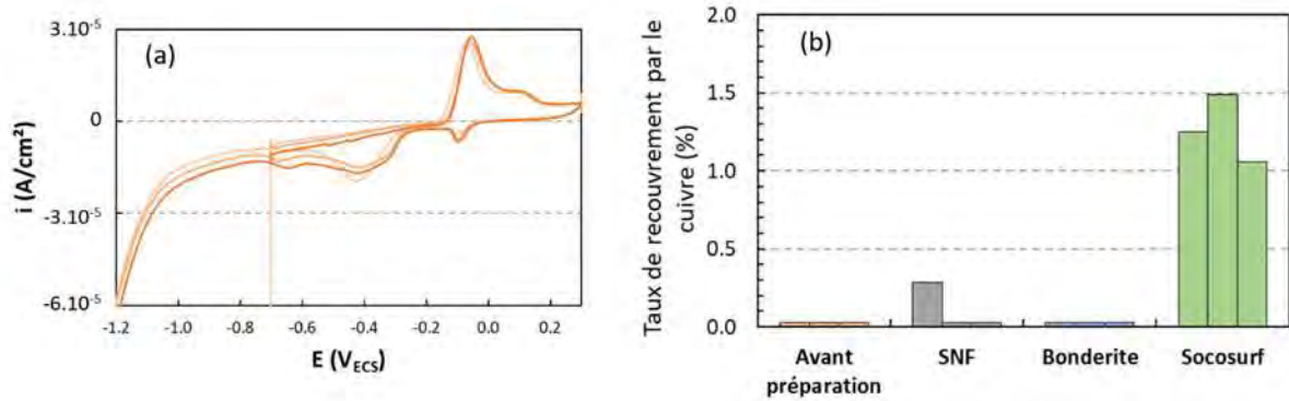
Figure 39 : (a) Polarisation cyclique du cuivre en milieu borate désaéré et (b) Taux de recouvrement par le cuivre en surface de l'alliage 2024-T3 A laminé avant préparation et après exposition à différents bains de décapage acide
