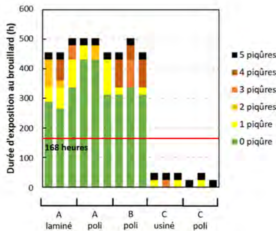
Figure 46 : Résultats de l'exposition au brouillard salin neutre des différents lots d'alliage 2024-T3 et T351 étudiés
