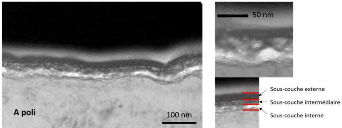
Figure 49 : Micrographie MET en champ clair de la couche de TCS formée sur substrat A_{poli} (lame FIB)
