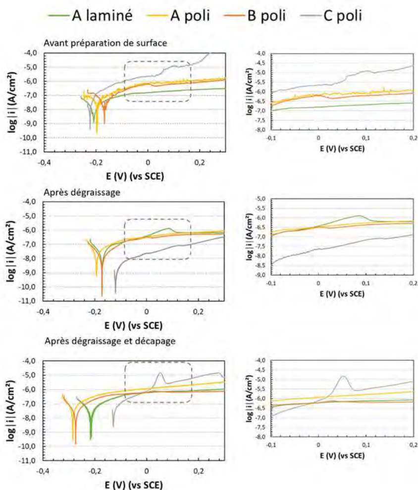
Figure 43 : Courbes de polarisation anodique tracées en milieu \text{Na}_2\text{SO}_4 0,1M après chaque étape de la préparation de surface pour les alliages d'aluminium 2024 étudiés
