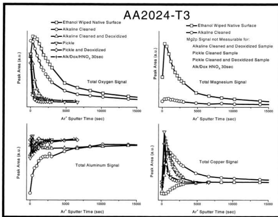
Figure 12 : Profils de concentration en fonction du temps de pulvérisation de l'alliage 2024-T3 réalisés à partir des pics XPS \text{O}1s , \text{Mg}2p , \text{Al}2p et \text{Cu}2p pour différents traitements de surface [49]
