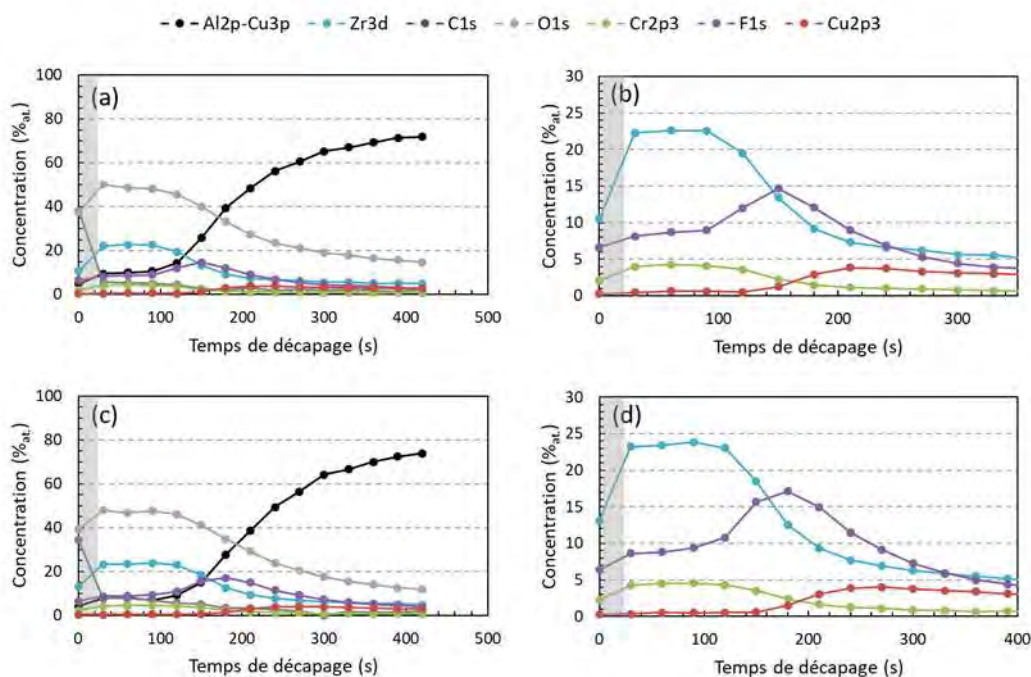
Figure 104 : Profils de concentration XPS des couches de conversion formées sur le substrat A_{poli} après (a, b) 300 et (c, d) 600 secondes d'immersion dans la solution de conversion TCS. La zone grisée correspond à la zone polluée par le carbone atmosphérique
