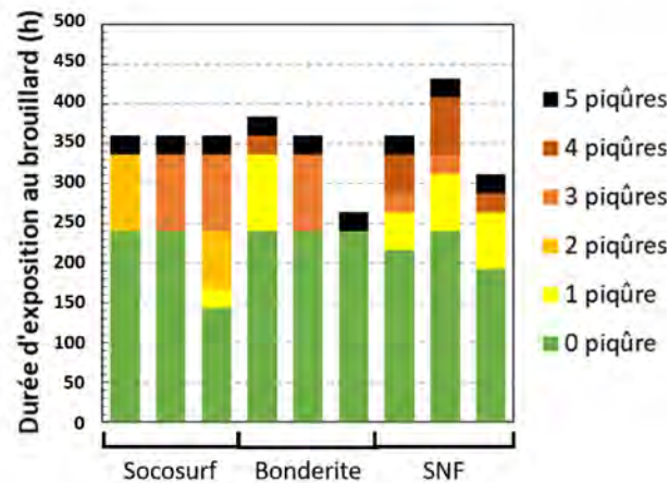
Figure 40 : Résultat de l'exposition au brouillard salin neutre du substrat 2024T3 A_{\text{laminé}} après traitement de surface TCS-PACS pour trois solutions de décapage différentes (Socosurf, Bonderite, SNF) utilisées durant la préparation de surface
