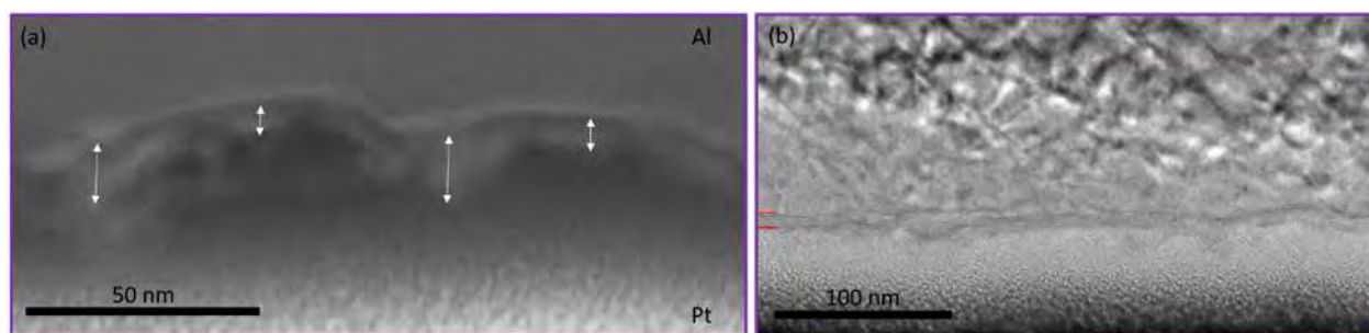
Figure 90 : Micrographie (a) STEM et (b) MET en champ sombre de la couche de conversion formée sur le substrat A_{poli} après 3 secondes d'immersion (les flèches blanches sur la micrographie (a) ainsi que les marques rouges sur la micrographie (b) indiquent la couche de conversion)
