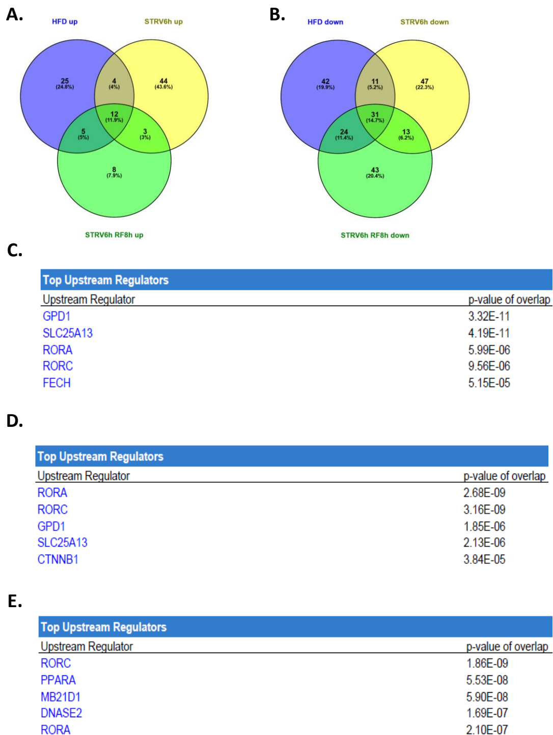
Figure 40 : RORα et RORγ pourraient en partie expliquer les effets géniques observés lors de la délétion hépatique d'HMGB1.
