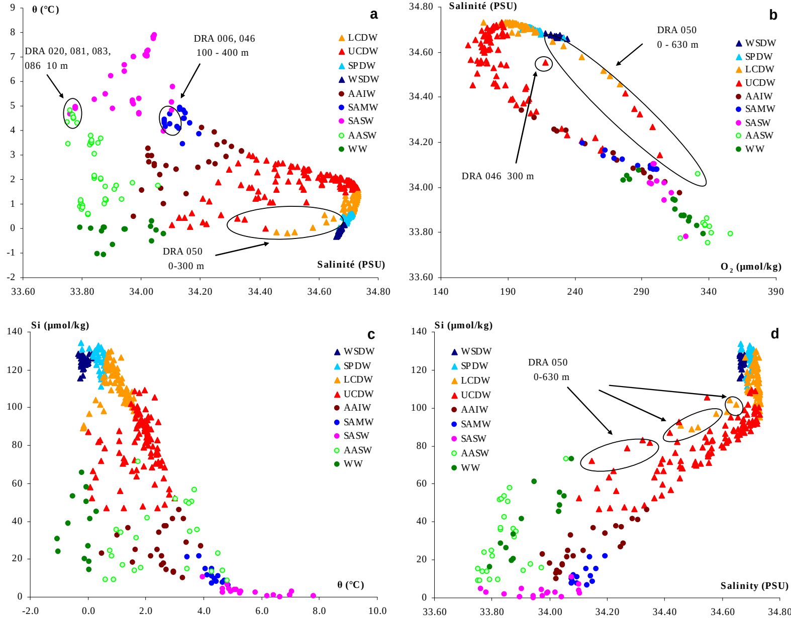
Figure VI.9 : Diagrammes \theta -S (a), S- O_2 (b), Si(OH)_4 - \theta (c) et Si(OH)_4 -S (d) pour les 22 stations CTD avec détermination du silicate par voltammétrie
