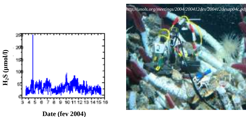
Figure III.16 : Déploiement du capteur potentiométrique H_2S sur le site EPR 9°50' N, Cruise AT-11-7 (Seyfried, 2004).
