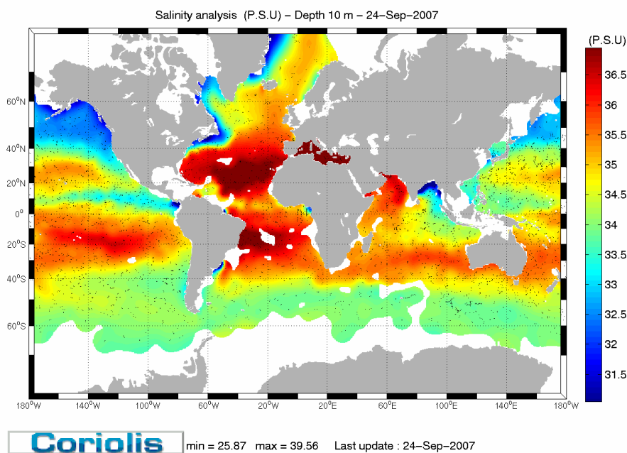
Figure III.5 : Exemple de données de salinité obtenues à 10 m de profondeur le 24 septembre 2007 http://www.coriolis.eu.org/
