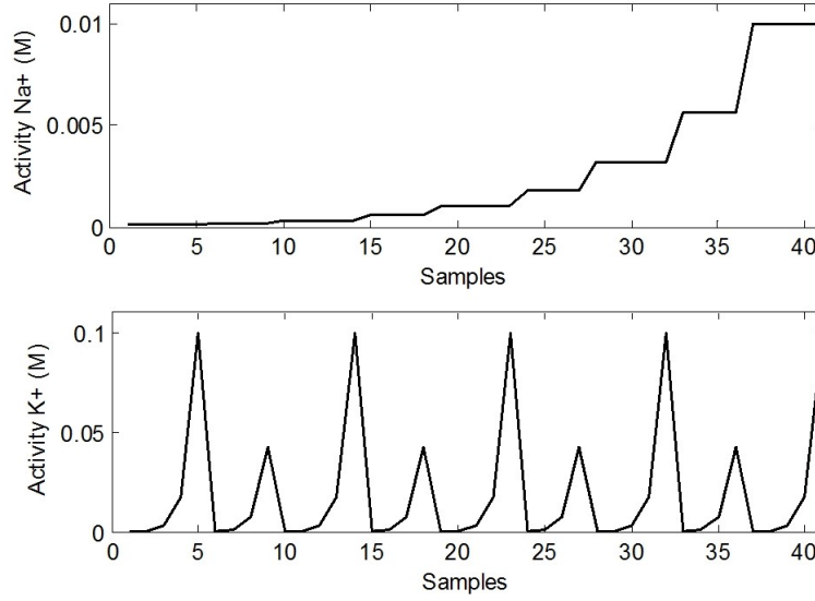
Figure 5.2: Activités des ions \text{Na}^+ et \text{K}^+ .
