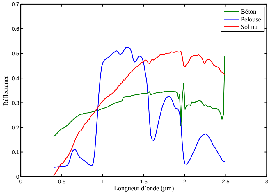
Figure 4.1: Spectres utilisés dans le Test 2
