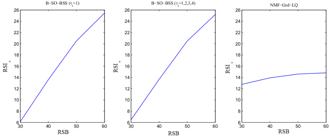
Figure 5.4: RSI_s en fonction du RSB dans le cas de l'Expérience 3.
