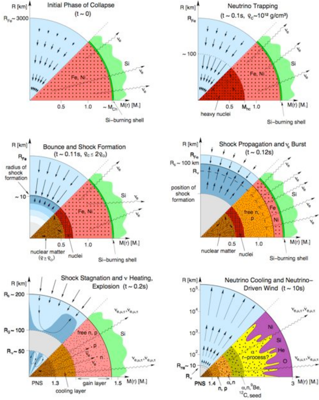
FIG. 1.1 – Synoptique des premières phases d’une supernova de type core-collapse : effondrement gravitationnel du progéniteur, rebond du cœur et formation d’un choc, essoufflement puis résurrection (à démontrer) du choc par la luminosité neutrinique de la PNS en contraction [d’après Janka et al., 2007].
