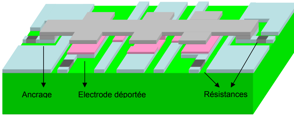
Figure II. 13: Schématisation d'un commutateur capacitif série avec électrodes déportées et résistances intégrées
