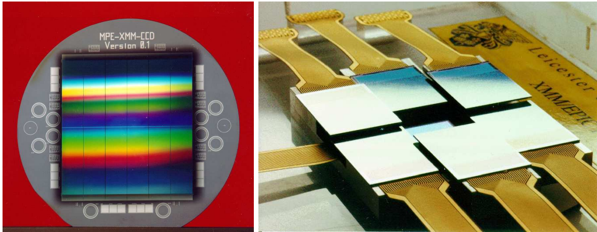
FIG. 3.2 – Photos des détecteurs PN (gauche) et MOS (droite) composant l'instrument EPIC.
