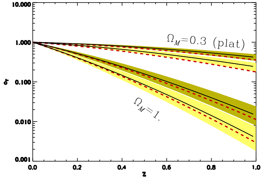
FIG. 5.15 – Effet du choix de la fonction de masse sur les comptages relatifs. Je représente ici l'évolution de l'abondance des amas, relativement à l'abondance locale, pour différents modèles cosmologiques (grande densité de matière en bas et faible densité en haut) et pour des amas de température 4 keV (zone foncé) et 6 keV (zone claire). Les courbes en tirets et en pointillées représentent respectivement les cas avec la fonction de masse de Press & Schechter pour les deux types d'amas (les zones pleines sont calculées avec la fonction de Sheth & Tormen).
