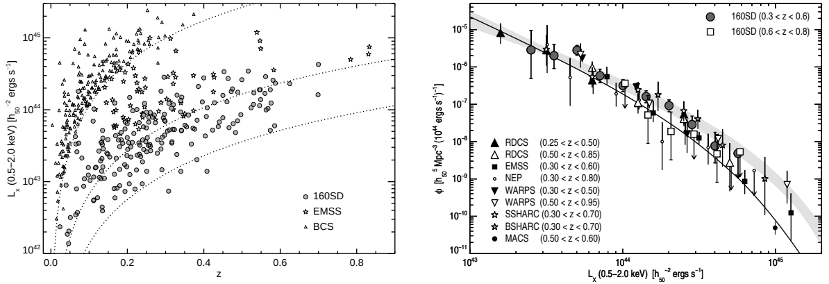
FIG. 4.8 – A gauche : distribution en luminosité X et en redshift des amas du 160deg 2 , EMSS et BCS. Les courbes pointillées représentent les flux limites 2.7 \times 10^{-12} , 1.5 \times 10^{-13} et 3 \times 10^{-14} erg.s -1 .cm -2 dans la bande [0.5–2.0 keV]. A droite : fonction de luminosité calculée à partir des différents échantillons disponibles [146].
