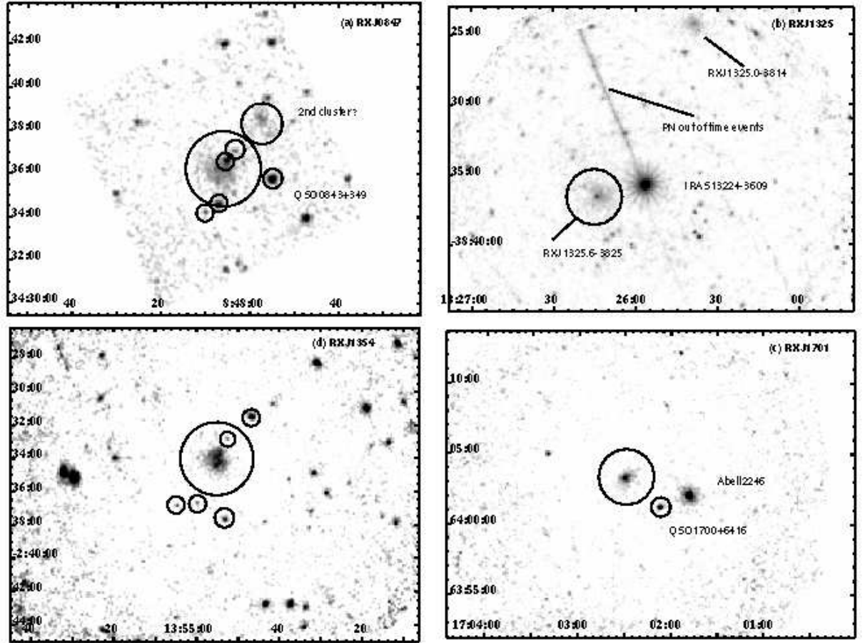
FIG. 3.6 – Images d’une région de environ \sim 15 \times 15 autour de RXJ0847.2(a), RXJ1325.5 (b), RXJ1701.3 (c) and RXJ1354.2 (d) - lissées par une gaussienne de largeur 4'' . Le large cercle représente la région d’extraction du spectre et les petits cercles les zones d’extraction de sources ponctuelles. Un nouveau candidat amas, XMMU J084701.8+345117 a été découvert (en haut a droite de RXJ0847.2). Les amas RXJ1325.5 et RXJ1325.0 sont très proches de la source IRAS 13224-3809. Dans le champ de l’amas RXJ1701.3, l’amas proche Abell 2246 et les QSO sont indiqués.
