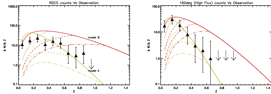
FIG. 5.19 – Comptages avec des seuils en température plus élevés que celui déduit du seuil de flux d’observation. Pour RDCS (à gauche) et 160deg 2 (à droite) avec les seuils : T=2, 3 et 4 keV et T=2, 3, 4 et 5 keV respectivement. Ces seuils ne sont ici appliqués qu’aux modèles puisque nous ne disposons pas des informations relatives aux amas individuels de l’échantillon RDCS. Par contre l’application de ces seuils au catalogue observé est possible avec le 160deg 2 , cf. figure 5.20.
