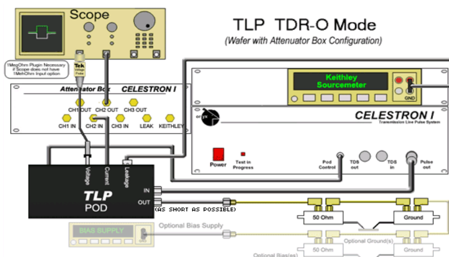
Figure 38: Connection de l'outils de test TLP avec Celestron.
