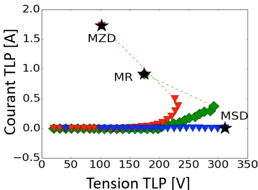
Figure 68: Itlp-Vtvp des trois planar-MESFET sur l'électrode de drain avec une tension de -15V appliquée sur la grille. Trois comportements distincts sont observés.
