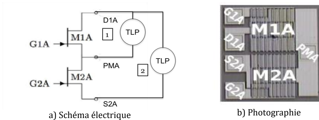
Figure 111: Schéma électrique et photographie de la fonction totem-pole, constitué de 2*12 cellules MESFET en parallèle.
