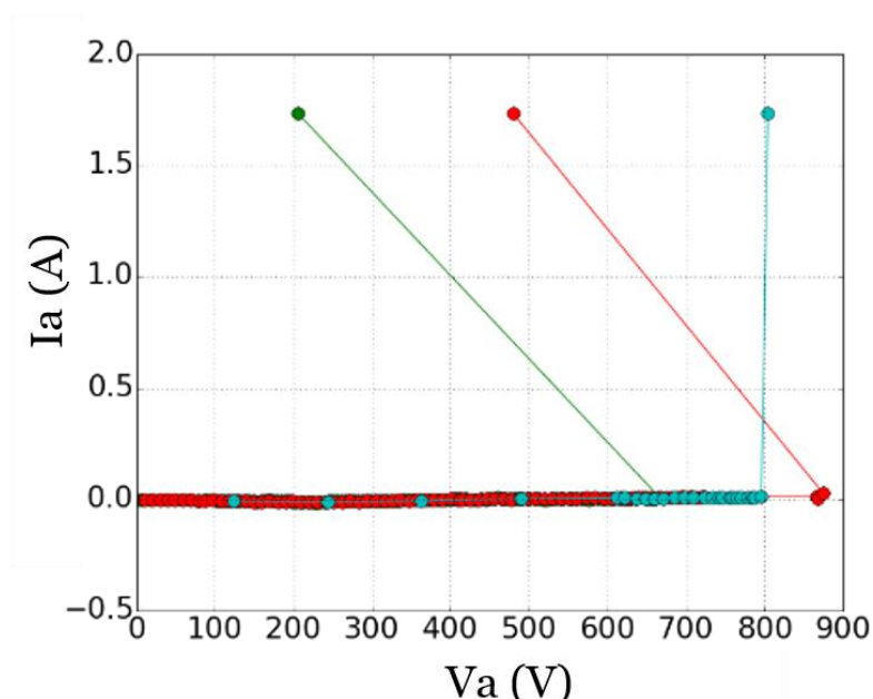
Figure 100: Itlp-Vtlp lors de stress TLP sur trois diodes Schottky en SiC polarisées en inverse. Aucun courant n'est supporté avant la défaillance subite.
