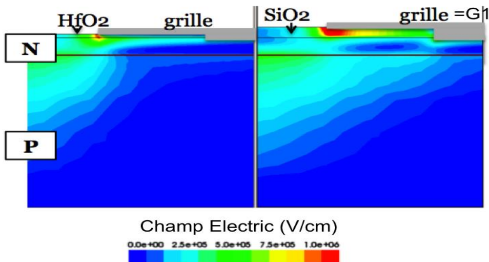
Figure 99: Comparaison entre le HfO 2 et le SiO 2 sur la répartition du champ électrique dans le MESFET SiC à V_{t1p}=200V .
