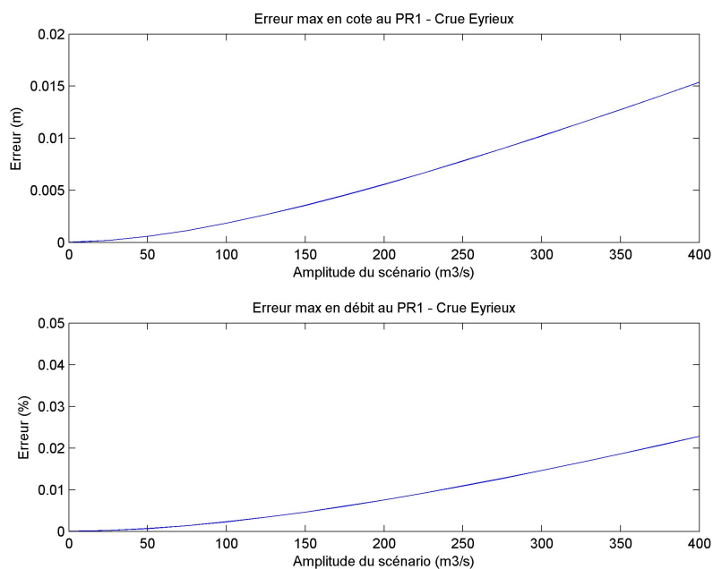
FIGURE B.10 – Évolution de la différence en débit et en cote entre le modèle linéaire et le modèle non-linéaire au PR1 pour différents échelons de débit à l’Eyrieux
