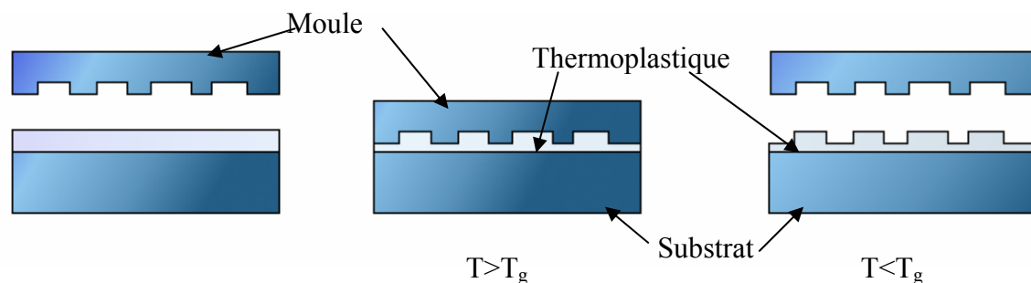
Figure 3.10 Principe de nanoimpression d'un thermoplastique
