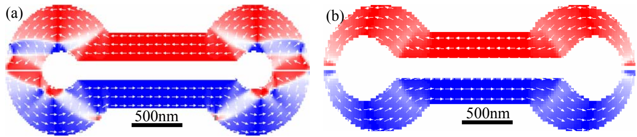
Figure 2.23 Simulation des électrodes. Dans l'optique de supprimer les vortex aux abords des séparations (a), la structure a été affînée, augmentant le couplage magnétique entre les deux électrodes (b)
