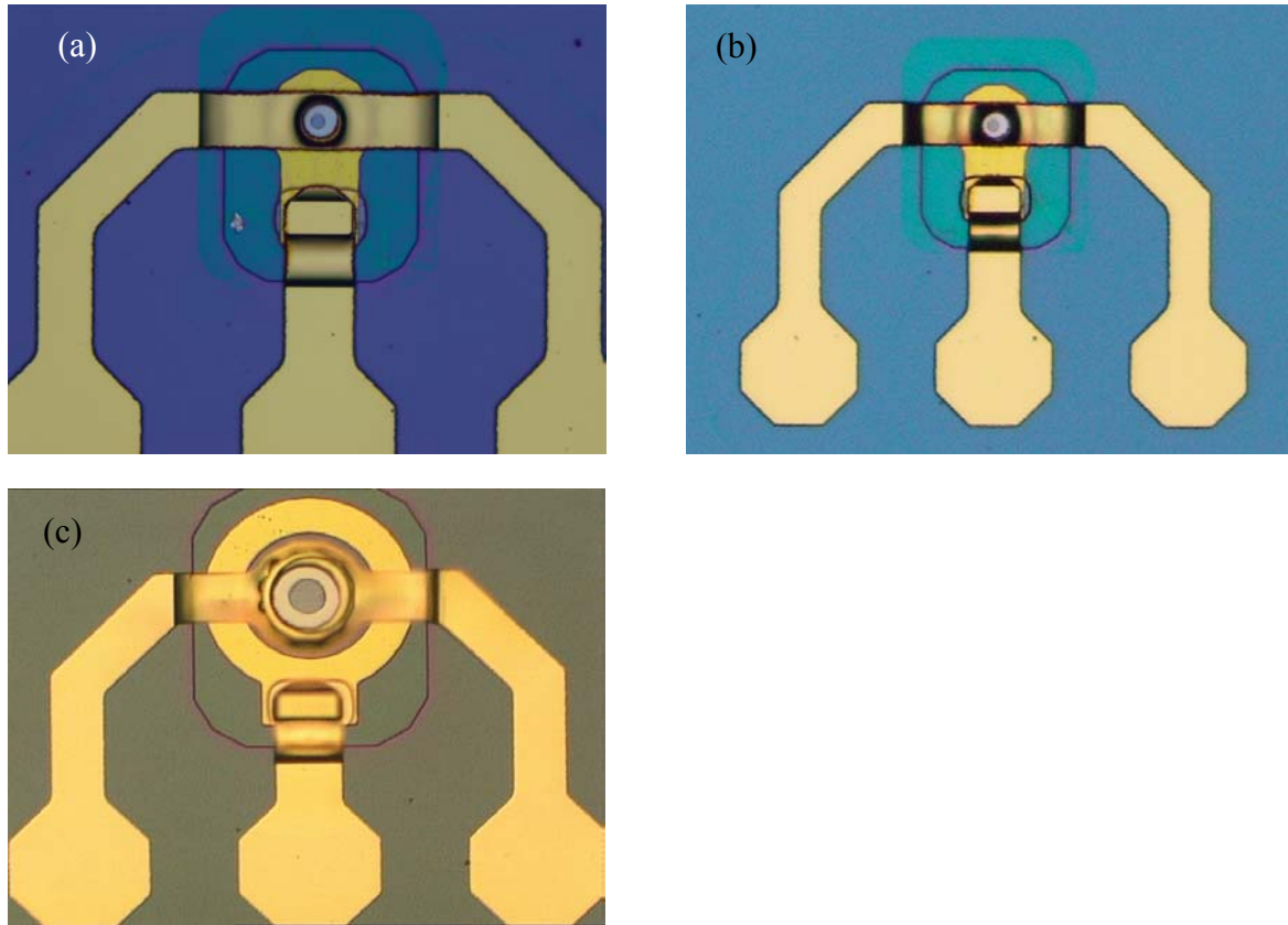
Figure 2.18 SpinLED à mesa de zone active de 20μm (a), 40μm (b), et 60μm (c) de diamètre
