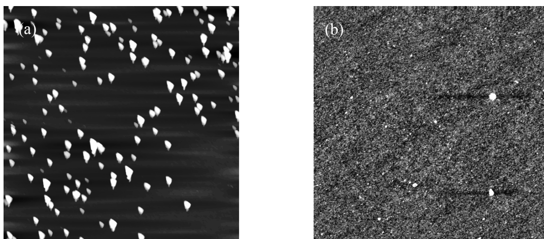
Figure 3.24 Observation AFM d'une surface de GaAs traitée avec (a) de l'APTS et (b) de l'APDEMS. La taille des agrégats est de 100nm dans le cas de l'APTS et de 3nm dans le cas de l'APDEMS
