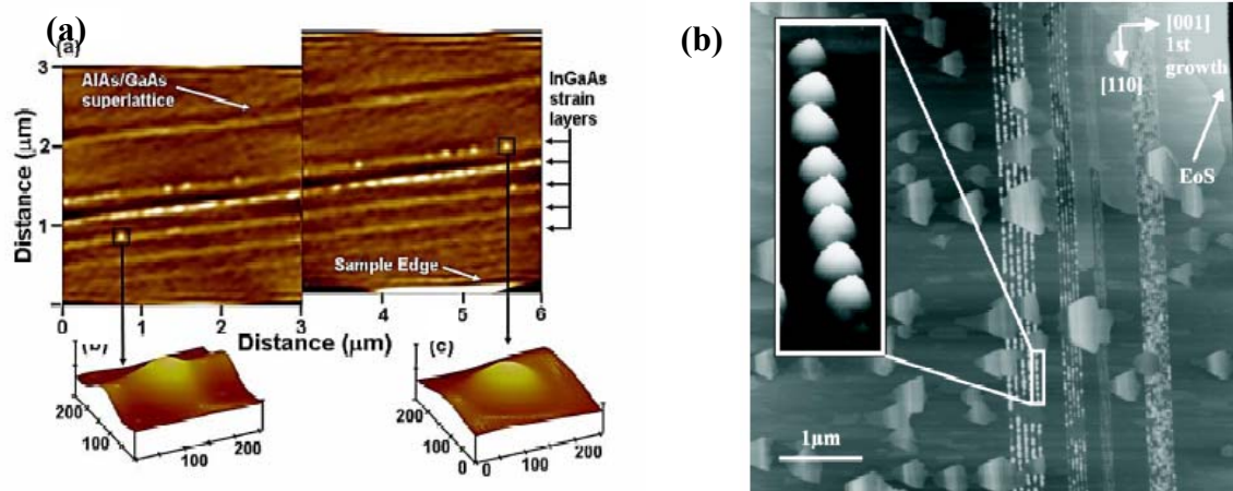
Figure 1.3 Image de MET et AFM montrant l'alignement des boîtes quantiques le long de puits quantiques clivés (a) GaInAs/GaAs et (b) AlAs/GaAs [Ballet01]
