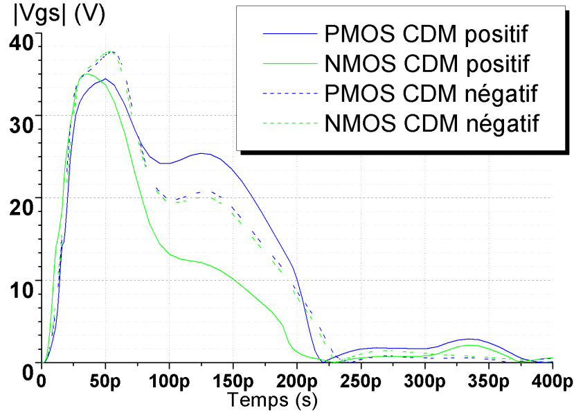
FIG. 2.25 – Surtension simulée au niveau des grilles du PMOS et du NMOS de l'étage stressé
