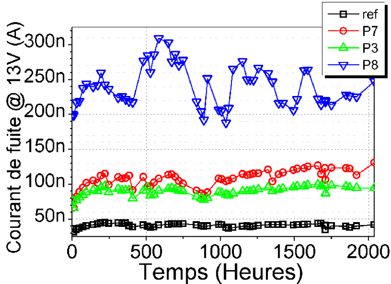
FIG. 3.14 – Courant de fuite avant et après le vieillissement de 2000 heures à 125^\circ\text{C}
