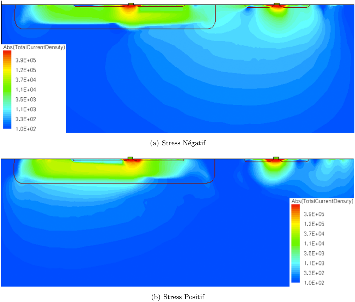
FIG. 2.24 – Résultats de simulation montrant la densité de courant dans la structure au niveau du pic en courant du stress SCDM
