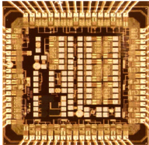
FIG. 2.5 – Véhicule de test monté dans un boîtier PGA 68
