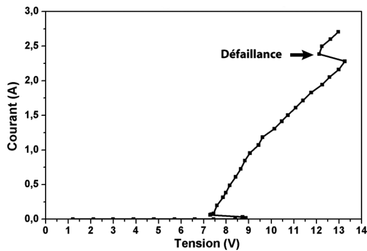
FIG. 3.9 – Caractéristique quasi-statique du GCNMOS
