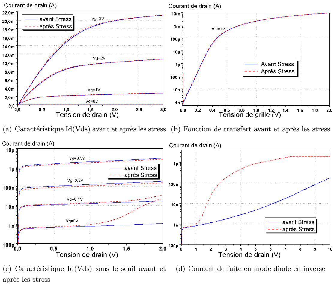
FIG. 3.24 – Évolution des caractéristiques statiques avant et après stress
