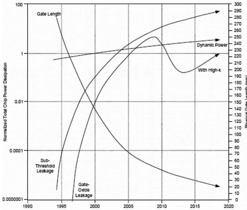
FIG. 1.14 – Evolution future des courants de fuite dans les circuits microélectroniques
