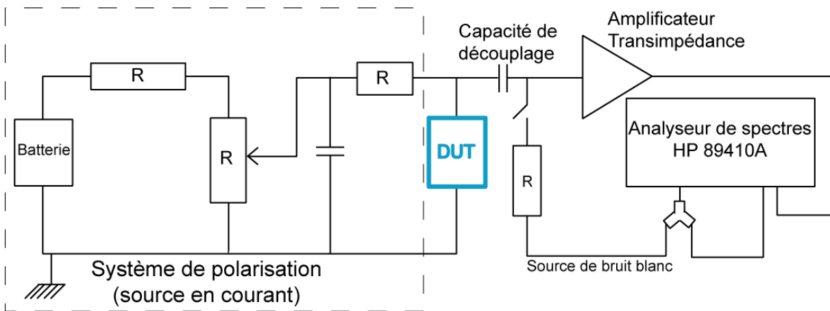
FIG. 3.6 – Banc de mesure du bruit basse fréquence
