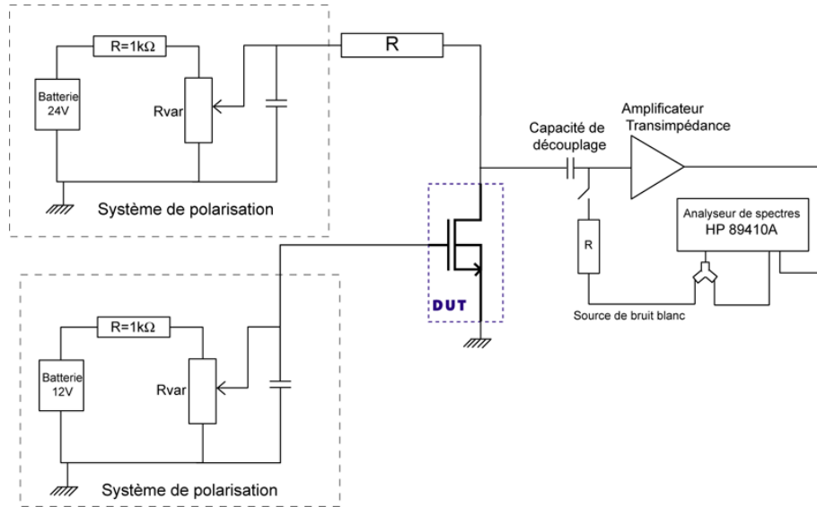
FIG. 3.25 – Schéma du banc de mesure du bruit basse fréquence
