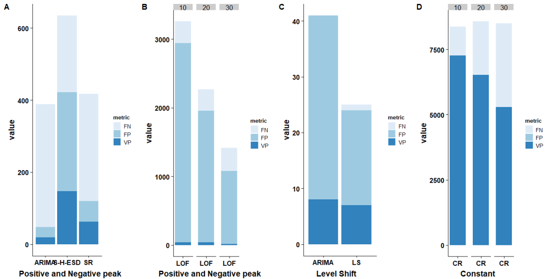
Figure III.2.2 – Évaluation des méthodes de détection d'anomalies sur les données d'index de calorie.
