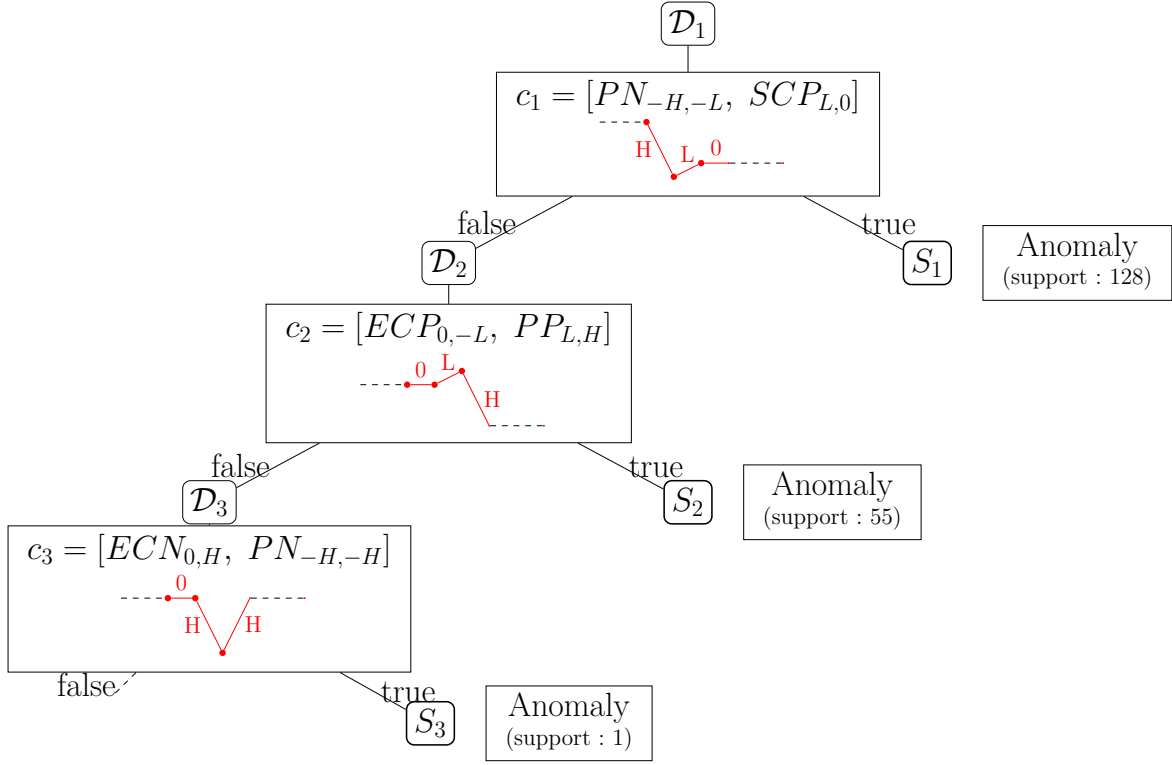
Figure II.3.5 – Illustration d'un arbre obtenu avec CDT.
