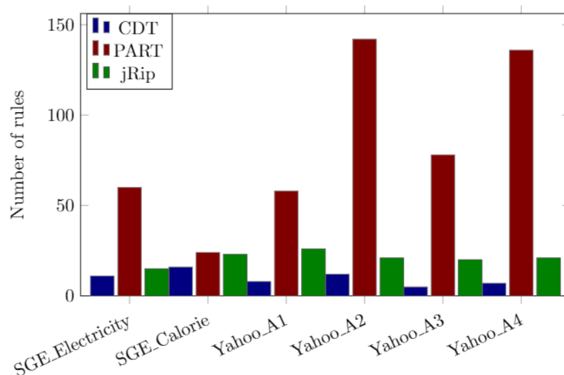
Figure III.3.2 – Le nombre de règles générées pour les algorithmes CDT, PART et JRip pour la détection d'anomalies.
