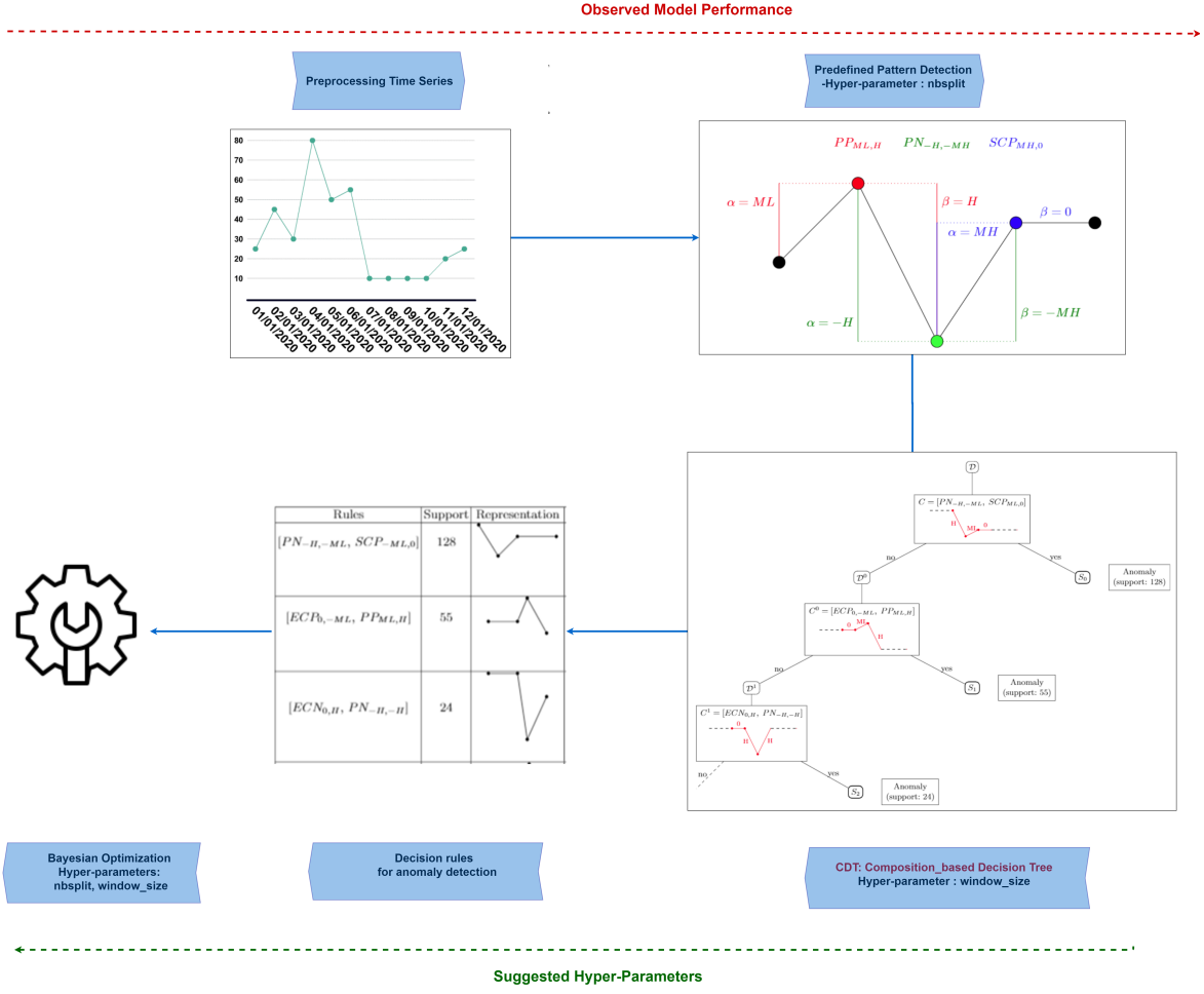
Figure II.3.1 – Les différentes étapes de l’approche CDT.
