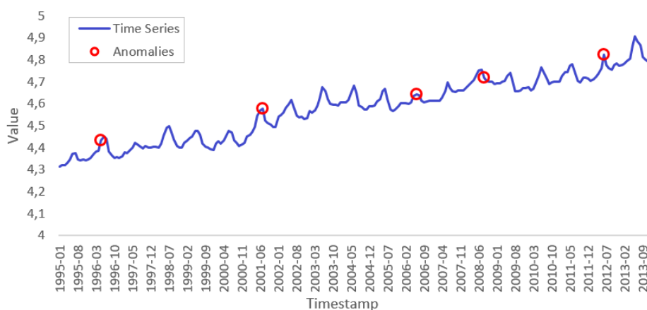
Figure III.1.1 – Exemple de DataSets HIPC avec des anomalies de types AO et TC.
