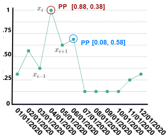
Figure II.3.2 – Exemple de variation de type Pic Positif (PP). Il y a deux modèles marqués PP_{[0.88,0.38]} et PP_{[0.08,0.58]} correspondant à multiple pics positifs mais avec des amplitudes différentes.
