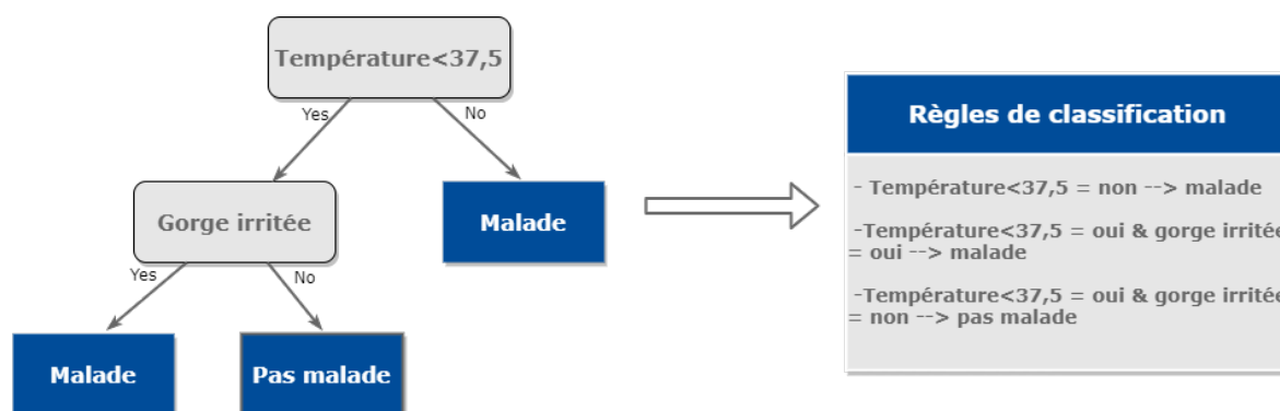
Figure I.2.6 – Technique de classification basée sur des règles d'arbre de décision.
