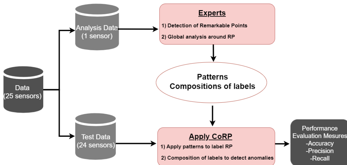
Figure III.2.1 – Processus d’évaluation de l’algorithme CoRP sur les données de SGE.
