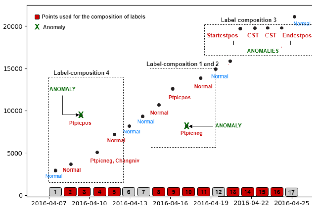
Figure II.2.4 – Résultat de la phase 2 de l'algorithme CoRP.
