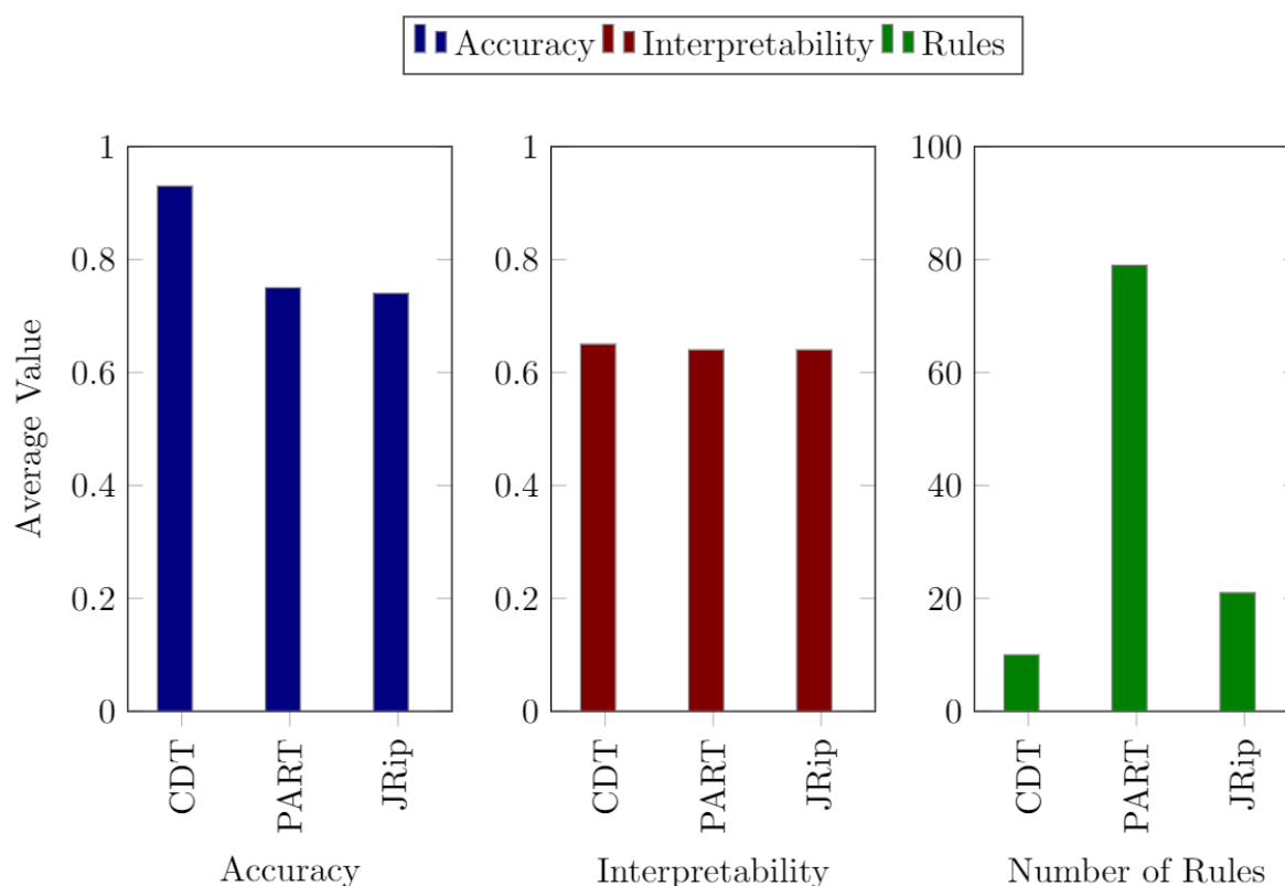
Figure III.3.3 – Le compromis entre la précision, l'interprétabilité et le nombre de règles pour les algorithmes CDT, PART et JRip.
