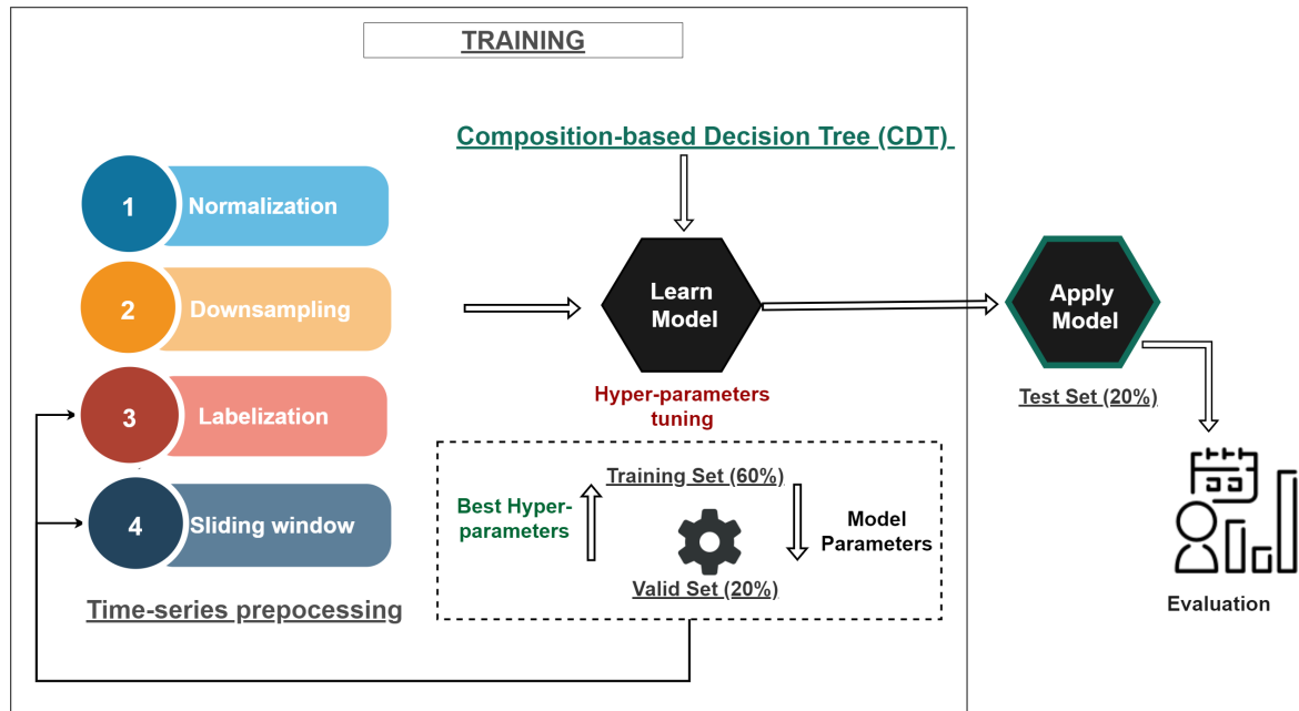
Figure III.3.1 – Processus d'évaluation de CDT
