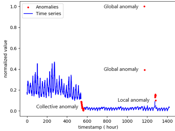
Figure III.1.2 – Exemple de DataSets Yahoo : des séries temporelles du trafic Web.
