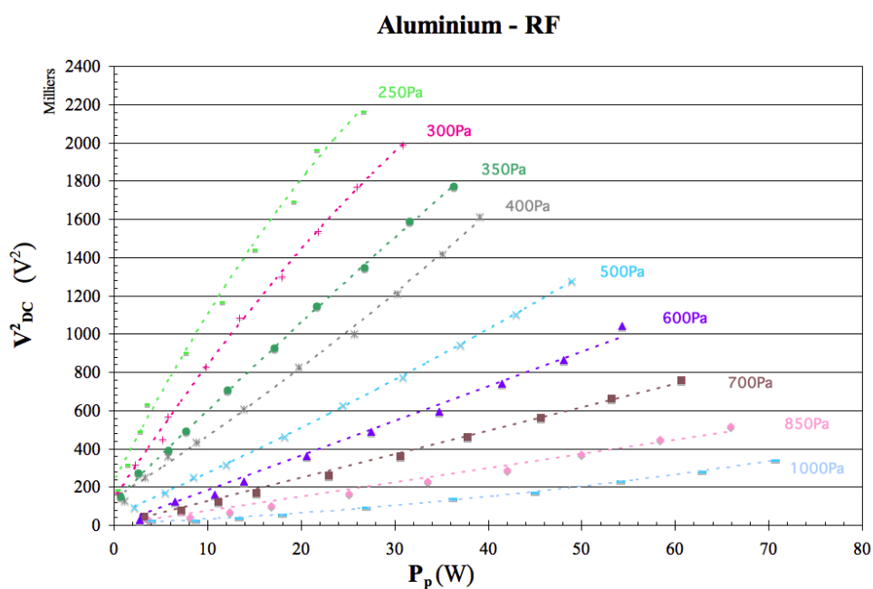
Graphique.II. 9. Variation du carré de la V_{DC} en fonction de la puissance pour l'aluminium en mode RF.
