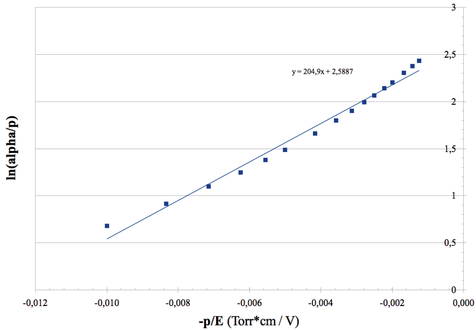
Graphique.III. 1. \ln(\alpha/p) en fonction de -p/E dans la gamme de 100-1000 \text{ V} \cdot (\text{Torr} \cdot \text{cm})^{-1} . Les points correspondent aux mesures et le trait continu à une régression linéaire.
