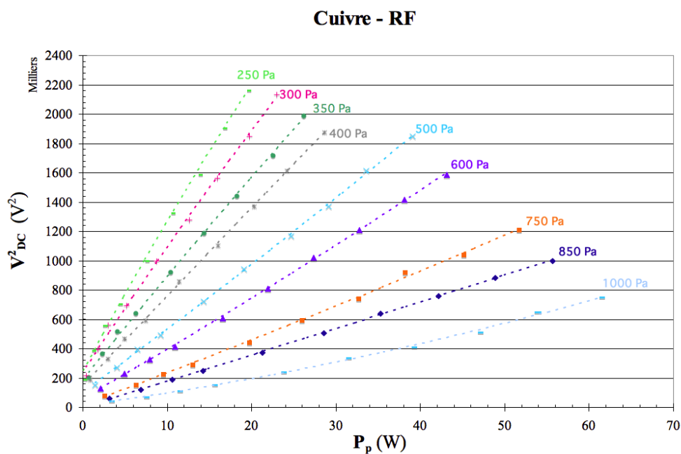
Graphique.II. 8. Variation du carré de la V_{DC} en fonction de la puissance pour le cuivre en mode RF.
