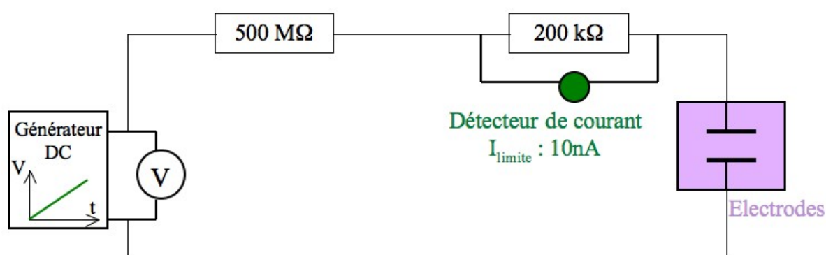
Figure.III. 5. Schéma du circuit électrique.
