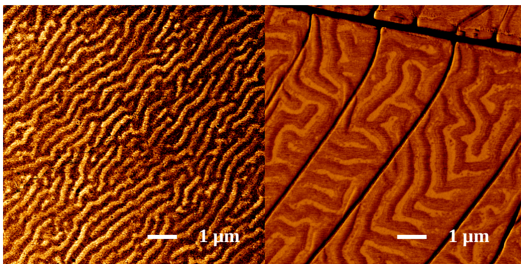
Figure 2 : Image AFM 10 \mu\text{m} x 10 \mu\text{m} d'une surface de PDMS ayant subi un traitement plasma \text{O}_2 , l'échelle en z est de 5 nm. A gauche le PDMS à été exposé à un plasma oxygène 200 W pendant 1 min. A droite le PDMS à été exposé à un plasma oxygène 200 W pendant 5 min.
