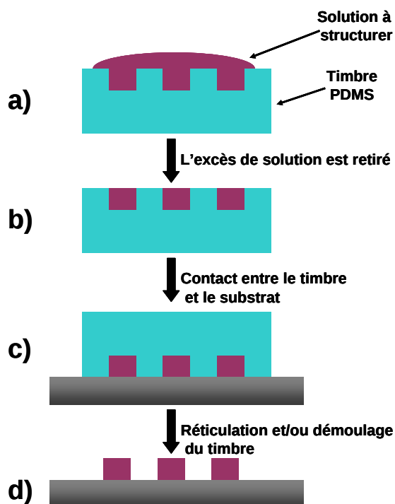
Figure 1 : Principe général du Microtransfer Molding ( \mu TM). a) La solution à structurer est déposée sur le timbre, b) L'excès de solution est retiré du timbre soit par un flux d'azote qui chasse la goutte du timbre soit en « raclant » la surface du timbre à l'aide d'un timbre de PDMS plat. c) Le timbre est ensuite amené en contact avec le substrat, la solution est réticulée si besoin et le timbre est retiré laissant des structures épaisses sur le substrat.
