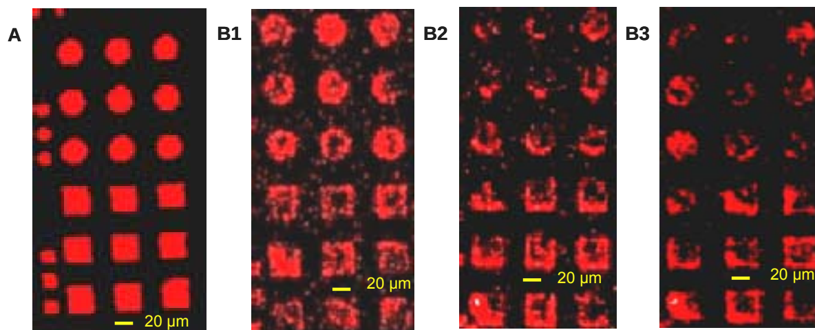
Figure 13 : (A) Image en fluorescence du premier dépôt, et (B) montre les dépôts numéros 5 (B1), 6 (B2) et 7(B3). Un timbre a été encre avec une solution d'oligonucléotide 10 \mu Mol de 15-mer 5'-Cy5 pendant 30 sec puis a été placé en contact pendant 2 minutes avec une dendrilame et ce 10 fois consécutivement en des positions différentes de la lame.
