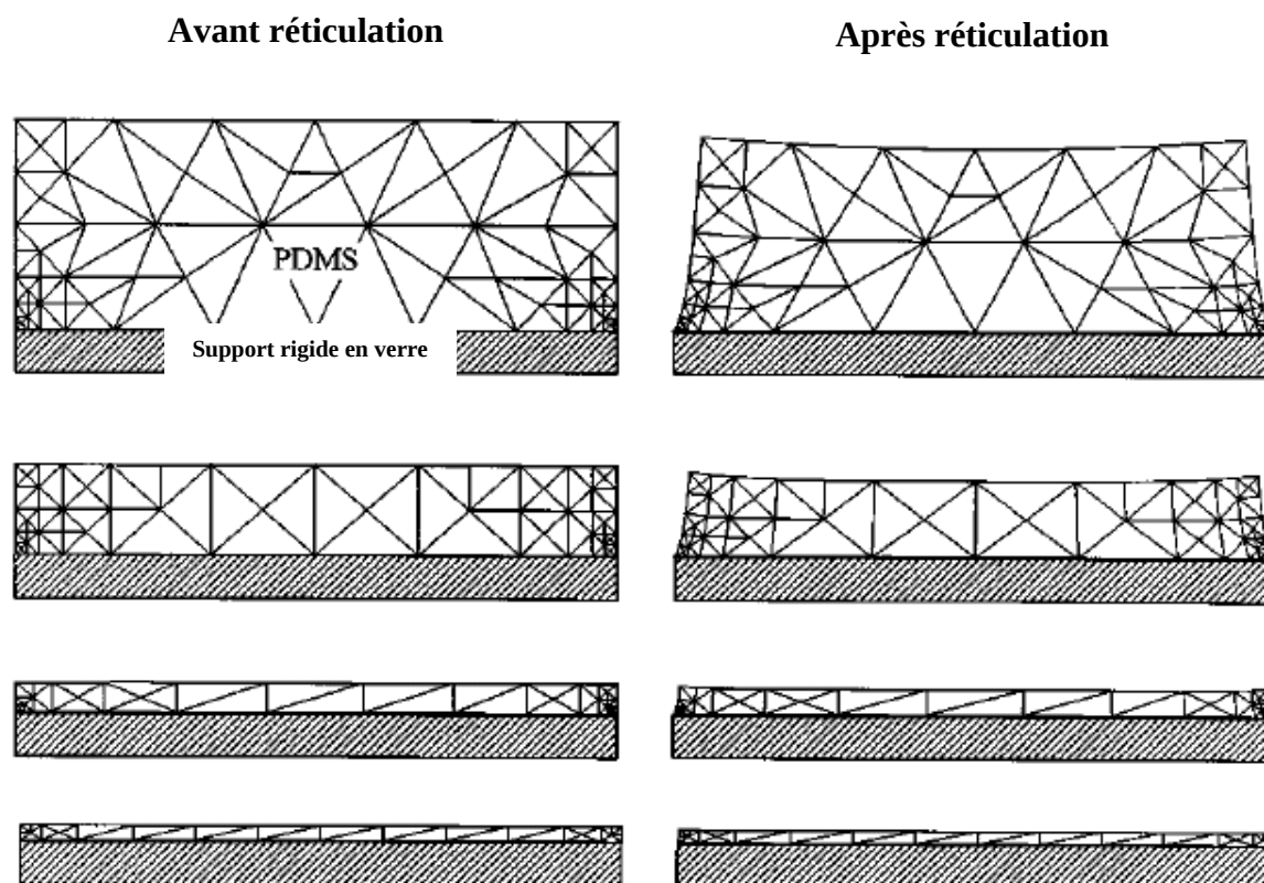
Figure 18 : Simulation du retrait thermochimique en fonction de l'épaisseur du timbre, avant et après réticulation. La partie gauche représente un timbre en PDMS avant réticulation déposé sur un support rigide en verre. Nous pouvons noter qu'aucune déformation n'est présente quelle que soit l'épaisseur du timbre. La partie droite représente le même timbre après réticulation. Nous pouvons constater que la déformation diminue avec la diminution en épaisseur du timbre.
