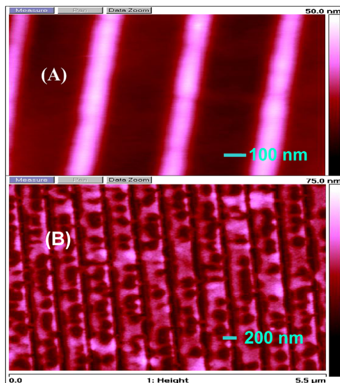
Figure 2 : Résolution ultime de \mu TM avec une solution de dendrimères. (A) Image AFM des motifs du timbre, la largeur des lignes est de 40 nm. (B) Image AFM du résultat du \mu TM de motifs de dendrimères sur du silicium, les lignes font 36 nm de large pour un pas de 400 nm.
