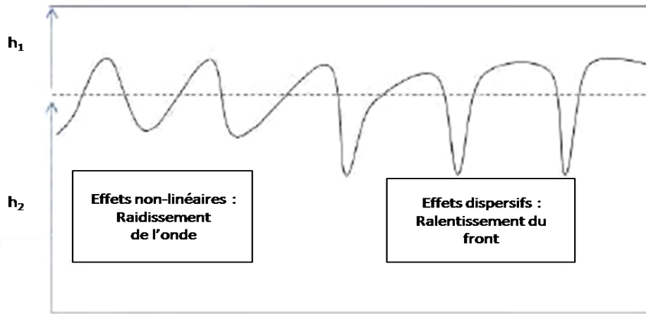
Figure 2.11 : Mécanisme de formation d'une onde solitaire. (Tiré de Dossmann, 2012)
