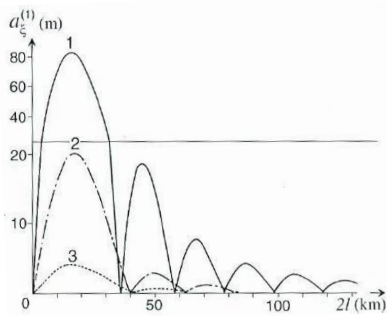
Figure 2.17: Amplitudes associées au déplacement vertical ( a_{\xi,n} = \frac{a_n k_{x,n}}{\omega} ) du premier mode barocline ( j = 1 ), généré par un flux de marée de \psi_0 = 200 \text{ m}^2/\text{s} pour différentes valeurs de hauteurs du mont océanique h_0 = (3.5, 2.5, 1) km (courbe 1, 2, 3) dans un océan de profondeur H = 4 km en fonction de la largeur, 2l du mont. Les paramètres de la pycnocline sont N\rho = 0.005 \text{ s}^{-1} , H\rho = 100 \text{ m} , \Delta H\rho = 50 \text{ m} . (Tiré de Vlasenko et al., 2005)
