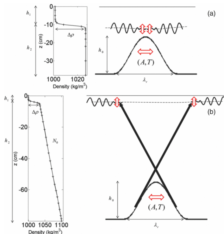
Figure 2.12 : Mécanisme de génération d'ondes solitaires. (a) génération primaire associée à un profil de stratification vertical « bicouche »; (b) génération secondaire associée à un profil de stratification vertical « tri-couche ». (Tiré de Dossmann et al., 2014)
