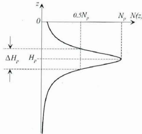
Figure 2.15: Profil de stratification N(z) utilisé par Vlasenko, Stashchuk et Hutter (2005). H_p désigne la profondeur de la pycnocline, N_p la valeur maximal de la stratification à cette profondeur et \Delta H_p la largeur de la pycnocline (Tiré de Vlasenko et al., 2005)
