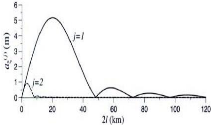
Figure 2.16 : Amplitudes associées au déplacement vertical ( a_{\xi,n} = \frac{a_n k_{x,n}}{\omega} ) des deux premiers modes baroclines ( j = 1, 2 ), générées par un flux de marée de \psi_0 = 20 \text{ m}^2/\text{s} au dessus d'un mont océanique de hauteur h_0 = 2 \text{ km} dans un océan de profondeur H = 4 \text{ km} en fonction de la largeur, 2l du mont. Les paramètres de la pycnocline sont N_p = 0.02 \text{ s}^{-1} , H_p = 100 \text{ m} , \Delta H_p = 50 \text{ m} . (Tiré de Vlasenko et al., 2005)
