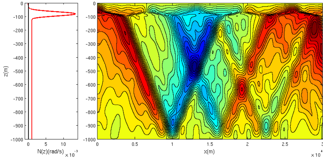
Figure 2.13 : (gauche) ligne rouge : profil de stratification N(z) pour les paramètres : f = 0 , H = 1000\text{m} , N_b = 1.10^{-3} \text{ s}^{-1} , N_p = 1.3.10^{-2} \text{ s}^{-1} ( H_p = 80 \text{ m} , \Delta H_p = 30\text{m} , \Delta \rho = 0.5 ) / ligne noire : \omega = 1.4.10^{-4} \text{ s}^{-1} . (droite) Reconstruction du champ de vitesse verticale w à partir de la superposition de 10 modes propres pour a_n \sim 1/n .
