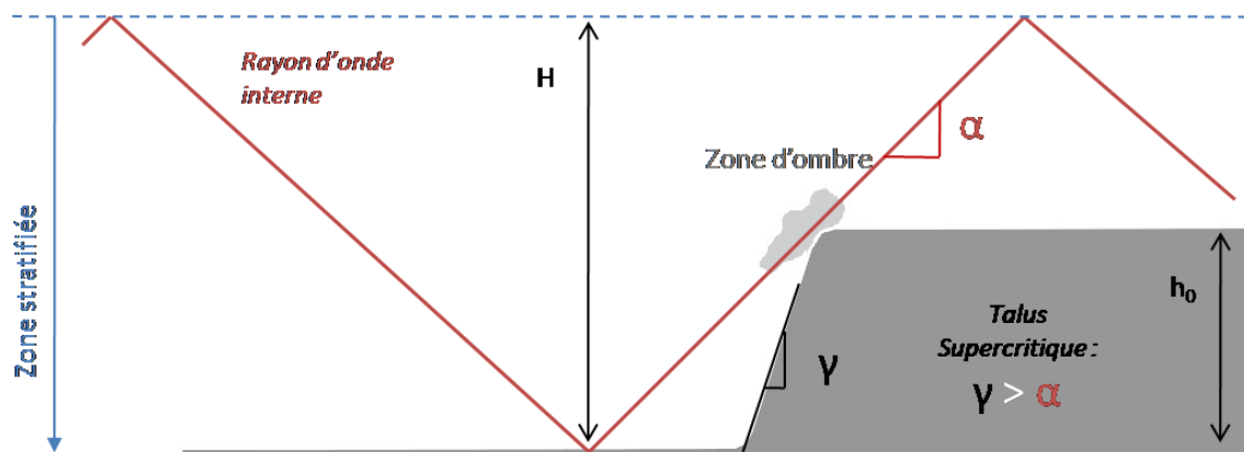
Figure 2.18 : Représentation schématisée de la génération d'un rayon d'ondes internes au-dessus d'une pente supercritique \alpha < \gamma .
