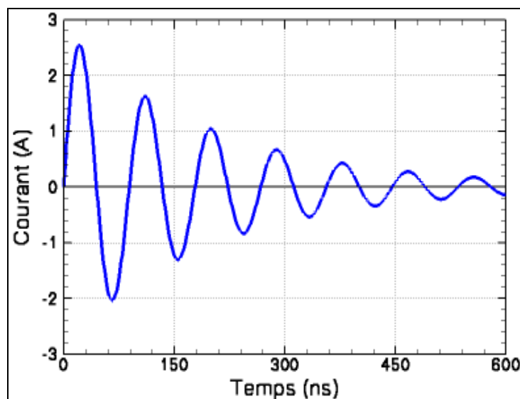
Figure 4: Forme d'onde en courant d'une décharge MM de 200 Volts.
