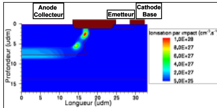
Figure 88: Distribution du taux d'ionisation par impact au point TLP ( V=40,4\text{ V} ; I=1,52\text{ A} ).
