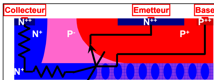
Figure 25: Coupe technologique d'un transistor NPN vertical avec couches enterrées diluée.
