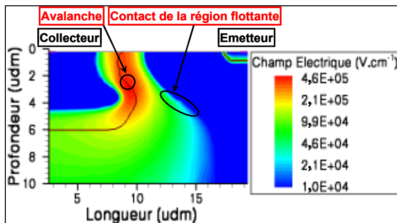
Figure 127: Distribution du champ électrique au claquage de la structure de référence (la région d'avalanche et la région où s'établit le contact avec la région flottante sont indiquées).
