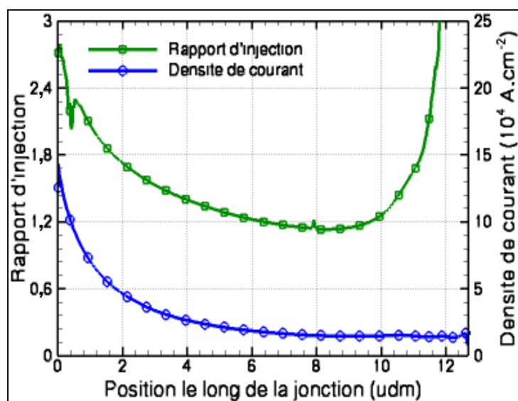
Figure 71: Rapport d'injection et densité de courant le long de la jonction émetteur-base pour un émetteur de longueur 12,7 \mu\text{m} .
