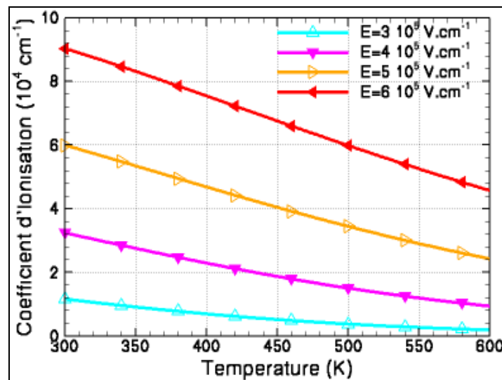
Figure 57: Coefficients d'ionisation des électrons suivant la température à des champs électriques de 3 \cdot 10^5 , 4 \cdot 10^5 , 5 \cdot 10^5 et 6 \cdot 10^5 V.cm -1 , d'après le modèle de Van Overstraeten - De Man [61].
