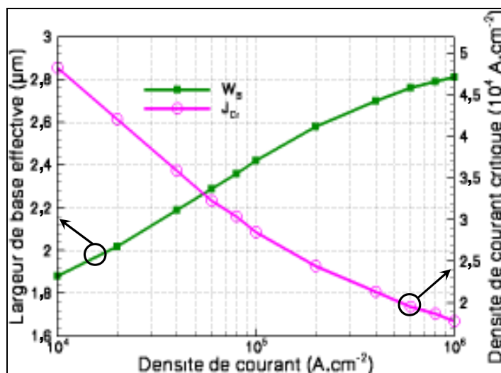
Figure 49: Largeur de base effective W_B et densité de courant critique J_{Cr} du transistor NPN pour des densités de courant allant de 10^4 à 10^6 \text{ A.cm}^{-2} .
