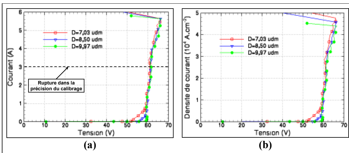
Figure 103: Caractéristiques TLP mesurées pour différentes distances D , en fonction du courant (a) et du courant ramené à la surface (b).
