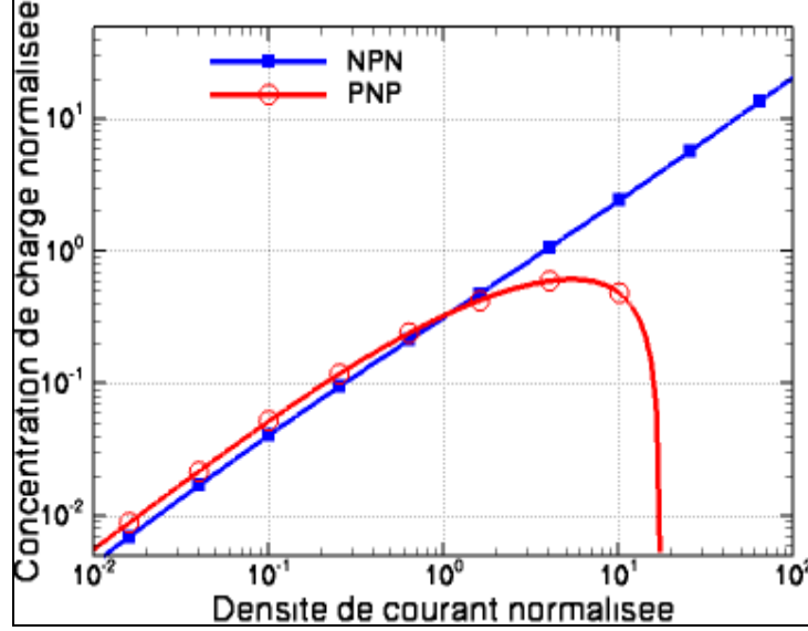
Figure 47: Concentration de charge normalisée ( p/p_{cr} ) suivant la densité de courant normalisée ( J/J_{Cr} ), d'après la formule (71).
