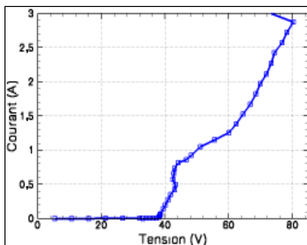
Figure 96: Caractéristique TLP de plus faible R_{ON} (surface 6,88 \cdot 10^3 \mu m^2 ).
