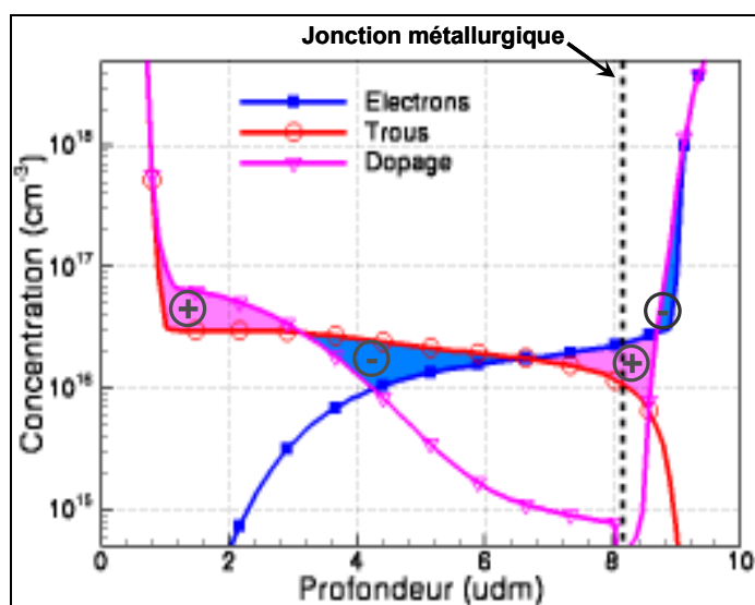
Figure 95: Distributions d'électrons, de trous et de dopants ionisés dans la diode au courant de 0,8 Ampères, faisant apparaître les charges d'espace positives (rouge) et négatives (bleu).
