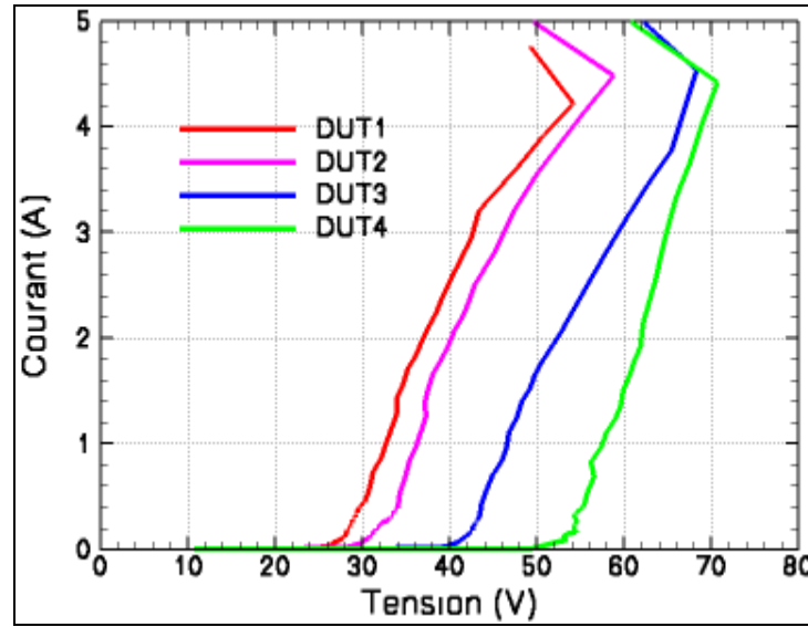
Figure 79: Caractéristiques TLP des composants DUT1-2-3-4 correspondants à une distance D croissante.
