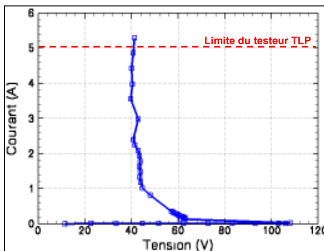
Figure 112: Caractéristique TLP mesurée.
