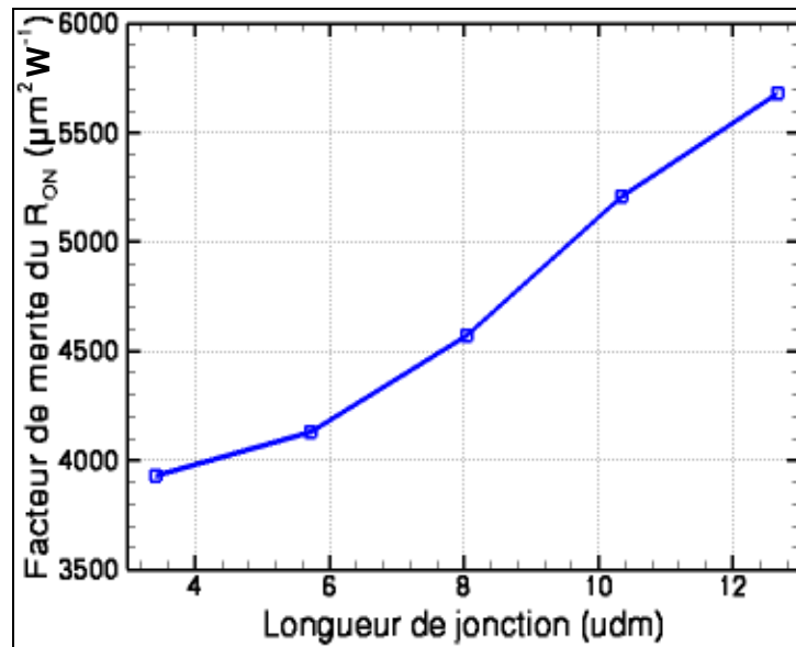
Figure 69: Facteur de mérite F_{ON} en fonction de la longueur de la jonction émetteur-base.
