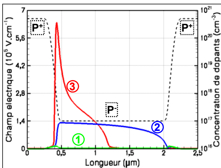
Figure 74: Distributions champ électrique en régime ohmique (1), en régime saturé (2) et pour J > J_{Max} (3).
