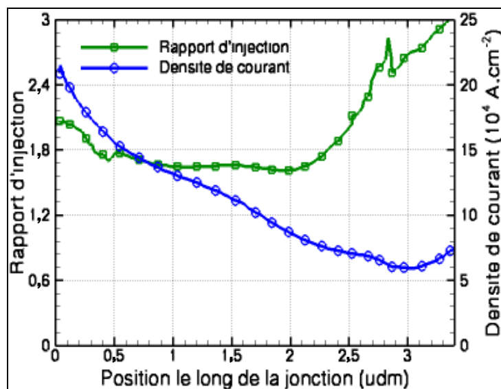
Figure 70: Rapport d'injection et densité de courant le long de la jonction émetteur-base pour un émetteur de longueur de 3,4 \mu\text{m} (la partie gauche du graphe est côté collecteur et la partie droite côté base).
