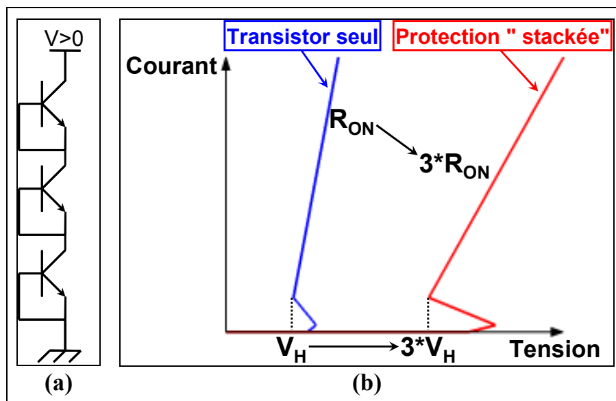
Figure 26: Schéma électrique de trois transistors NPN en série (a), et caractéristique I-V résultante (b).
