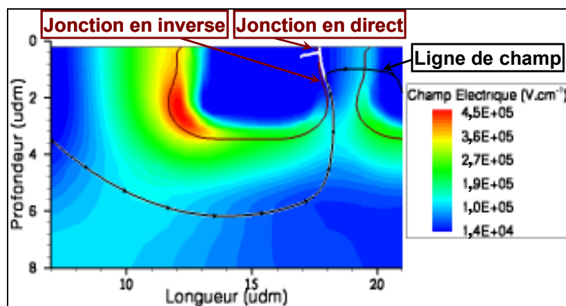
Figure 144: Distribution du champ électrique au voisinage de la région flottante au point TLP ( V=43,3 V ; I=73,4 mA), montrant les zones de la région flottante polarisée en direct et en inverse (séparées par les lignes blanches) et indiquant une ligne de champ suivie par les électrons (ligne noire).
