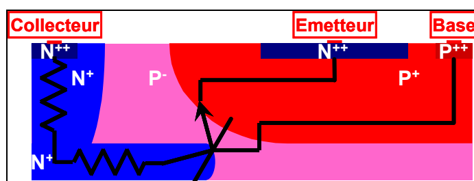
Figure 24: Coupe technologique d'un transistor NPN vertical avec couches enterrées partielle.
