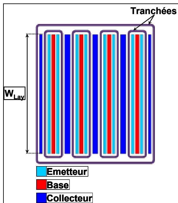
Figure 111: Layout schématique du transistor NPN testé montrant les tranchées profondes et les contacts.
