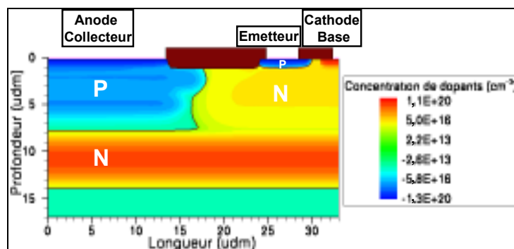
Figure 85: Profil de dopage de la structure retenue pour l'étude en simulation.
