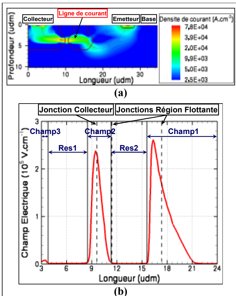
Figure 132: Distribution de la densité de courant dans le composant de distance 0,9 udm au point TLP ( V=33,7 V ; I=132 mA ) (a), montrant la ligne de courant pour tracer le profil du champ électrique (b).
