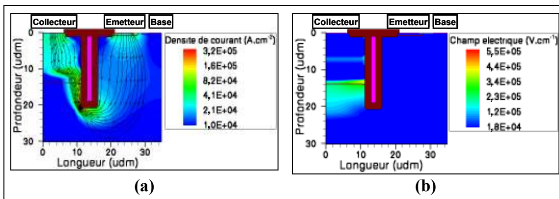
Figure 109: Distributions de la densité de courant, où les lignes de courants sont représentées, (a) et du champ électrique (b), au point TLP ( V=53 V ; I=690 mA).
