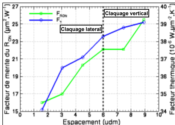
Figure 98: Facteur de mérite du R_{ON} à 1,5 \cdot 10^4 \text{ A} \cdot \text{cm}^{-2} et du facteur thermique en fonction de la distance D .
