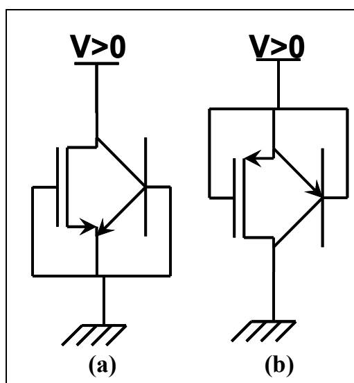
Figure 32: Schémas électriques équivalents d'un ggNMOS (a) et d'un guPMOS (b).
