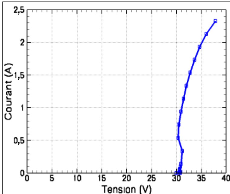
Figure 149: Caractéristique TLP simulée d'un transistor avec région flottante optimisée (surface 10^4 \mu m^2 ).
