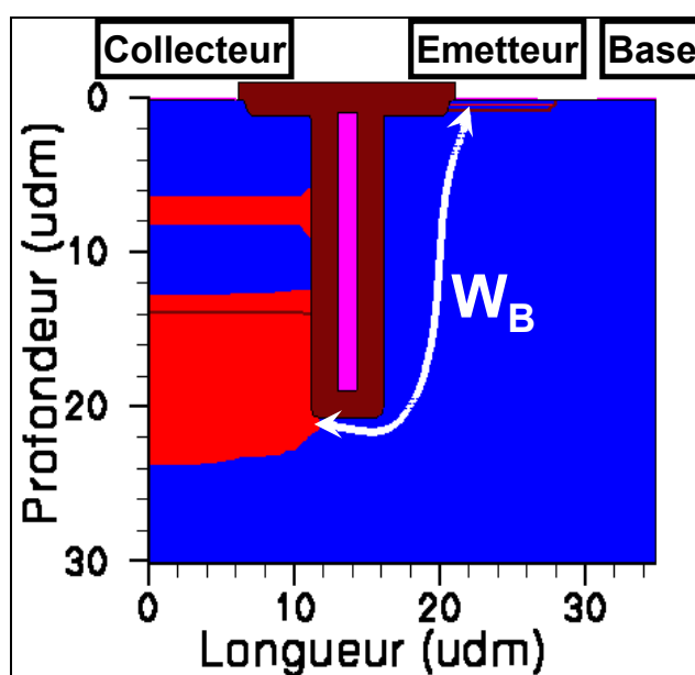
Figure 110: Répartition de la ZCE (rouge) au point TLP ( V=53 V ; I=690 mA), et ligne de courant dans la base représentative de la base interne W_B .
