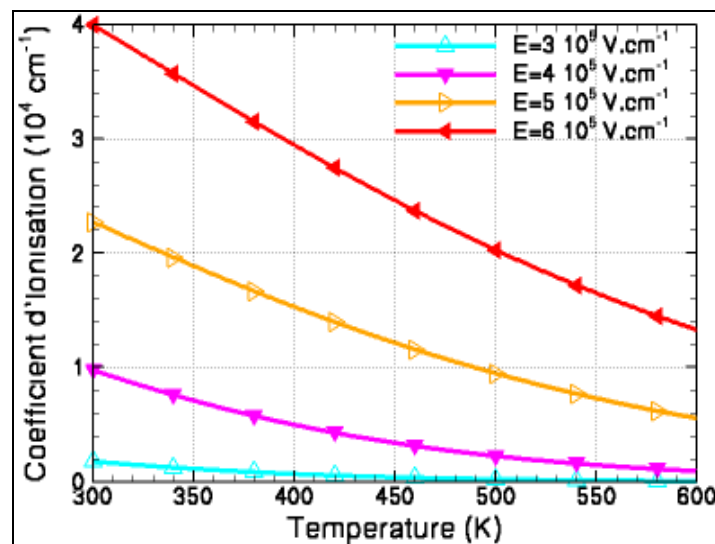
Figure 58: Coefficients d'ionisation des trous suivant la température à des champs électriques de 3 \cdot 10^5 , 4 \cdot 10^5 , 5 \cdot 10^5 et 6 \cdot 10^5 V.cm -1 , d'après le modèle de Van Overstraeten - De Man [61].
