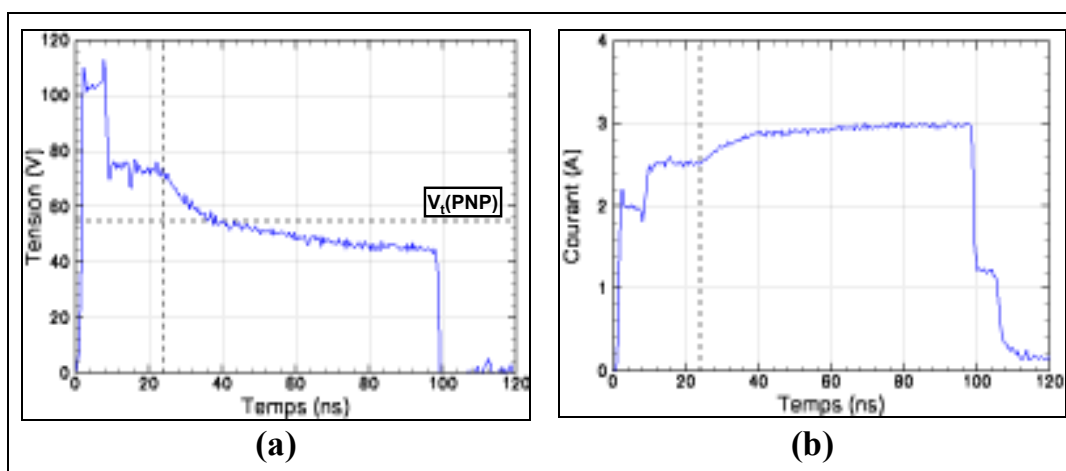
Figure 118: Oscillographes TLP de la tension (a) et du courant (b) pour le point ( V=41,4 V ; I=2,92 A) (mesure effective après les dix premières nanosecondes).
