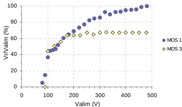
Figure 2-29 : pourcentage V_R/V_{\text{alim}} en fonction de la tension d'alimentation. Mesures pour le MOS 1 et le MOS 3.
