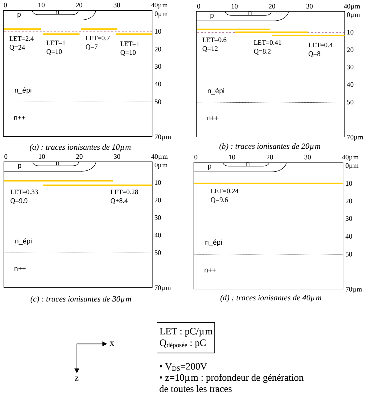
Figure 3-19: schématisation de traces ionisantes dans la demi-cellule de MOSFET polarisée à 200V. Les traces sont positionnées à la même profondeur z=10\mu\text{m} mais à différentes abscisses et sont simulées chacune indépendamment. La longueur des traces est de : (a) 10 \mu\text{m} , (b) 20 \mu\text{m} , (c) 30 \mu\text{m} et (d) 40 \mu\text{m} . Le LET est en pC/ \mu\text{m} et le range en \mu\text{m}
