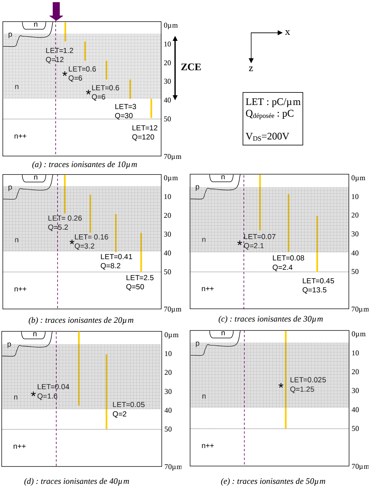
Figure 3-13: schématisation de traces ionisantes dans la demi-cellule de MOSFET polarisée à 200V. Les traces sont positionnées à la même abscisse x mais à différentes profondeurs et sont simulées chacune indépendamment. La longueur des traces est de : (a) 10 μm, (b) 20 μm, (c) 30 μm, (d) 40 μm et (e) 50 μm. Le LET est en pC/μm, la charge Q est en pC et le range en μm
