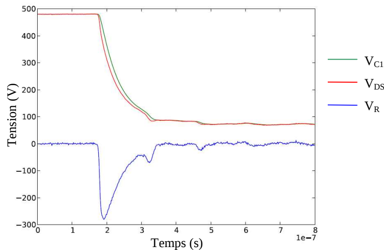
Figure 2-28 : acquisition de la tension V_R lors d'irradiations ions lourds sur le MOS 3. Tension V_{DS} et V_{C1} déduites par le calcul
