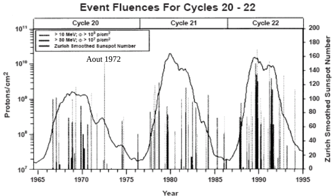
Figure 1-1: Cycles d'activité solaires. Corrélation entre les fluences de protons nés d'évènements solaires et le nombre de taches solaires pour les cycles 20 à 22. Le nombre de taches solaires est représenté par la courbe et les fluences de protons solaires par les lignes verticales. [BAR97]
