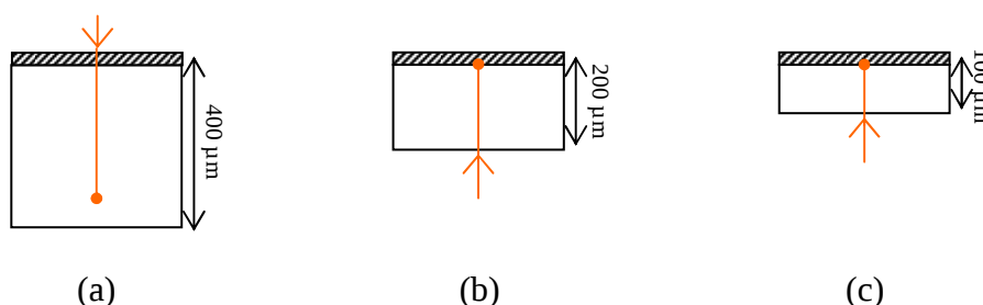
Figure 3-9: schémas des différentes ouvertures pour les tests ions lourds : (a) ouverture face avant pour les ions lourds, (b) ouverture face arrière avec amincissement de 200 \mu m, (c) ouverture face arrière avec amincissement de 300 \mu m
