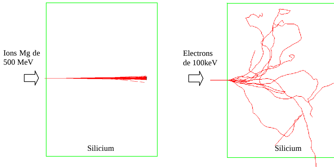
Figure 1-10: image du parcours d'ions magnésium d'énergie initiale 500 MeV et d'électrons d'énergie initiale 100 keV dans 500 \mu\text{m} de silicium
