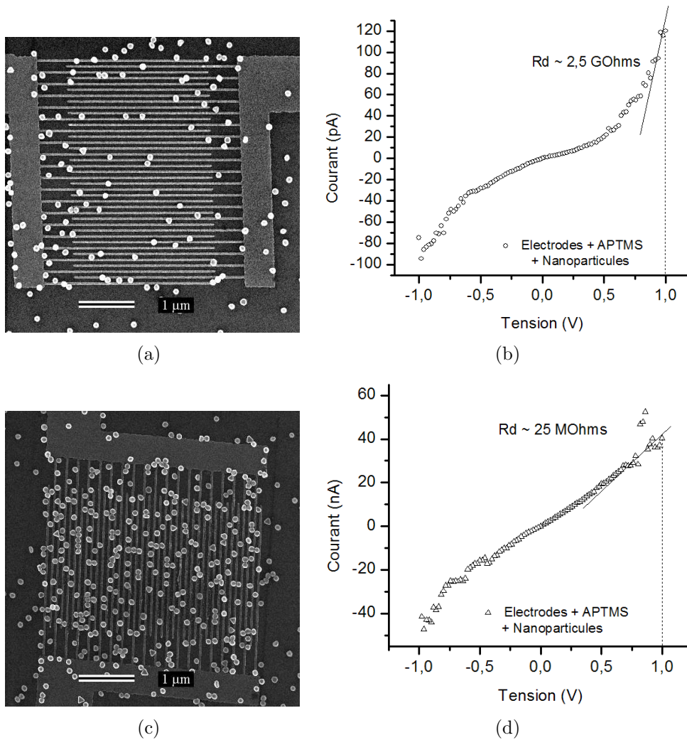
FIG. 3.27 – Deux exemples de dispositifs présentant des densités de dépôt différentes et les caractéristiques courant/tension associées.
