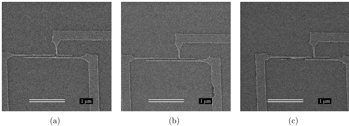
FIG. 2.24 – Exemples de réalisation de dispositifs à trois électrodes pour trois doses différentes 6nC/cm (a), 8nC/cm (b), 11nC/cm (c).
