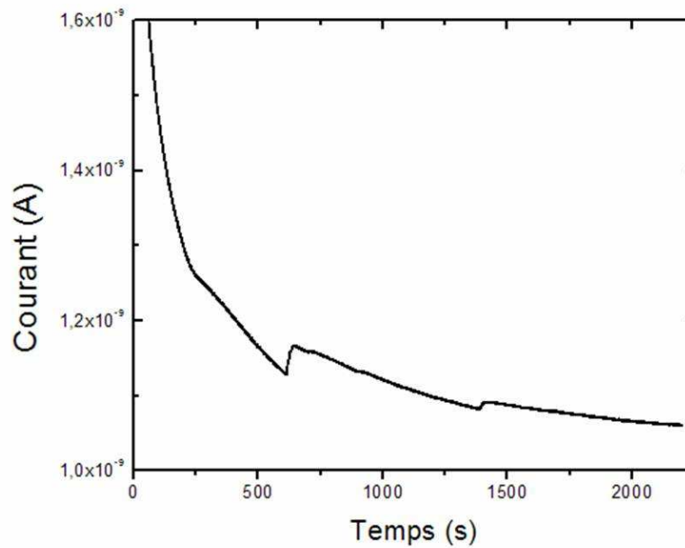
FIG. 3.34 – Caractéristiques I(t) du dispositif en lors de l'incubation de la solution de nanoparticules de 100nm de diamètre sous une tension de polarisation de 1V. Le dispositif est un réseau d'électrodes interdigitées de 100nm de pas et d'espace inter-électrodes de 65nm et a été fonctionnalisé par de l'APTMS avant l'assemblage d'un micro-cuve en PDMS.
