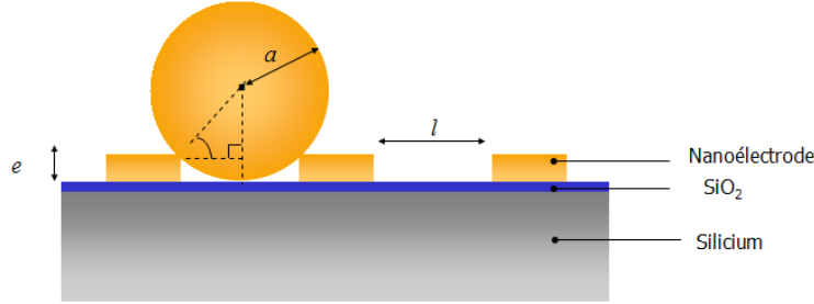
FIG. 3.12 – Adaptation des dimensions des dispositifs satisfaisant aux conditions de "pontage" des électrodes par les nanoparticules d'Or. l représente l'espace inter-électrode, e l'épaisseur des électrodes et a le rayon des nanoparticules
