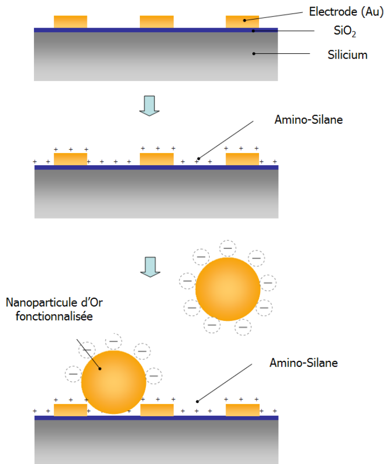
FIG. 3.2 – Description schématique de la stratégie de détection de nanoparticules métalliques déposées sur un réseau de nanoélectrodes interdigitées.
