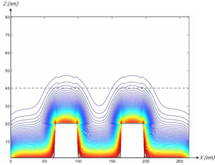
FIG. 3.22 – Tracé des lignes équipotentiellles (unités arbitraires) décrivant les variations du potentiel attractif exercé par la surface à proximité d'un réseau d'électrodes interdigtées de 65nm de large, au pas de 100nm et de 20nm d'épaisseur.
