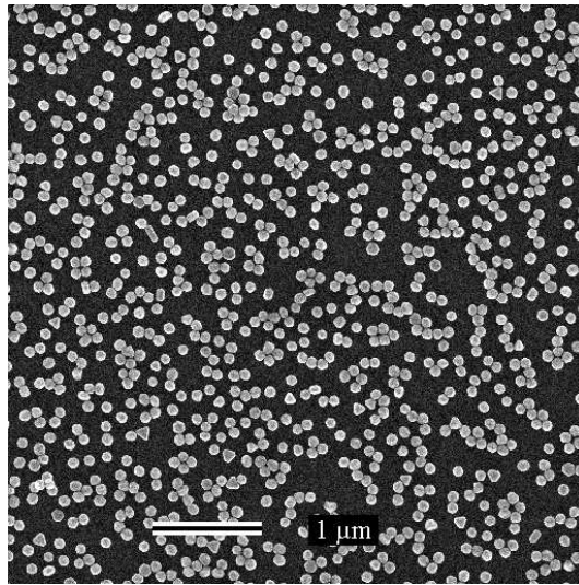
FIG. 3.6 – Image MEB d'une surface de silice fonctionnalisée par de l'APTMS après 2 heures d'incubation d'une solution de nanoparticules d'Or stabilisées par des groupes citrate. Le diamètre moyen des particules est de 100nm. La densité obtenue est d'environ 4.10^9\text{particules}/\text{cm}^2
