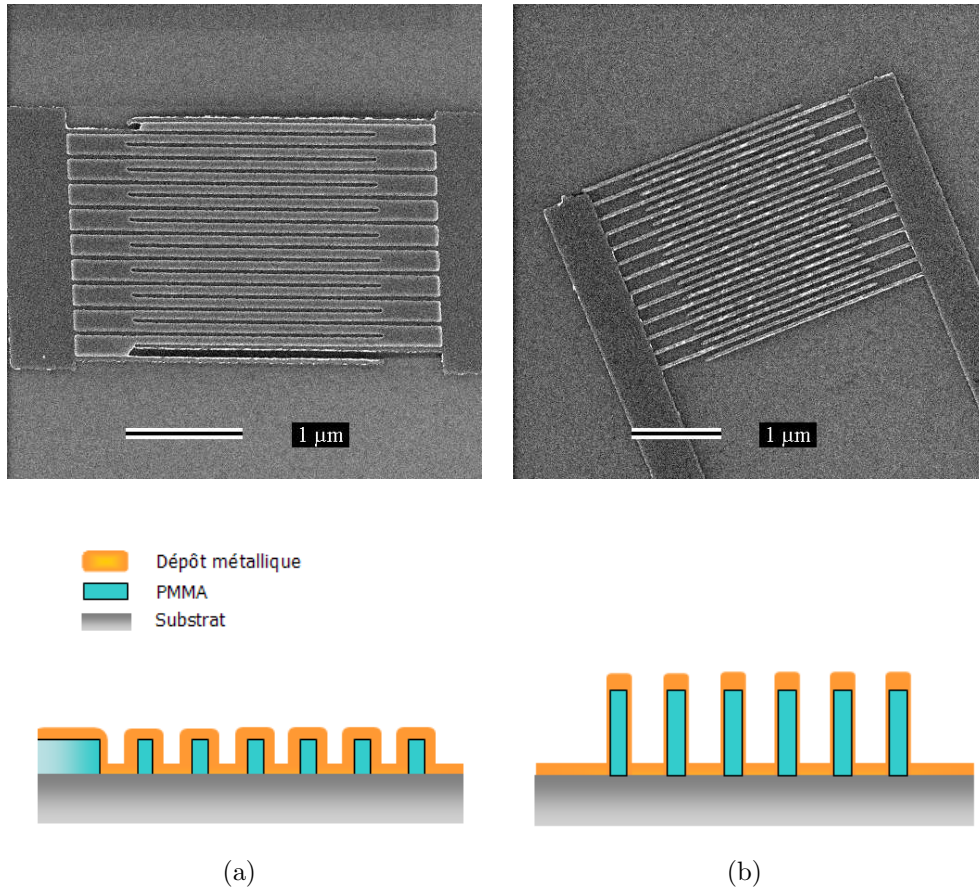
FIG. 2.16 – Influence de l'épaisseur de résine sur la réalisation du lift-off pour des électrodes inter-digitées au pas de 100nm insolées avec une dose de 7\text{nC/cm} . Une épaisseur de résine de 50nm (a) est insuffisante pour la réalisation du lift off. L'utilisation d'une épaisseur de 130nm (b) permet de diminuer l'épaisseur de résine présente sur les flancs des structures et réaliser le lift-off.
