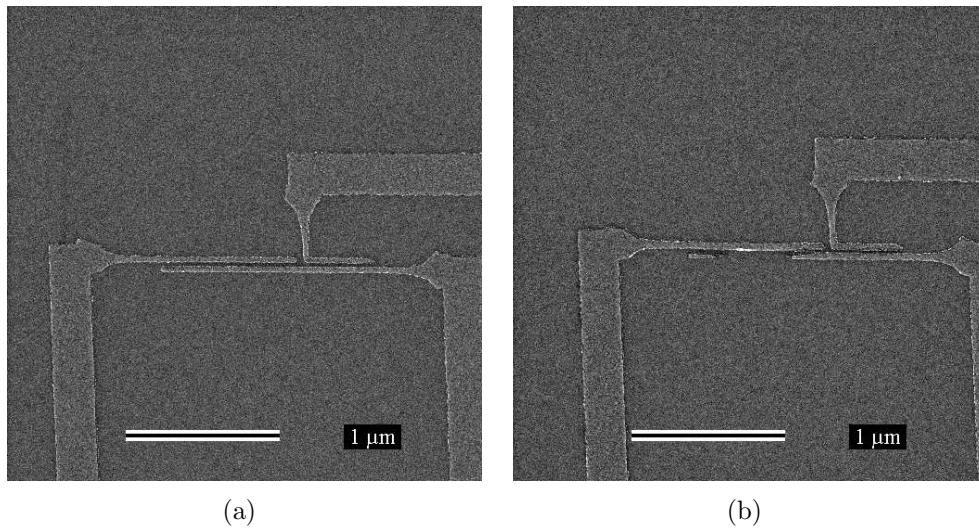
FIG. 2.13 – Illustration de l'influence de l'épaisseur de résine. Les deux structures ont été insolées avec une dose de 8\text{nC/cm} . Dans le cas (a) l'épaisseur de résine est de 100\text{nm} et de 140\text{nm} dans le cas (b).
