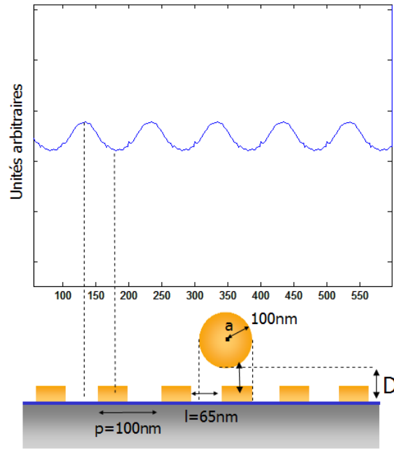
FIG. 3.23 – Variations relatives de l'énergie d'interaction électrostatique entre une particule chargée de 100\text{nm} de diamètre sur une réseau d'électrodes de 65\text{nm} de large au pas de 100\text{nm} et de 20\text{ nm} d'épaisseur. Le profil a été obtenu suivant un axe perpendiculaire aux électrodes pour une séparation entre la particule et le substrat de 25\text{nm} .
