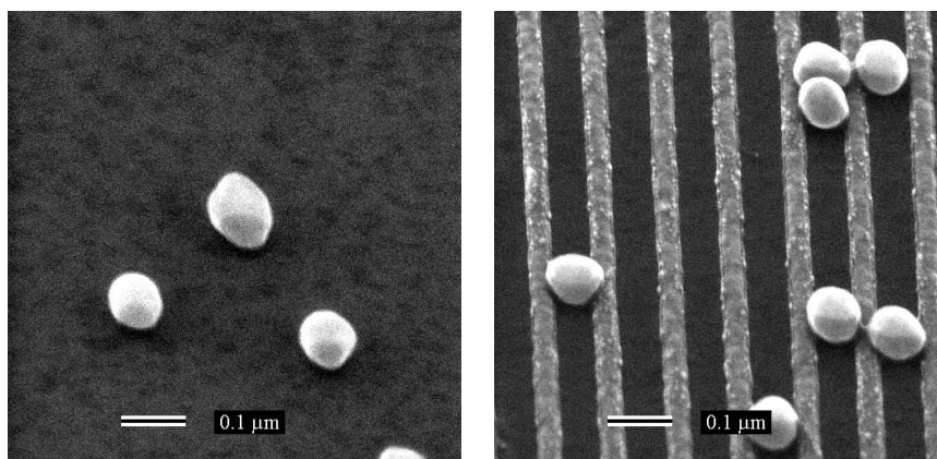
FIG. 4.10 – Exemple d'observation MEB à fort grandissement de particules d'Or fonctionnalisées par des molécules de type anti-biotine et déposées sur dispositif après interaction cible-sonde sur une surface de silice (a) et sur un réseau d'électrodes (b).
