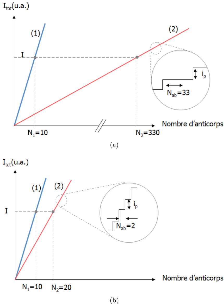
FIG. 4.18 – Comparaison des réponses électriques de deux dispositifs de type réseaux d'électrodes interdigitées aux pas de 100nm (a) et 40nm (b) pour lesquels sont utilisées respectivement des particules de 78 et 20 nm de diamètre. Les valeurs de courant sont exprimées en multiple de i_p
