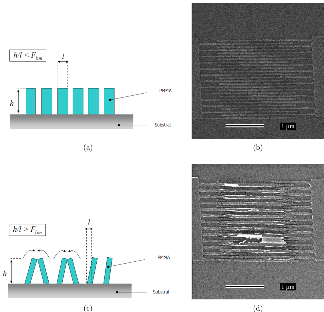
FIG. 2.12 – Illustration de l'influence des facteurs de formes des structures. Les structures présentées ont été obtenues dans une couche de PMMA de 140nm d'épaisseur après développement dans une solution de MIBK/IPA(1 :3) pendant 1 min 30s et lift-off. Les doses utilisées sont de 6nC/cm dans le cas (b) et de 14nC/cm dans le cas (d)
