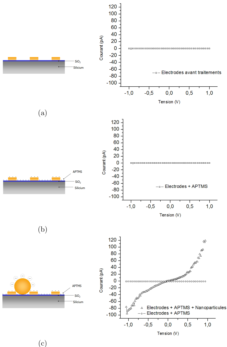
FIG. 3.26 – Évolution des caractéristiques courant(pA) - tension(V) d'un dispositif basé sur un réseau d'électrodes interdigitées au cours des étapes menant au dépôt de nanoparticules d'Or Dispositif avant traitement (a), après silanisation lavage et séchage (b), après dépôt des particules (c), lavages et séchage. Les 39 électrodes présentent une épaisseur de 20nm sont espacées de 65nm. Le diamètre moyen des particules est de 100nm.
