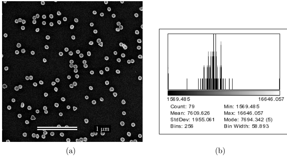
FIG. 3.13 – Image MEB d'un dépôt de nanoparticules (Grandissement 30k\times ). Le diamètre moyen a été évalué à 98nm avec une dispersion moyenne de \pm 15nm .
