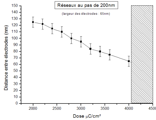
FIG. 2.23 – Courbe d'évolution de la valeur de l'espace inter-électrodes en fonction de la dose d'insolation pour un réseau d'électrodes interdigitées aux pas de 200nm obtenus par insolation dans une couche de PMMA (996000) de 300nm d'épaisseur après développement dans une solution de MIBK/IPA (1 : 3), dépôt d'une couche de 20nm d'Or et lift-off.
