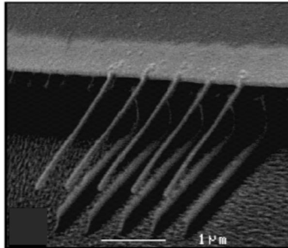
FIG. 1.10 – Image MEB d'un réseau de bras de levier nanométriques en Chrome (longueur : 2\mu\text{m} , épaisseur : 50\text{nm} , largeur : 150\text{nm} ) [25].
