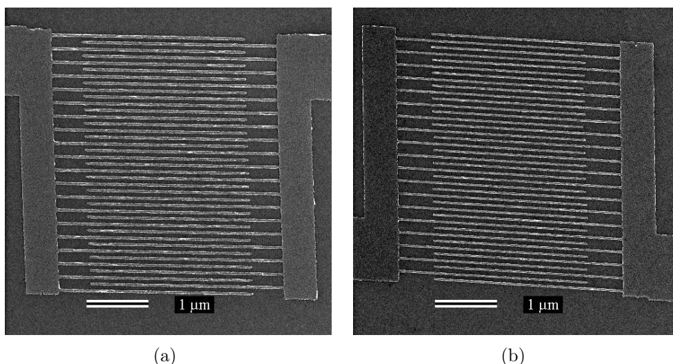
FIG. 2.25 – Images MEB de deux exemples de dispositifs de type réseaux d'électrodes interdigitées obtenus après insolation sous une dose de 7nC/cm dans une couche de PMMA(996000) de 140nm d'épaisseur, dépôt d'une couche d'Or de 20nm et lift-off. Dans le premier cas (a), le développement a été effectué dans une solution à 20 °C de MIBK/IPA (1 : 3) pendant 42s et dans une solution d'IPA pur à 20 °C sous d'ultrasons pendant 14s.
