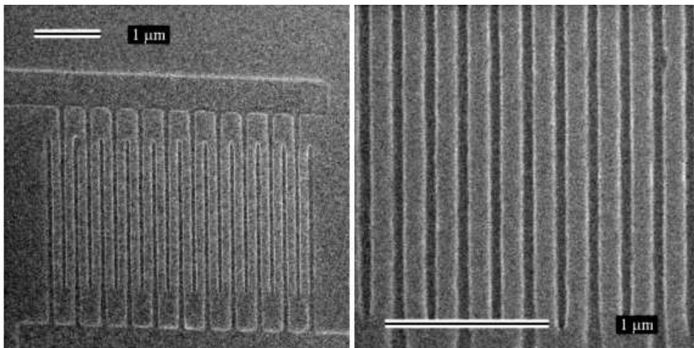
FIG. E.7 – Exemples de structures correspondants à des réseaux d'électrodes interdigitées au pas de 200nm et de 60nm de large répliquées dans un matériau polymère de type epoxy-siloxane [177]. Dans ces expériences, les moules ont été réalisés par lithographie électronique et gravure RIE du substrat. La hauteur des structures fabriquée est d'environ 100nm.
