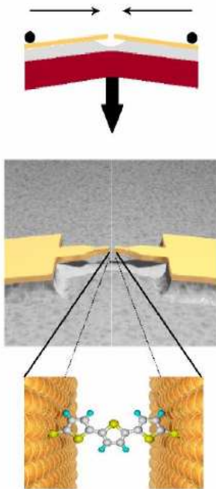
FIG. 1.16 – Illustration de la fabrication de nanjonctions par flexion sur un substrat déformable. Un fil suspendu est rompu par déformation du substrat. La distance inter-électrodes est ajustée en contrôlant cette déformation.
