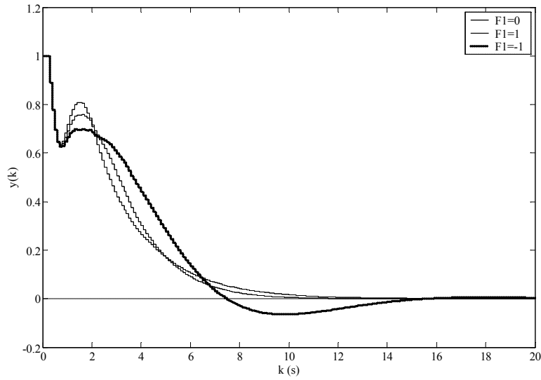
Figure 5.7. Réponse temporelle de la sortie y_1 pour F_l = -1, 0, 1
