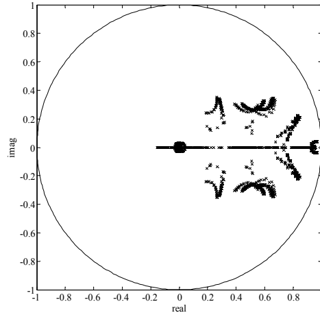
Figure 5.6. Localisation de pôles du système à boucle fermée pour k entre 0 et 10 s, et F_l entre -1 et 1 .
