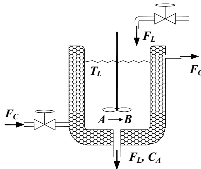
Figure 6.4. Réacteur.
