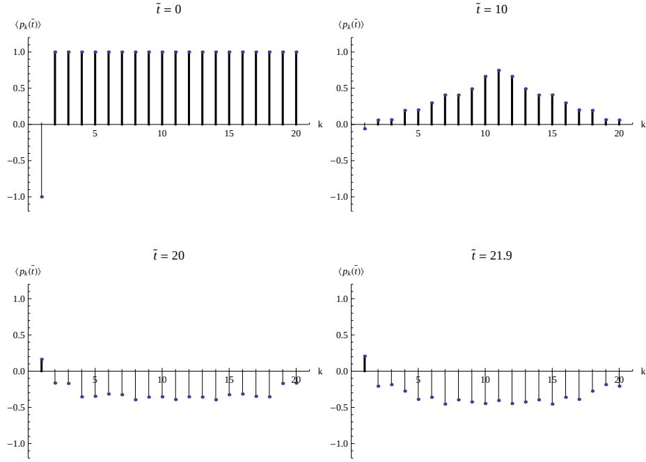
FIGURE 3.33 – Polarisation individuelles pour \hat{H}_3^{(C)} avec N_C = 20 spins pour \tilde{t} = 0, 10, 20 et 21.9 où le changement de la polarisation totale est maximal.
