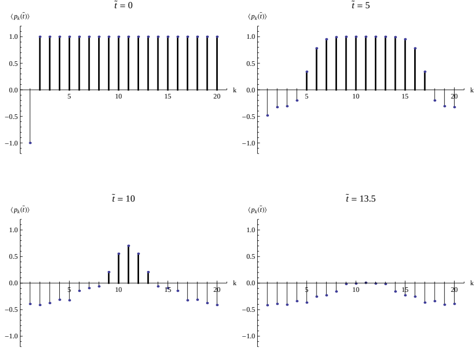
FIGURE 3.32 – Polarisation individuelles pour \hat{H}_2^{(C)} avec N_C = 20 spins pour \tilde{t} = 0, 5, 10 et 13.5 où le changement de la polarisation totale est maximal.
