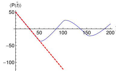
FIGURE 3.17 – Comparaison entre les polarisations totales moyennes : résultat exact (équation (3.22), courbe bleue continue) et terme linéaire de l'approximation WKB (équation (3.25), courbe rouge pointillée), pour N_L = 50 .
