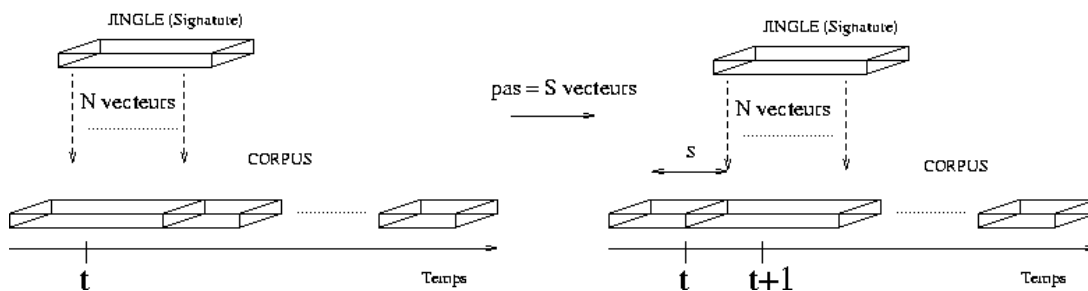
FIG. 4.4 – Comparaison entre le jingle et le corpus par distance Euclidienne.
