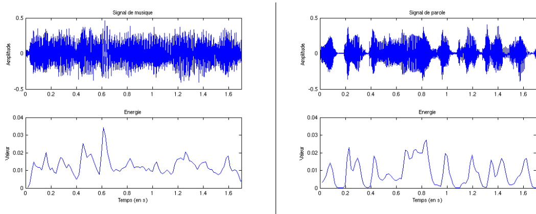
FIG. 1.4 – Évolution de l'énergie pour la musique et pour la parole sur 1,7 s.
