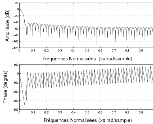
FIG. 3.3 – Réponse en fréquence et en phase du filtre RIF.
