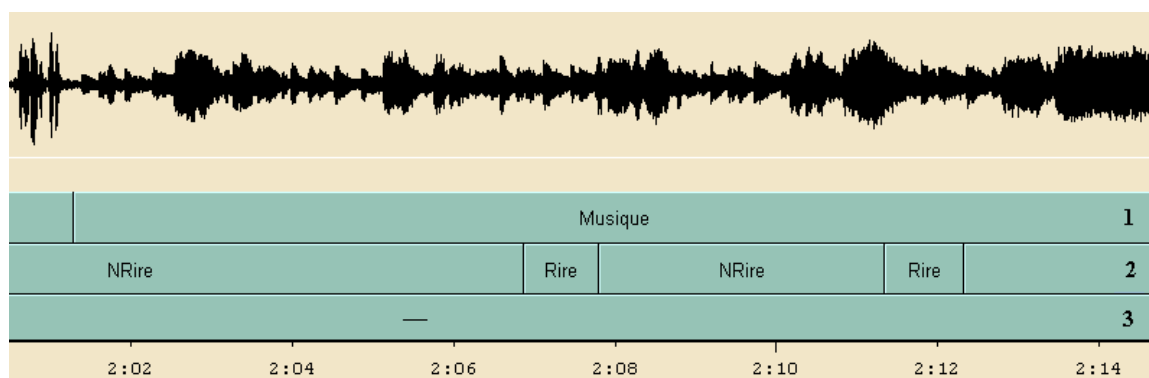
FIG. 5.6 – Suppression des étiquettes « rires » (ligne 3) grâce à l’apport d’information du système de classification musique/non-musique (ligne 1) sur le système de classification rires/non-rires (ligne 2). La durée des deux segments « Rire » est d’environ 1 s.
