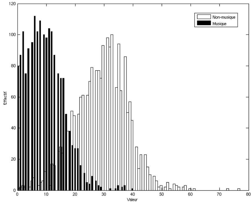
FIG. 3.13 – Distribution du nombre de segments par seconde pour la non-musique et pour la musique.
