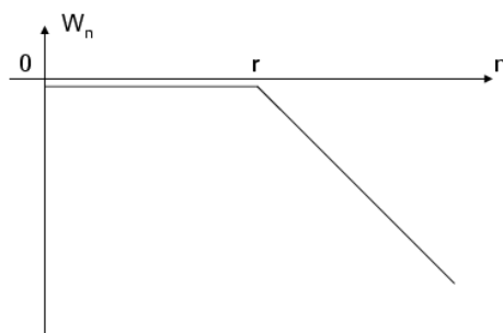
FIG. 3.7 – Variations de la somme cumulée W_n .
