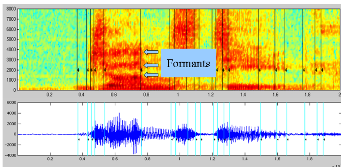
FIG. 1.1 – Spectrogramme de parole : alternance de sons voisés et non voisés sur 1,2 s de signal. Dans le cas voisé, une structure formantique est présente.
