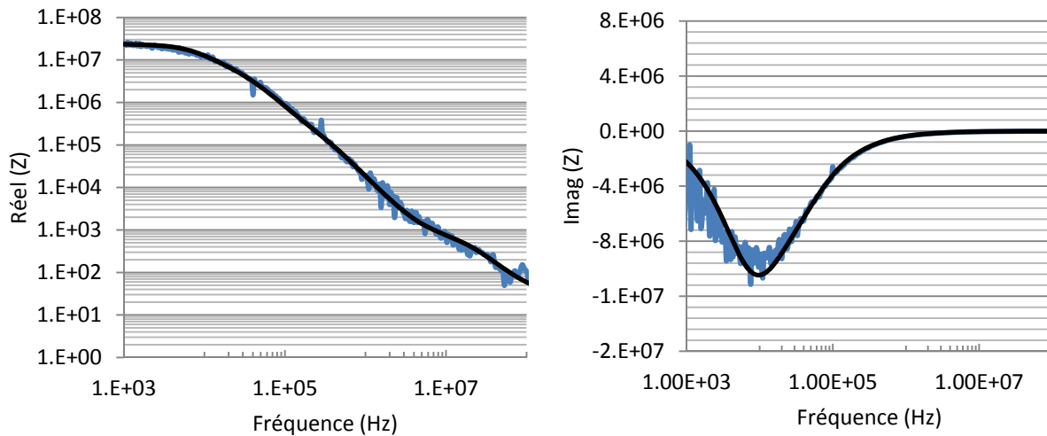
Figure II.31: comparaison du modèle localisé (noir) et de la mesure (bleu). (a) partie réelle de Z . (b) partie imaginaire de Z . Le dispositif est polarisé en mode diode ( V_{GS} = 0V ) avec le drain en circuit ouvert. Composant AEC1893
