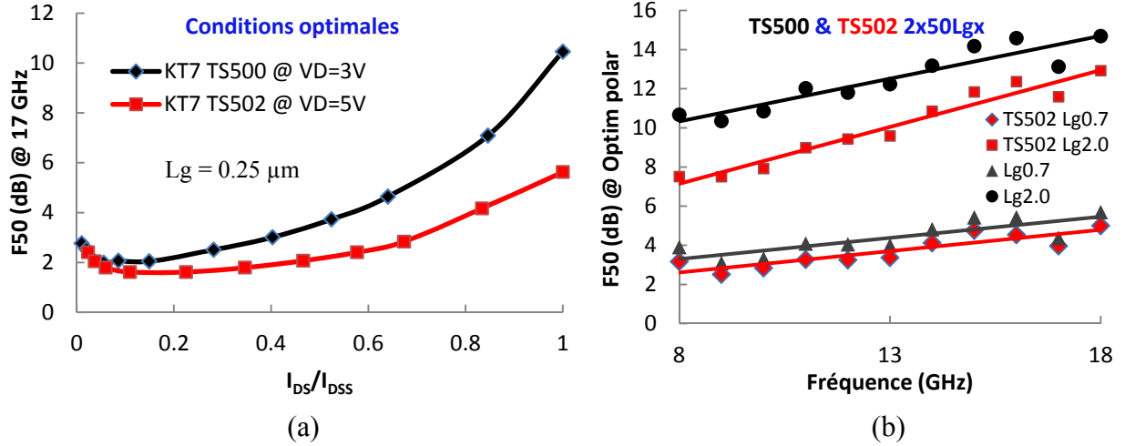
Figure III.29: Comparaison des F_{50} des composants TS500 et TS502. (a) L_g = 0.2 \mu m , en fonction de I_D/I_{DSS} à V_{DS} = 3 et 5V . (b) dans les meilleures conditions de polarisation pour différentes longueurs de grille.
