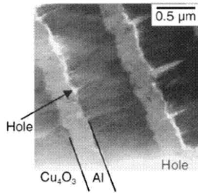
Figure 15. Multicouches \text{Cu}_4\text{O}_3/\text{Al} réalisées par PVD - observation au TEM [92]
