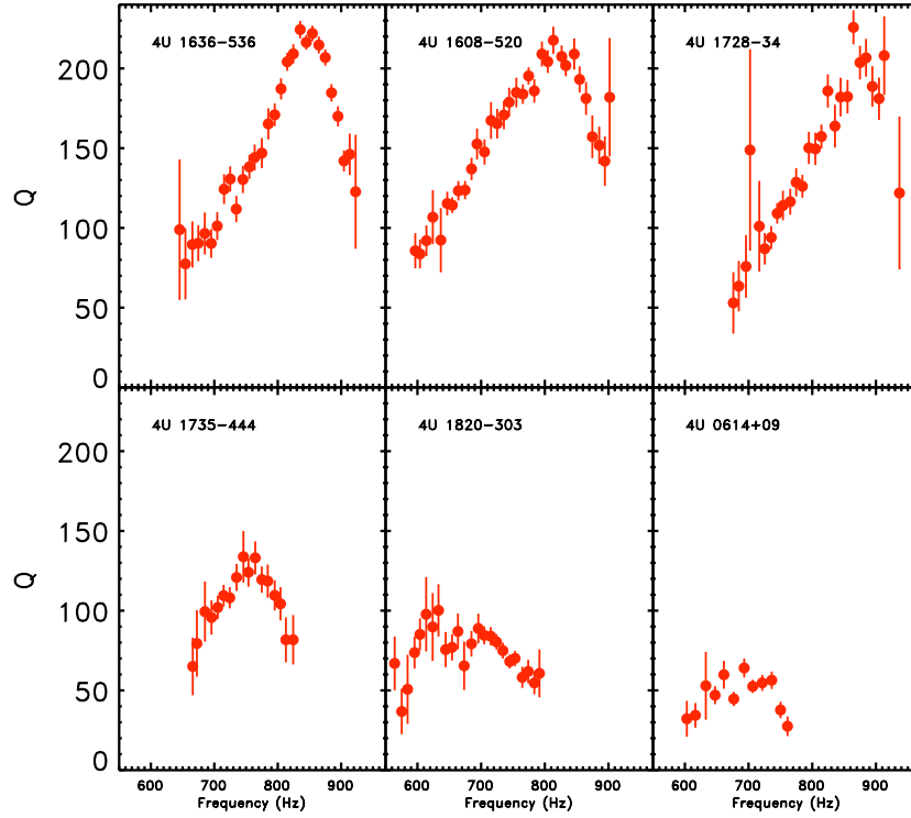
FIGURE 5.1 – Relation entre le facteur de qualité moyen et la fréquence du QPO kHz,1 pour les sources 4U 1636-536, 4U 1608-52, 4U 1728-34, 4U 1735-444, 4U 1820-303 et 4U 0614+09. Les observations ont été groupées par intervalle de fréquence de largeur comprise entre 10 et 25 Hz en utilisant la technique de shift-and-add. La chute du facteur de qualité à haute fréquence est clairement visible pour les 6 sources étudiées. Ce comportement est typique des QPO kHz,1 (voir Barret et al., 2006). On peut ainsi estimer précisément le facteur de qualité maximal pour chacune des sources.
