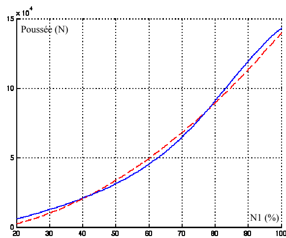
figure 3.3 : Comparaison entre le modèle de simulation, en rouge (précision par rapport au modèle OSMA : [-2.67\% ; 1.99\%] à 10^{-3} ) et le modèle de synthèse, en bleu. Le mach est de 0.06 (correspondant à une vitesse d'environ 30 kt), l'altitude est nulle et la température est standard ( \Delta ISA=0 ).
