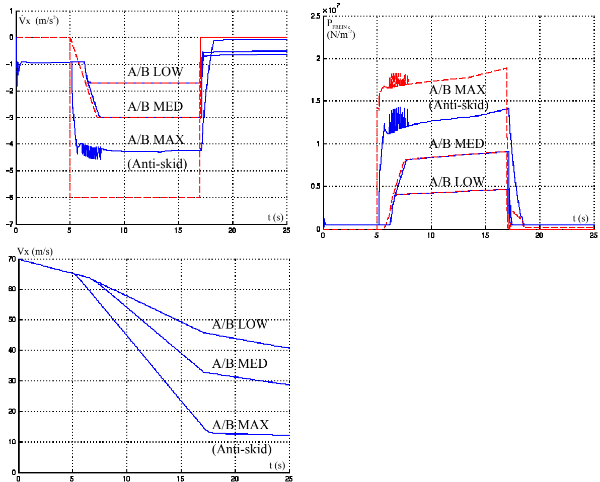
figures 3.26 a, b et c : Réponse obtenue avec une commande d'ordre 2, pour des sollicitations « autobrake » aux niveaux « LOW », « MED » et « MAX ».
