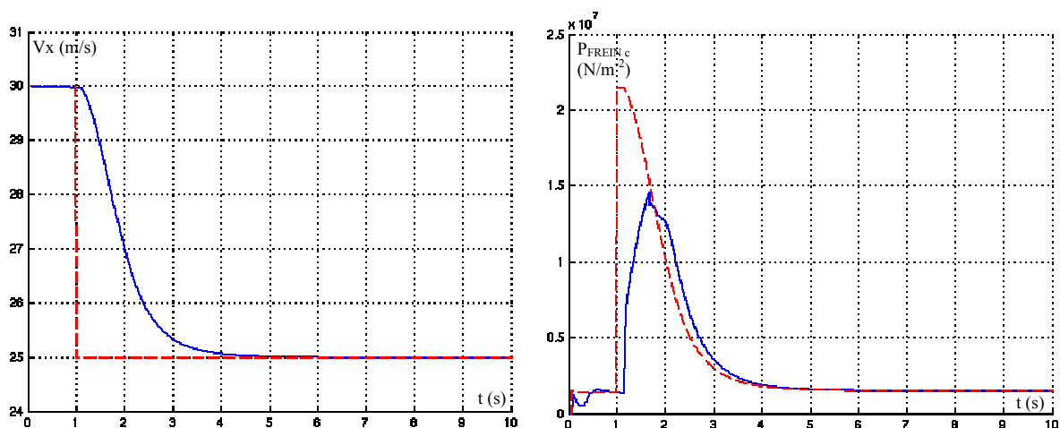
figures 3.15 a et b : Réponse obtenue pour une commande du 1 er ordre avec \omega = 1 et un régime moteur adapté à la consigne en vitesse.
