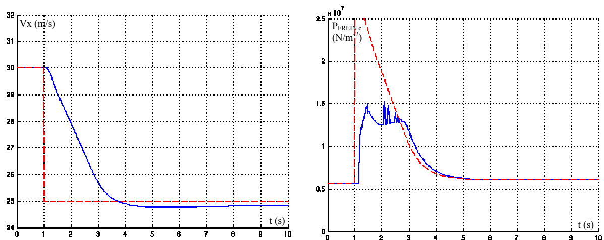
figures 3.19 a et b : Réponse obtenue pour une commande du 1 er ordre associée à un correcteur intégral et à un dispositif anit-windup ( \omega = 1 et N1 = 72\% ).
