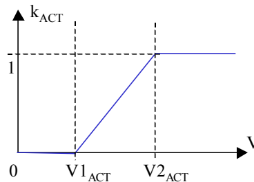
figure 4.1 : Exemple de fonction de répartition de la consigne entre roues avant et gouverne de direction.
