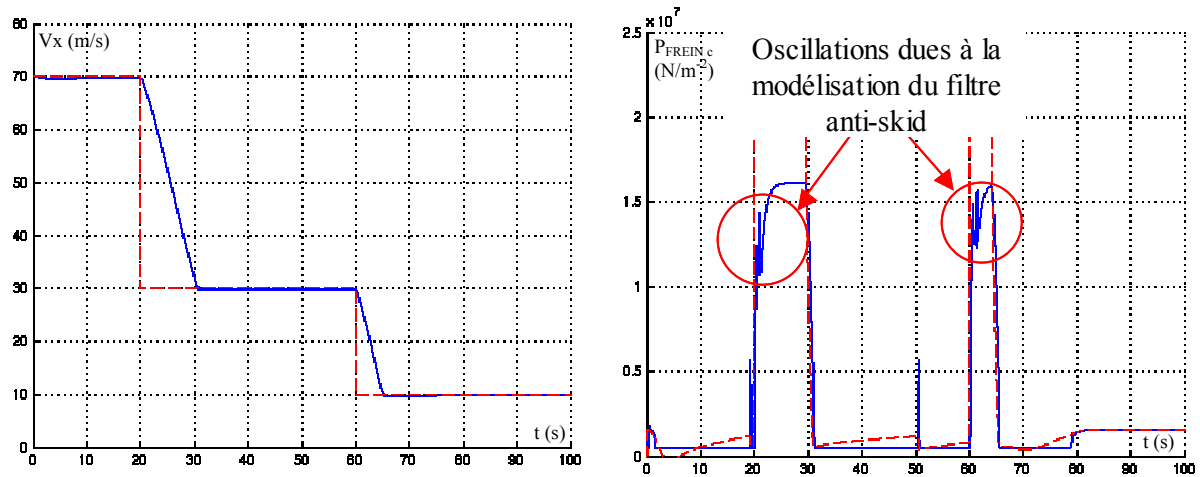
figures 3.14 a et b : Réponse obtenue pour une commande du 1 er ordre avec \omega = 1 et un régime moteur adapté à la consigne en vitesse.
