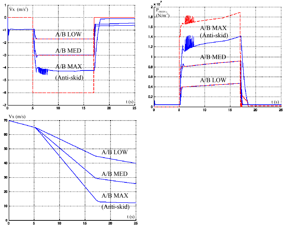
figures 3.24 a, b et c : Réponse obtenue avec une commande d'ordre 2, pour des échelons de décélération aux niveaux « LOW », « MED » et « MAX ».
