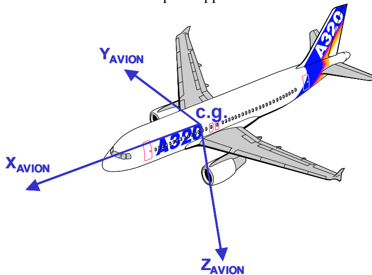
figure 1.1 : représentation du repère “avion”.
