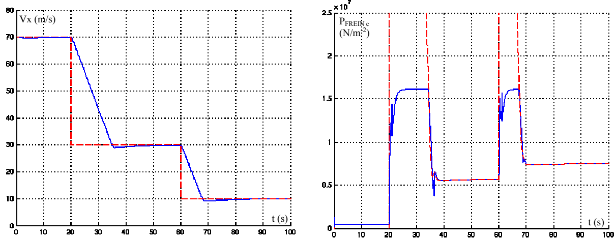
figures 3.18 a et b : Réponse obtenue pour une commande du 1 er ordre associée à un correcteur intégral et à un dispositif anti-windup ( \omega = 1 et N1 = 72\% ).
