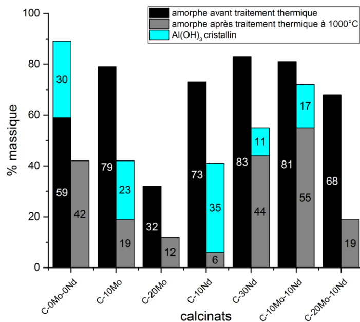
Figure 96 : Proportions massiques d'amorphe dans les calcinats avant et après traitement thermique à 1000 °C déterminées par DRX ex-situ associée à un affinement de type Rietveld. La présence de \text{Al}(\text{OH})_3 cristallin dans certains calcinats témoigne d'une hydratation pendant la phase de stockage.
