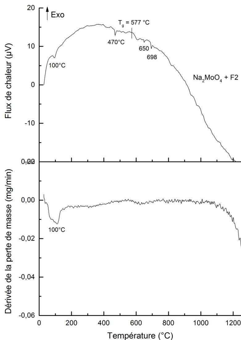
Figure 106 : Analyses thermiques différentielle et thermogravimétrique du mélange \text{Na}_2\text{MoO}_4 avec la fritte F2 pour un rapport masse fritte/masse verre (F/V) de 0,97.
