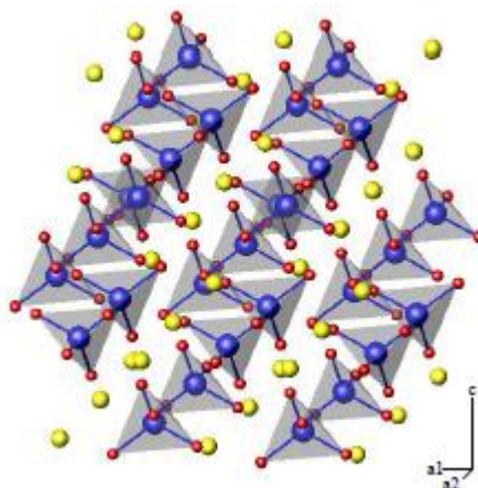
Figure 31 : Structure de la phase cristalline \text{CaMoO}_4 . Sphères bleues : cations \text{Mo}^{6+} ; Sphères jaunes : cations \text{Ca}^{2+} ; Sphères rouges : anions \text{O}^{2-} . Dans cette figure, la taille des sphères n'est pas tracée en fonction de la taille réelle des ions [54].
