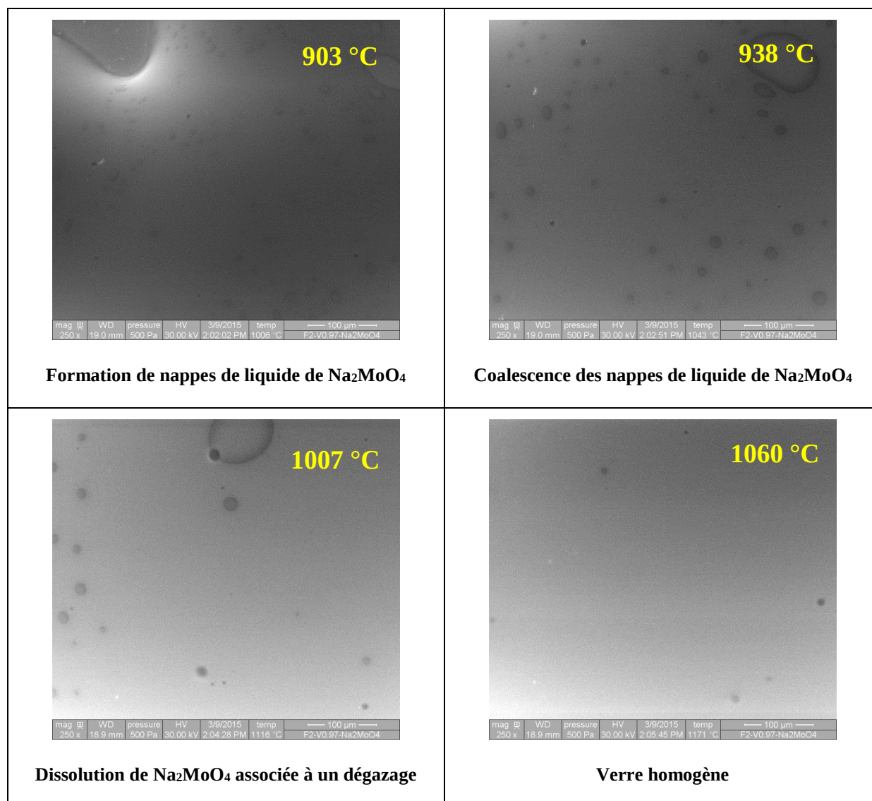
Figure 107 : Images acquises par microscopie électronique à balayage environnemental in-situ en température pour le mélange entre la fritte F2 et le composé pur Na 2 MoO 4 avec un rapport masse fritte/masse de verre (F/V) de 0,97 (rampe 50 °C/min ; sous air, avec une pression de 500 Pa).
