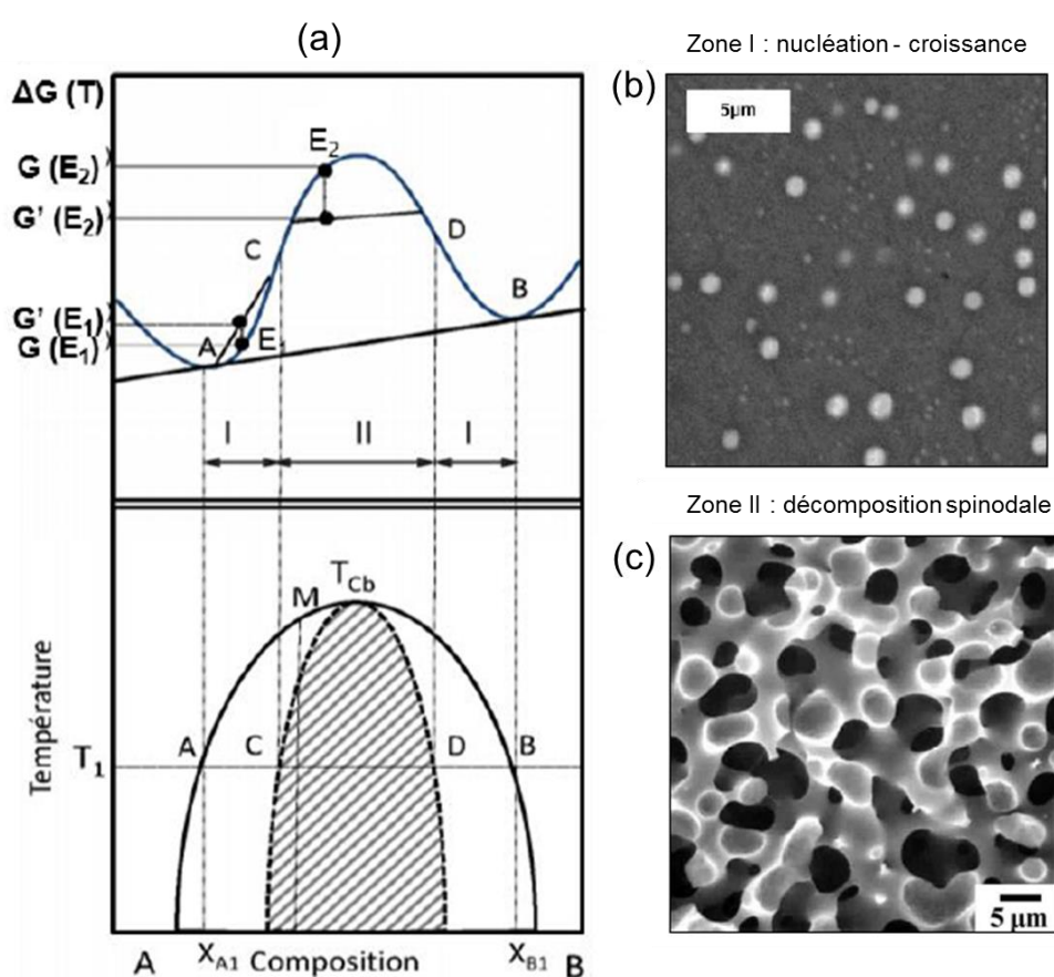
Figure 28 : (a) Evolution de la fonction \Delta G(T) d'un système binaire A-B lors d'une faible variation de composition autour des compositions E_1 et E_2 . Ces compositions appartiennent respectivement à la zone I qui correspond à une zone de nucléation-croissance (stable) et à la zone II qui correspond à une zone de décomposition spinodale (instable) ; Clichés MEB de phases séparées produites (b) par nucléation-croissance dans un verre borosilicaté enrichi en \text{MoO}_3 , \text{P}_2\text{O}_5 , \text{ZrO}_2 et \text{CaO} [58] (c) par décomposition spinodale dans un verre poreux de type Shirasu contenant \text{ZrO}_2 [59] d'après [56].
