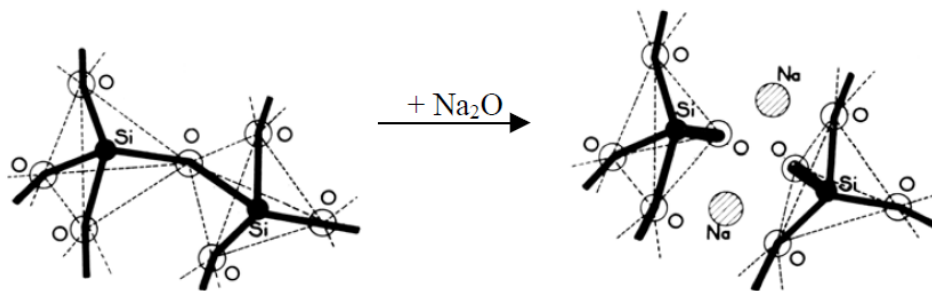
Figure 12 : Formation d'une paire d'oxygènes non-pontants par introduction d'une molécule de \text{Na}_2\text{O} dans un verre de silice [1].
