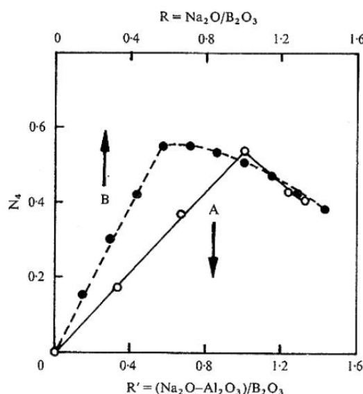
Figure 24 : Variation de N_4 en fonction du rapport R' = ([Na_2O] - [Al_2O_3]) / [B_2O_3] (courbe A) ou du rapport R = [Na_2O] / [B_2O_3] (courbe B) des verres de compositions 30SiO_2-30B_2O_3-[0-25]Al_2O_3-[40-15]Na_2O [38].
