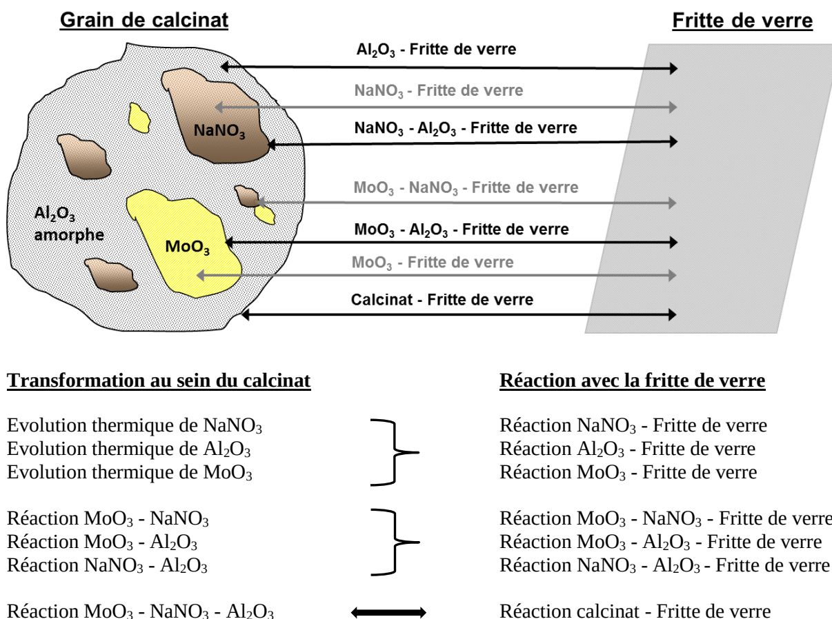
Figure 42 : Schéma descriptif des réactions possibles au sein d'un calcinat enrichi en oxyde de molybdène et lors de l'interaction avec la fritte de verre.
