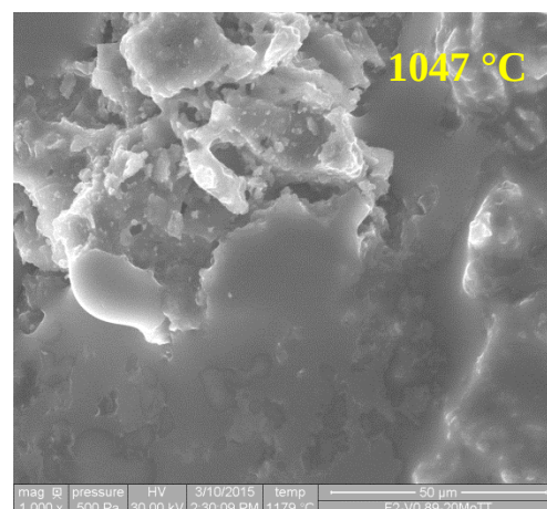
Formation de nappes de liquide de \text{Na}_2\text{MoO}_4
