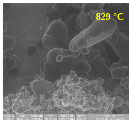
Ramollissement de la fritte de verre
