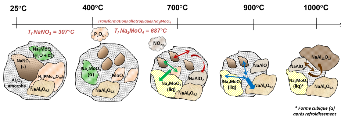
Figure 94 : Schématisation du mécanisme de transformation d'un calcinat appartenant au système ( \text{Na}_2\text{O}-\text{Al}_2\text{O}_3-\text{MoO}_3 ) lors d'une élévation de température de 25 °C à 1100 °C.
