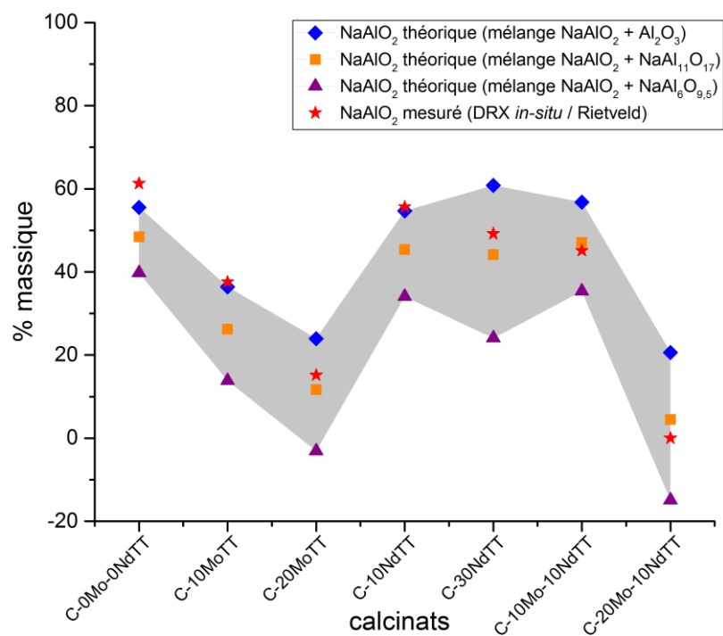
Figure 100 : Pourcentages massiques théoriques de \text{NaAlO}_2 considéré en mélange avec \text{Al}_2\text{O}_3 pur ou \text{NaAl}_{11}\text{O}_{17} ou \text{NaAl}_6\text{O}_{9,5} et pourcentages massiques mesurés par DRX in-situ associée à un affinement de type Rietveld pour chaque calcinat.
