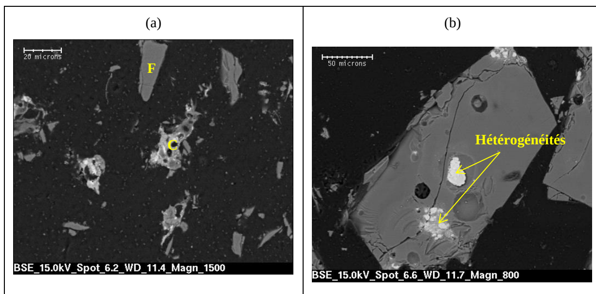
Figure 51 : Images MEB représentant (a) une vue d'ensemble de l'échantillon après un traitement de 5 minutes à 700\text{ }^{\circ}\text{C} du mélange entre C-20MoTT (noté C) et la fritte de verre F2 (notée F); (b) un grain de fritte de verre présentant des hétérogénéités après un traitement de 5 minutes à 1000\text{ }^{\circ}\text{C} .
