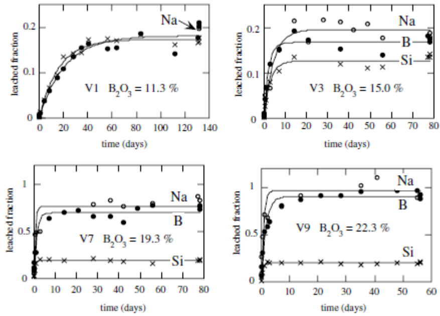
Figure 41 : Cinétiques de dissolution de quatre verres pour un rapport surface spécifique du verre/volume de la solution de S/V = 100 \text{ m}^{-1} . Les concentrations dissoutes sont tracées en fonction du temps pour Si (X), B (●) et Na (○). Les lignes sont obtenues en ajustant les données avec l'Équation 29[115].
