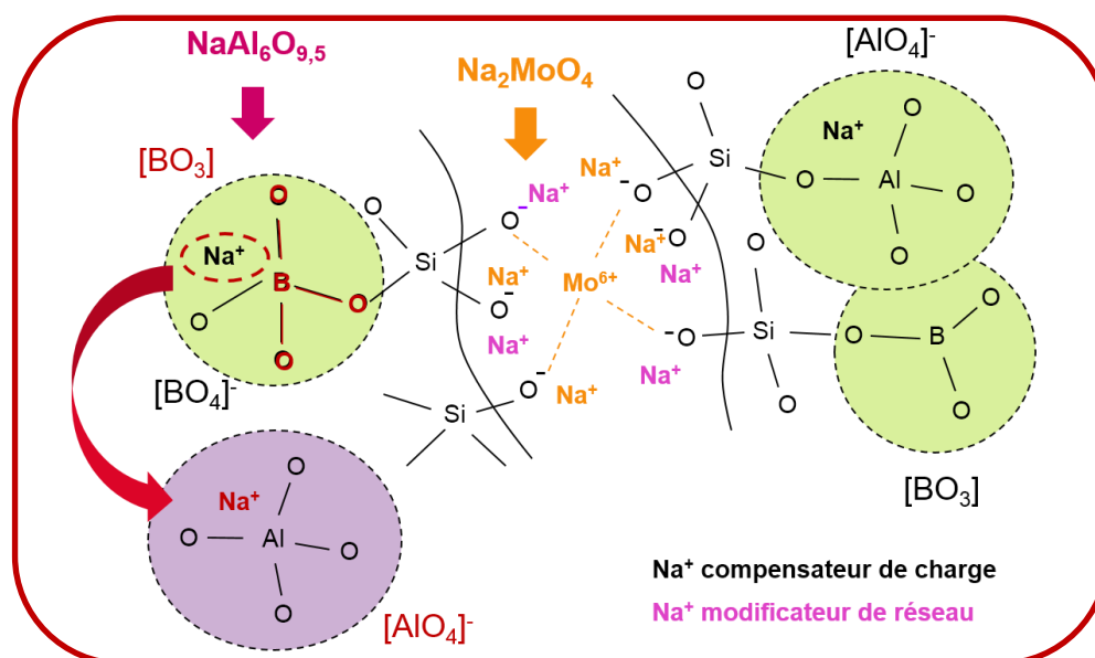
Figure 134 : Représentation schématique des modifications structurales du réseau borosilicaté induites lors de la dissolution des phases cristallines \text{NaAl}_6\text{O}_{9,5} et \text{Na}_2\text{MoO}_4 au cours de l'élaboration d'un verre simplifié contenant de l'oxyde de molybdène.
