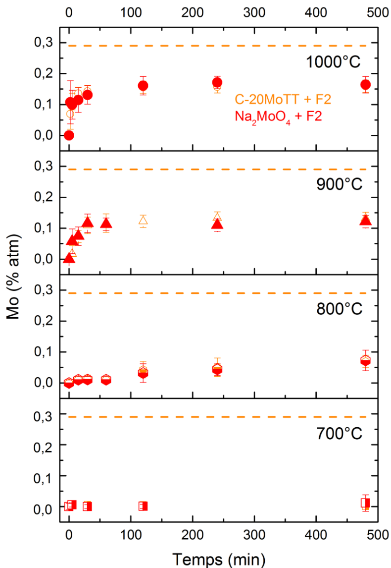
Figure 138 : Mise en évidence de l'indépendance de la dissolution du molybdène par comparaison des % atomiques en Mo incorporés dans le verre déterminés par analyses microsonde des verres issus des tests de réactivité entre la fritte de verre F2 et le calcinat C-20MoTT ou le composé pur de Na 2 MoO 4 .
