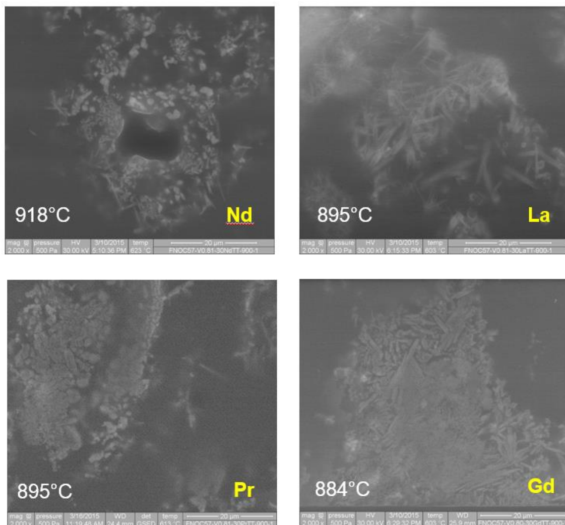
Figure 142 : Clichés acquis après 5minutes à 900 °C hors du MEB-Environnemental sur des mélanges FNOC57+C-30TRTT (TR= Nd, La, Pr et Gd) mettant en évidence la cristallisation de \text{Ca}_2\text{TR}_8(\text{SiO}_4)_6\text{O}_2 .
