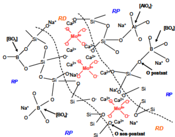
Figure 26 : Schéma structural d'un verre aluminoborosilicaté contenant du molybdène [54]. Les entités tétraédriques [MoO_4]^{2-} sont localisées dans les régions dépolymérisées de la structure du verre. Les lignes en pointillés séparent les régions polymérisées (RP) des régions dépolymérisées (RD)(Figure issue de [55]).
