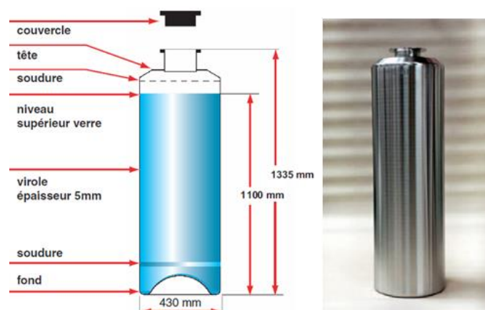
Figure 3 : Conteneur Standard de Déchets Vitrifiés CSD-V [27].
