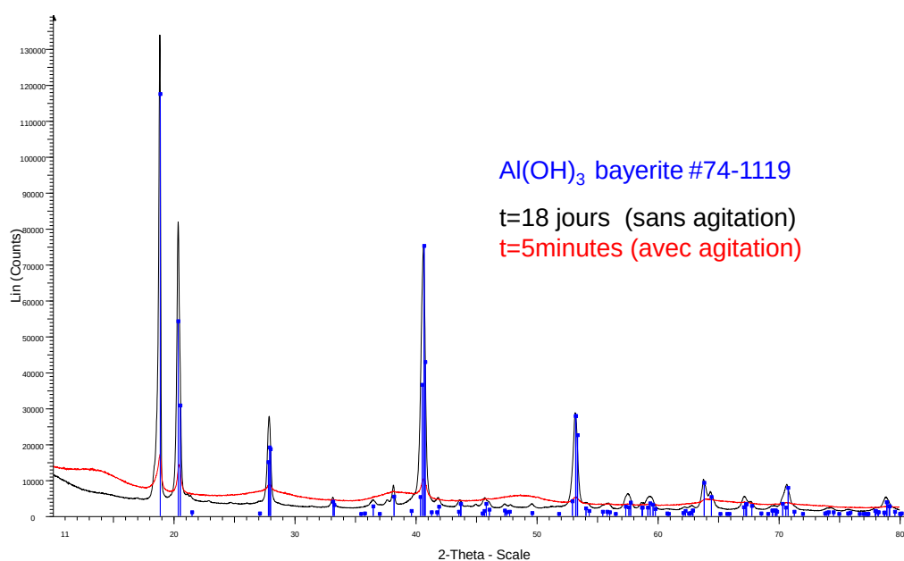
Figure 74 : Mise en évidence de l'hydratation de \text{NaAlO}_2 en \text{Al}(\text{OH})_3 par Diffraction des Rayons X. Tests réalisés à température ambiante à partir d'un mélange de \text{NaAlO}_2 commercial et d'eau ultra pure avec ou sans agitation et en fonction du temps. Le précipité a été filtré puis séché à 120 °C pendant une nuit.
