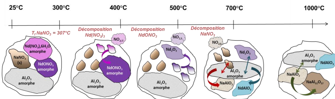
Figure 95 : Schématisation du mécanisme de transformation d'un calcinat appartenant au système ( \text{Na}_2\text{O}-\text{Al}_2\text{O}_3-\text{Nd}_2\text{O}_3 ) lors d'une élévation de température de 25 °C à 1000 °C.
