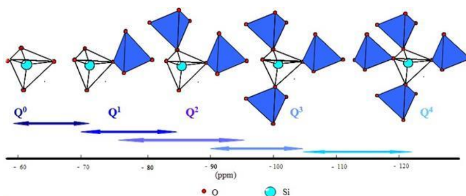
Figure 13 : Représentation des différentes configurations structurales \text{Q}^n ainsi que leur gamme de déplacements chimiques associée (en ppm).
