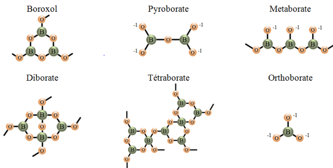
Figure 20 : Intermédiaires structuraux de types borates intervenant au sein des verres B_2O_3 - M_2O [24].
