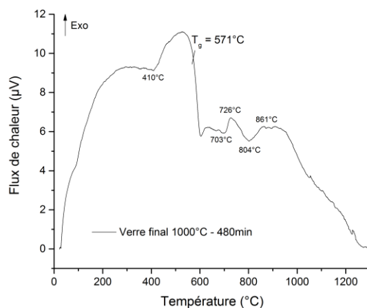
Figure 149 : Analyse thermique différentielle du verre final homogène issu du test de réactivité entre le composé pur \text{Na}_2\text{MoO}_4 et la fritte F2 maintenu à 1000 °C pendant 480 minutes avec un rapport F/V=0,97 .
