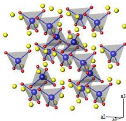
Figure 30 : Structure de la phase cristalline \text{Na}_2\text{MoO}_4 . Sphères bleues : cations \text{Mo}^{6+} ; Sphères jaunes : cations \text{Na}^+ ; Sphères rouges : anions \text{O}^{2-} . Dans cette figure, la taille des sphères n'est pas tracée en fonction de la taille réelle des ions [54].
