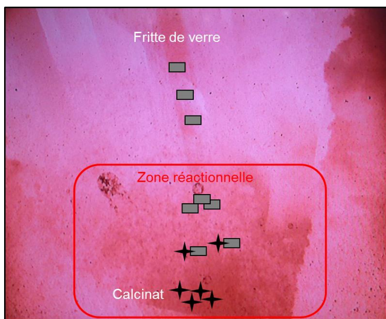
Figure 5 : Photographie prise lors d'un essai de vitrification sur l'installation prototype évolutif de vitrification (PEV) réalisé avec un débit d'alimentation en calcinat important (vue de haut).
