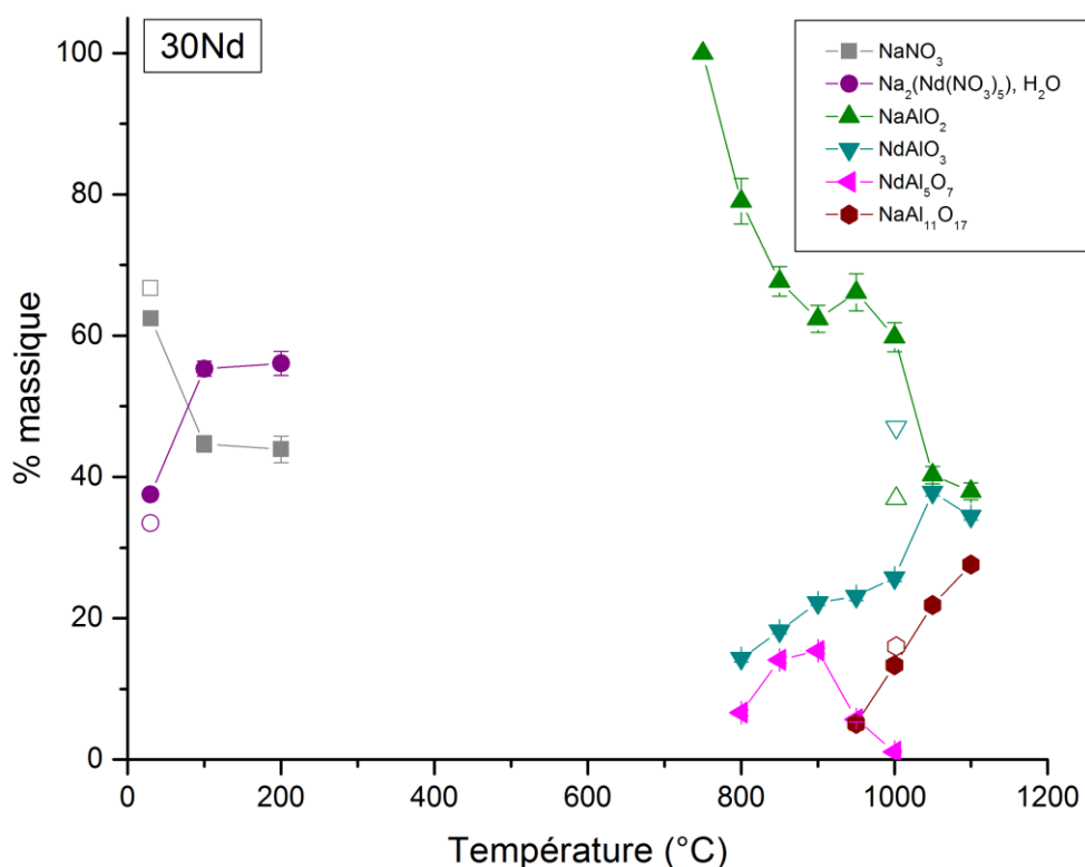
Figure 83 : Evolution des fractions cristallines déterminées par affinement Rietveld en fonction de la température du calcinat C-30Nd (normalisées sans tenir compte de la fraction amorphe). Les symboles évidés correspondent aux quantifications renormalisées sans amorphe ni \text{Al}(\text{OH})_3 obtenues par DRX ex-situ à la température ambiante et à 1000 °C.
