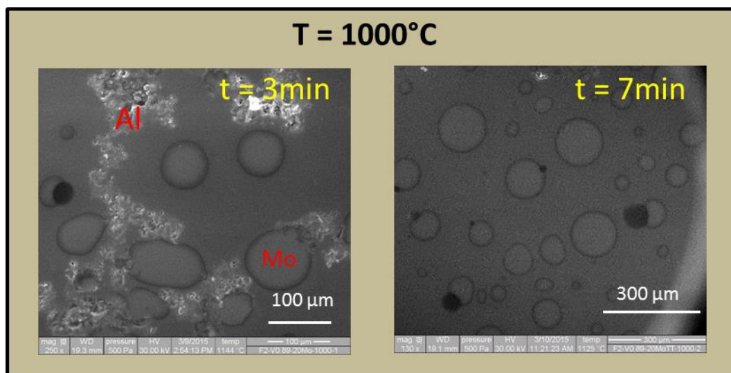
Figure 124 : Clichés du mélange C-20MoTT + F2 maintenu à 1000 °C trois minutes et sept minutes hors du MEBE.
