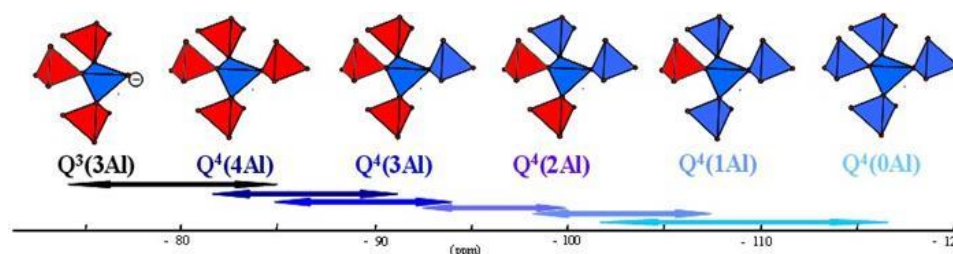
Figure 17 : Représentation des unités \text{Q}^4(m\text{Al}) et \text{Q}^3(m\text{Al}) : les tétraèdres de silicium sont en bleu par rapport aux tétraèdres d'aluminium en rouge.
