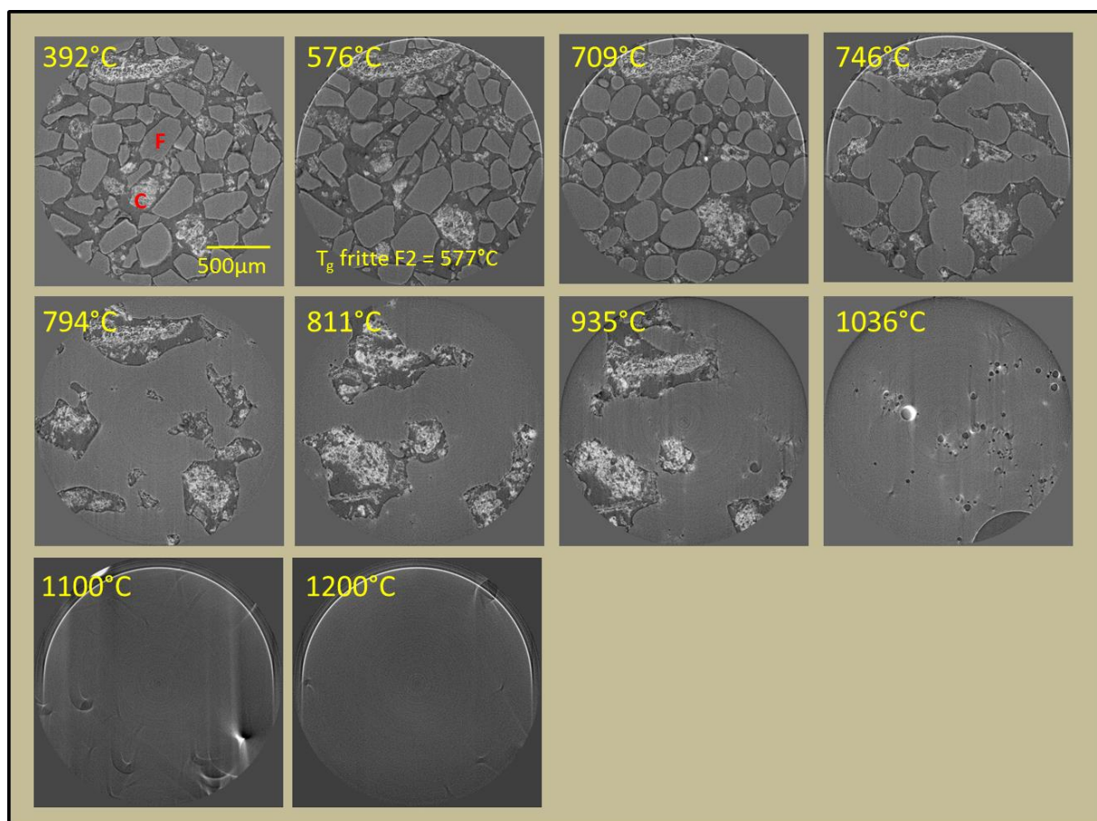
Figure 113 : Clichés d'une section du mélange C-20MoTT + F2 (F/V=0,90) acquis par microtomographie X in-situ en température (ESRF-ligne ID19). Les grains de calcinat sont notés (C) et ceux de fritte de verre sont notés (F).
