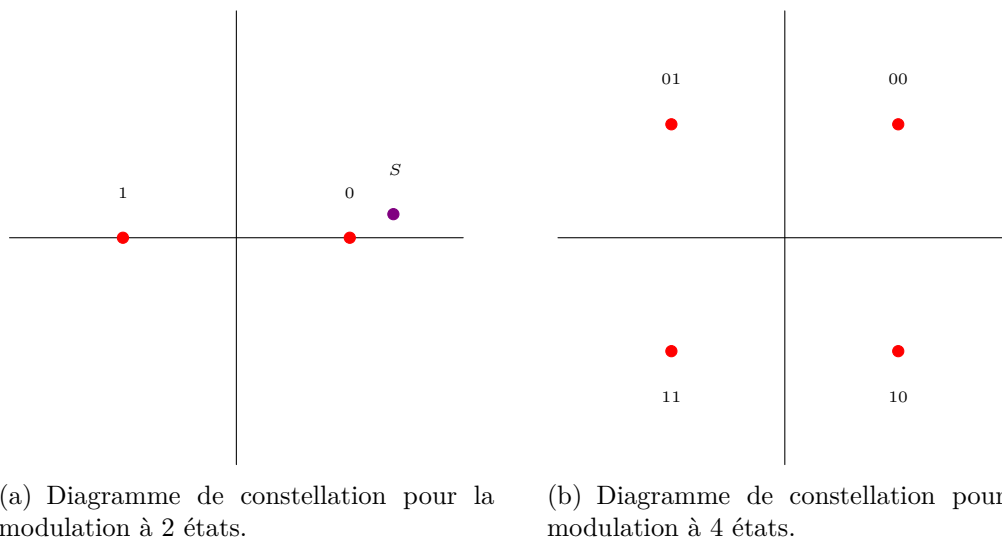
FIGURE 1.3 – Une représentation graphique des codages binaires est celle des diagrammes de constellation dans laquelle chaque point représente un symbole c_k . Les diagrammes de constellation théoriques des schémas de modulation numérique à 2 et à 4 états sont respectivement présentés sur les figures 1.3(a) et 1.3(b) (points rouges). Lors de la phase de réception d'un signal, les symboles sont examinés. Ces symboles peuvent avoir été altérés. Le récepteur estime alors le point de la constellation idéale le plus proche du symbole reçu. Un exemple est donné sur la figure 1.3(a) dans lequel un symbole S est reçu déformé. Dans ce cas, le récepteur choisira la valeur 0 lors du décodage du symbol.
