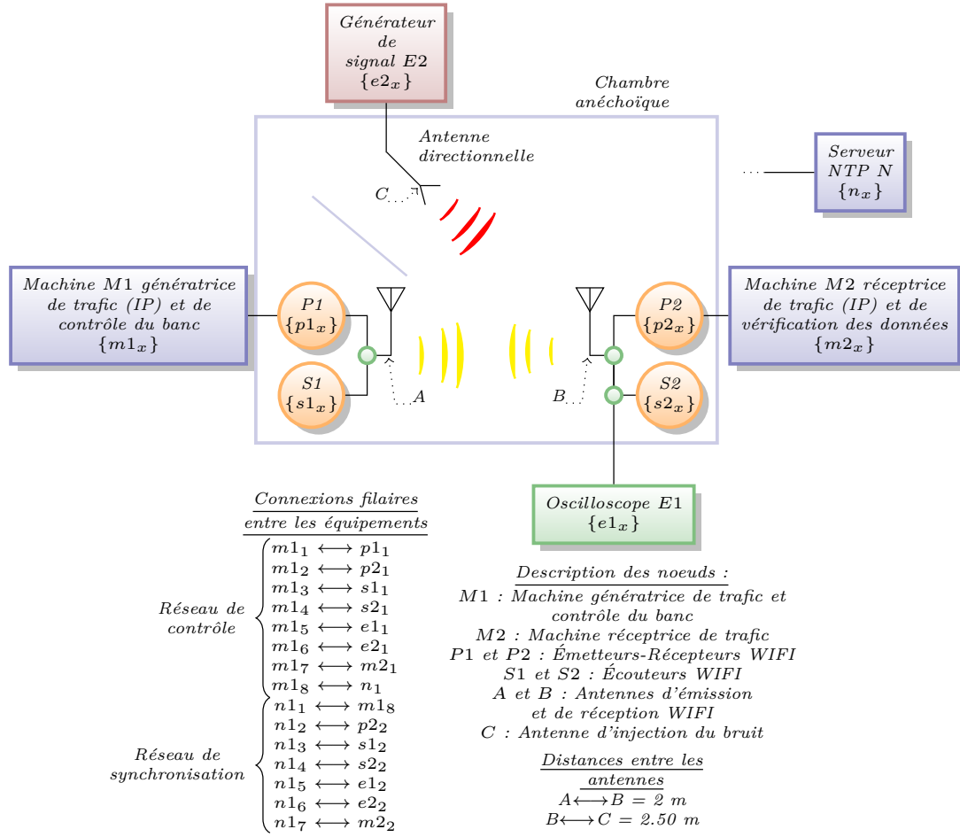
FIGURE 4.7 – Description complète du banc de test et des différents réseaux utilisés. La notation \{a_x\} correspond à l'ensemble des interfaces de l'équipement A . La notation a \longleftrightarrow b signifie qu'il existe une connexion entre l'interface a et l'interface b . Pour ne pas surcharger les boîtiers, le trafic est généré sur la machine M1 et réceptionné sur la machine M2 . Les boîtiers P1 et P2 sont donc paramétrés comme des ponts entre leur connexion filaire et leur connexion sans-fil. Les noeuds S1 et S2 sont les noeuds écouteurs facultatifs mis en place pour ne pas biaiser les mesures. L'ensemble des équipements est commandé par l'intermédiaire du réseau de contrôle et d'un logiciel situé sur la machine M1 .
