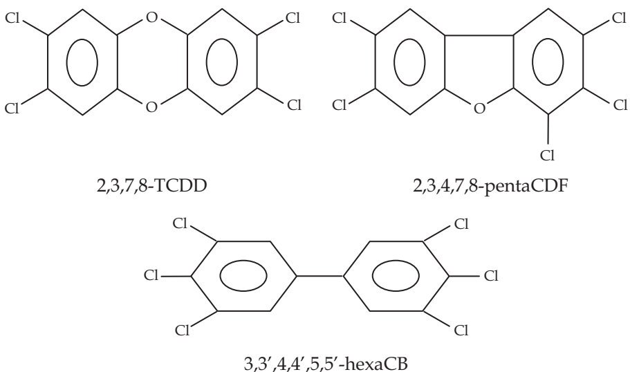
Figure 52.5 : Schéma des isomères de PCDD (2,3,7,8-TCDD ou « dioxine de Seveso »), de PCDF et de PCB les plus toxiques
