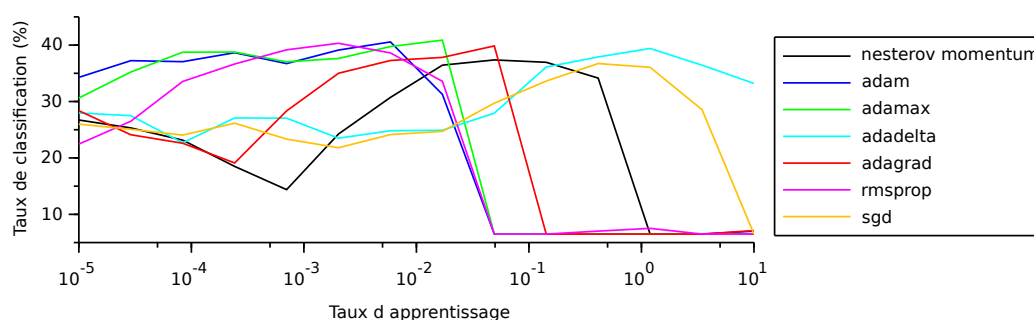
FIGURE 5.6 – Évolution du taux de classification en fonction du taux d'apprentissage et de la règle de mise à jour des poids
