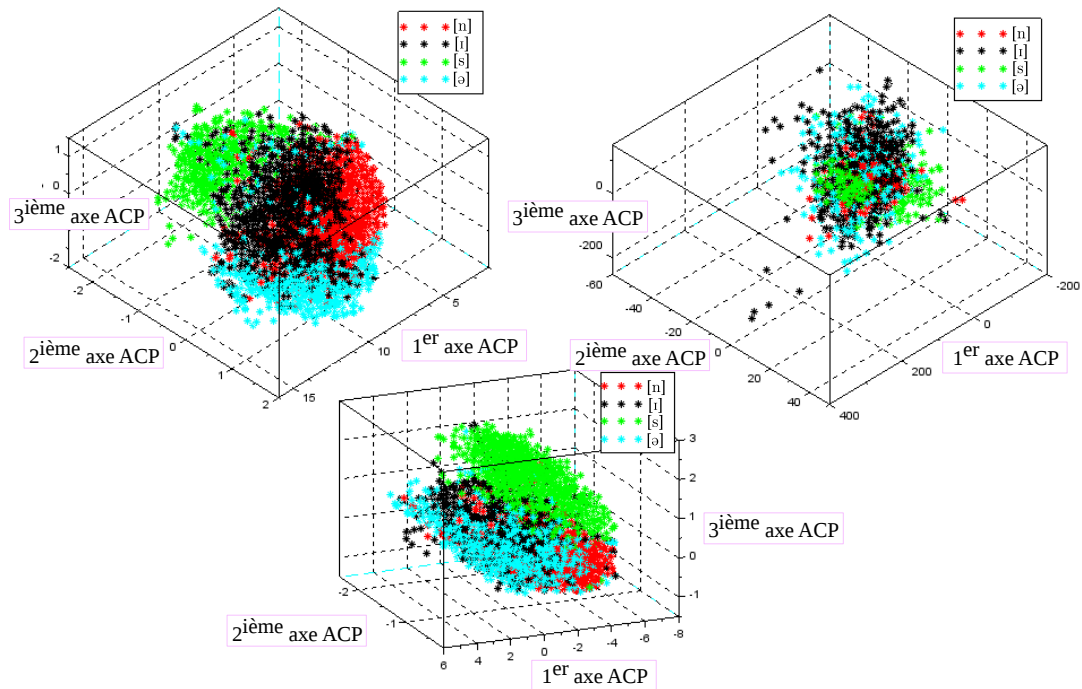
FIGURE 2.18 – Projection des réalisations du locuteur s01 des 4 phonèmes [n], [l], [s] et [ə] sur les axes formés par les MFCC (à gauche), MFCC centrée normés (au milieu) et les bancs de filtres (à droite)
