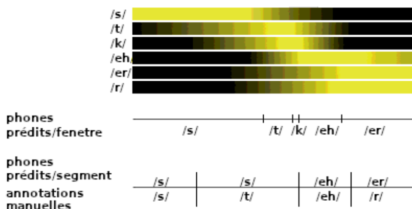
FIGURE 3.16 – Illustration de probabilités par trame (posterior-grammes) obtenues sur un segment et analyse des erreurs par fenêtre et par segment
