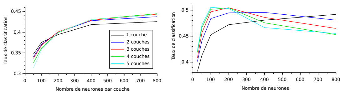
FIGURE 3.9 – Taux de classification obtenu sur BUCKEYE-DEV par un MLP en fonction du nombre de couches cachées et du nombre de neurones par couche, avec dropout (à gauche) ou sans (à droite)
