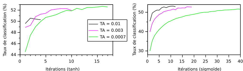
FIGURE 3.11 – Résultats selon le Taux d'Apprentissage (TA) pour la tangente hyperbolique (à gauche) et la fonction sigmoïde (à droite)
