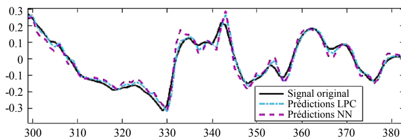
FIGURE 5.21 – Signal original et signaux reconstruits à l'aide de vrais coefficients LPC et ceux générés par notre réseau de neurones
