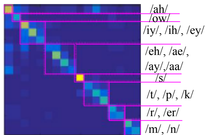
FIGURE 3.17 – Matrice de confusion des prédictions du réseau de neurones pour 17 phonèmes différents. Après regroupement des phonèmes affichant les erreurs d'attribution les plus élevées, 77% des exemples sont dans le bon groupe
