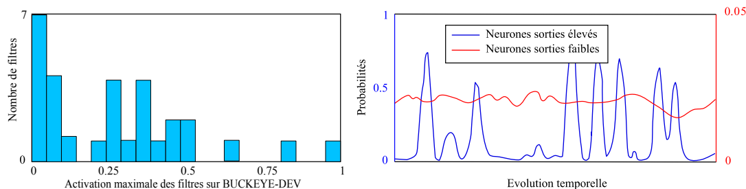
FIGURE 3.13 – Répartition des filtres selon leurs activations (à gauche) et résultats pour les filtres les plus faibles (à droite)
