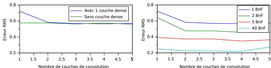
FIGURE 5.14 – Erreur RMS pour un réseau avec ou sans couche dense autour de la couche dense de Bottleneck (à gauche) et selon le nombre de couches de convolution (à droite)
