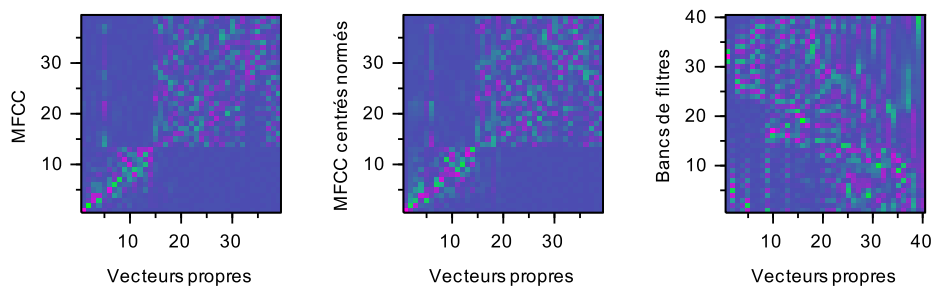
FIGURE 2.19 – Matrice des vecteurs propres correspondant à l'ACP réalisée sur les MFCC (à gauche) et les bancs de filtres (à droite)
