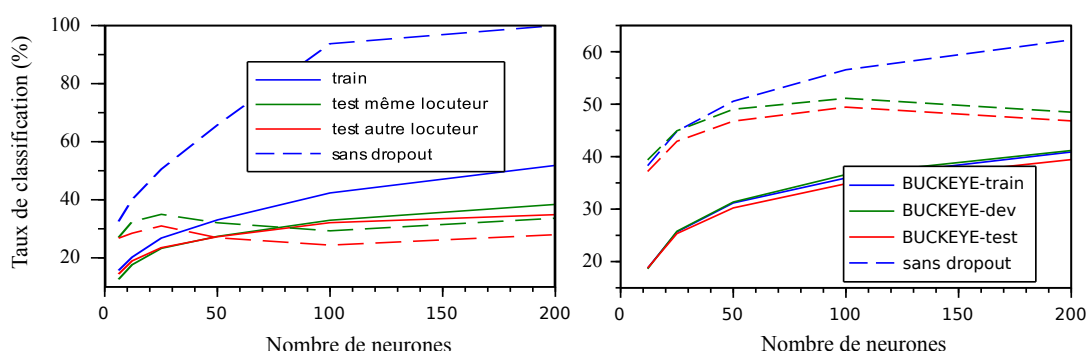
FIGURE 3.7 – Influence du dropout sur la robustesse à de nouvelles données d'un MLP pour la classification de phonèmes pour un unique locuteur dans l'ensemble d'apprentissage (à gauche) ou tout le corpus d'apprentissage (à droite)
