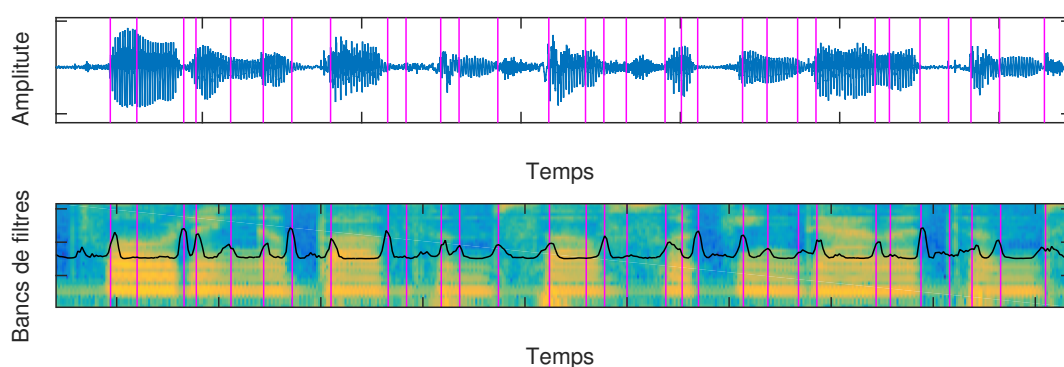
FIGURE 4.8 – Probabilités en sortie du CNN pour la segmentation sur BUCKEYE-TEST (en noir) superposé au spectrogramme ( en bas ) avec les vrais frontières phonétiques (en mauve). Le signal audio est donné dans le graphique du haut
