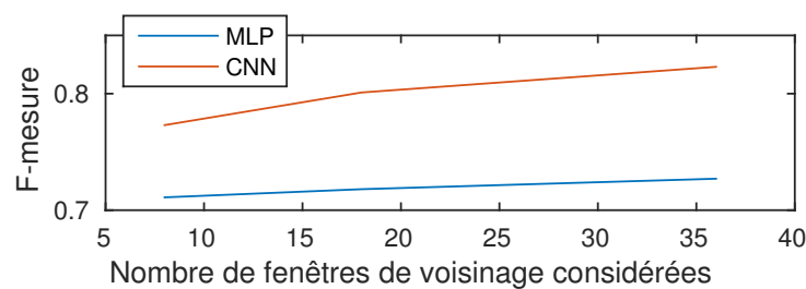
FIGURE 4.6 – Comparaison des F-mesures du MLP et du CNN selon le nombre de fenêtres de voisinage sur BUCKEYE-DEV
