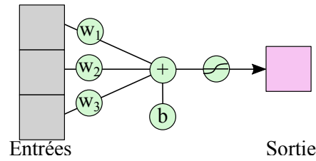
FIGURE 2.23 – Schéma d'un neurone. Une projection non linéaire avec biais ( b ) : les entrées (carrés gris) sont multipliées par les poids du neurone ( w_i ) puis sommées
