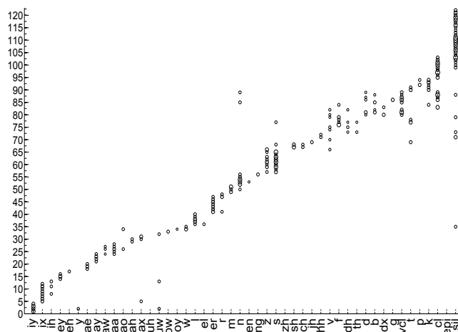
FIGURE 2.7 – Image issue de (C.-y. LEE et J. GLASS 2012) illustrant la pureté des groupes obtenus sous forme de matrice de confusion, avec seulement les paires groupes/phonèmes présentes plus de 200 fois pour plus de clarté
