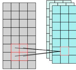
FIGURE 2.26 – Illustration de la sortie d’une couche de convolution de trois filtres de taille (2x2)
