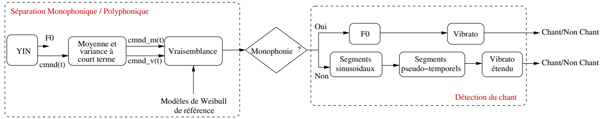
FIG. 4.5 – Schéma général du système de détection du chant.
