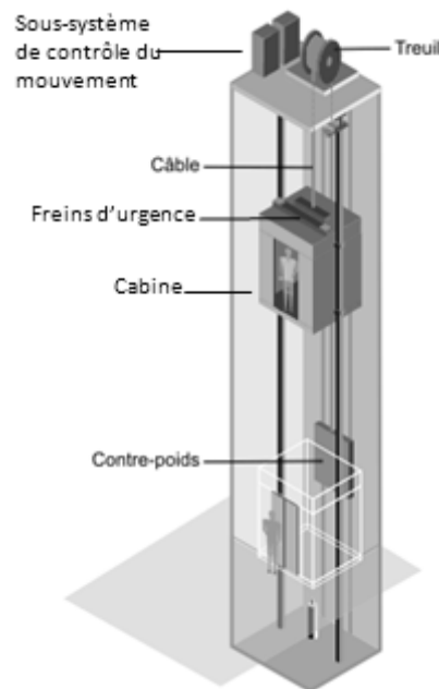
Figure III.16 : Système ascenseur
