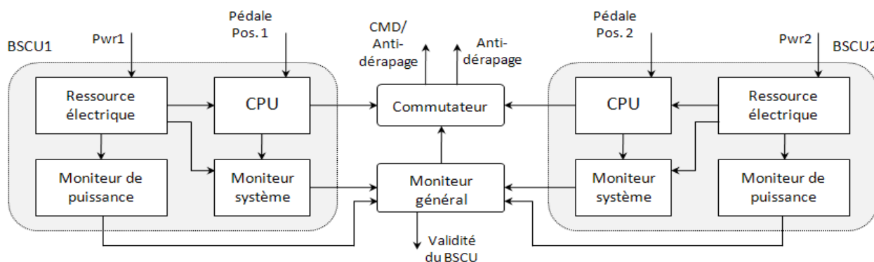
Figure V.3 : Système BSCU
