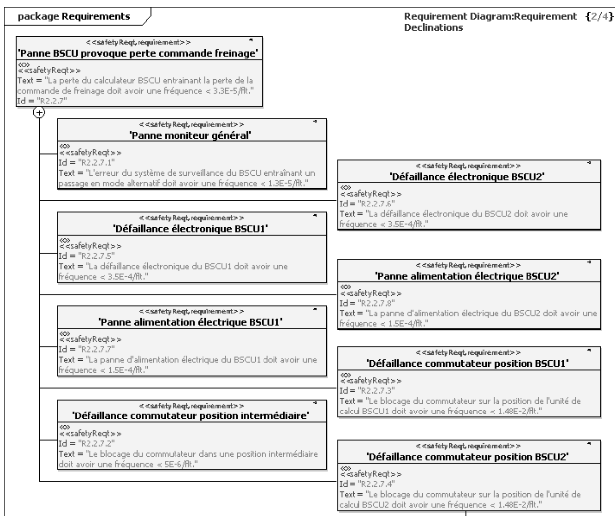
Figure B.4 : Calculateur BSCU – Diagramme de déclinaison des exigences (partie 1/2)
