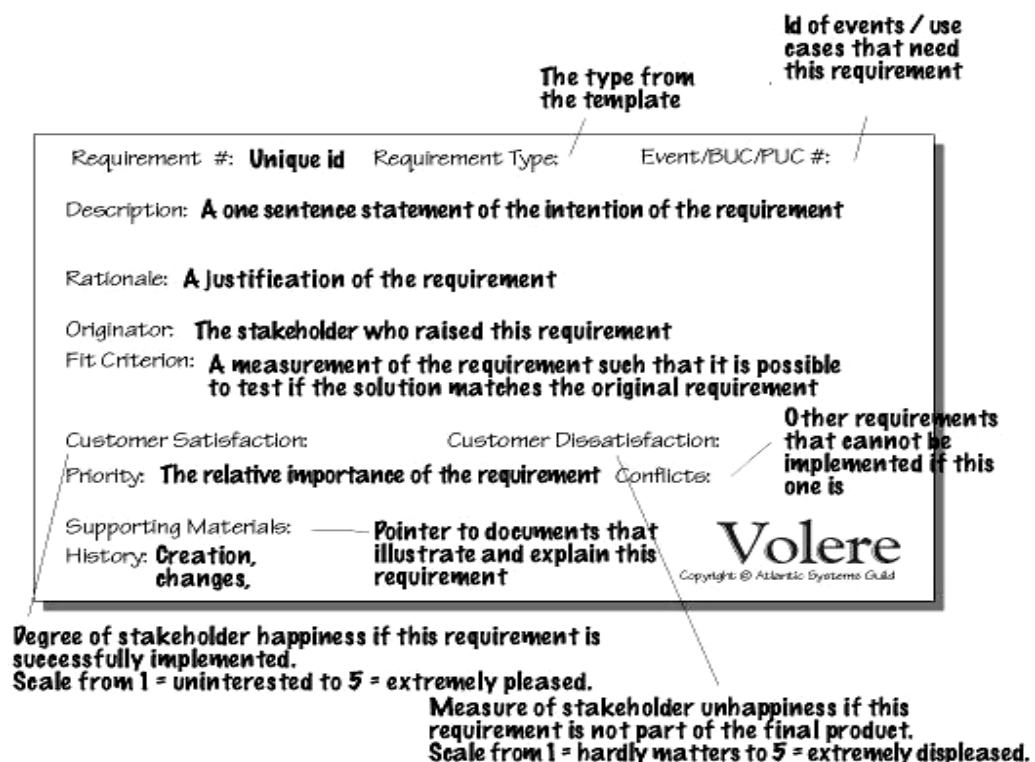
Figure IV.13 : SnowCard Volere
