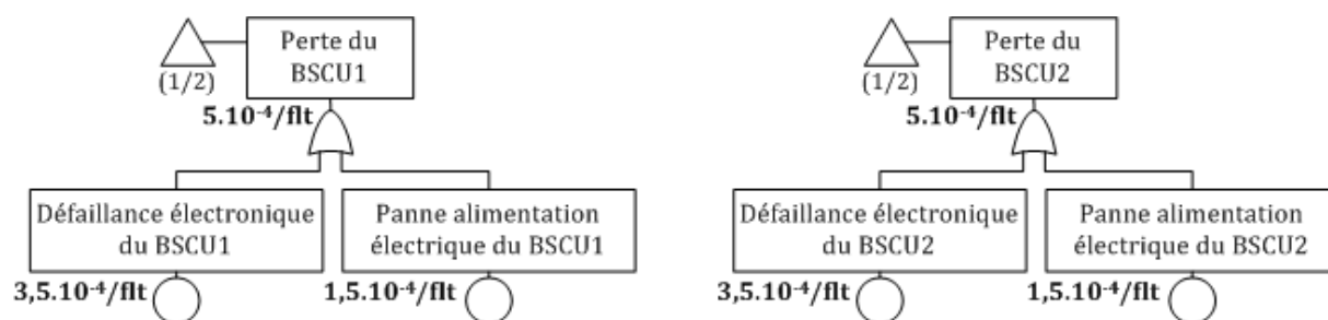
Figure V.11 : Arbre de défaillance de « une défaillance du BSCU provoque la perte de la commande de freinage » (2/2)
