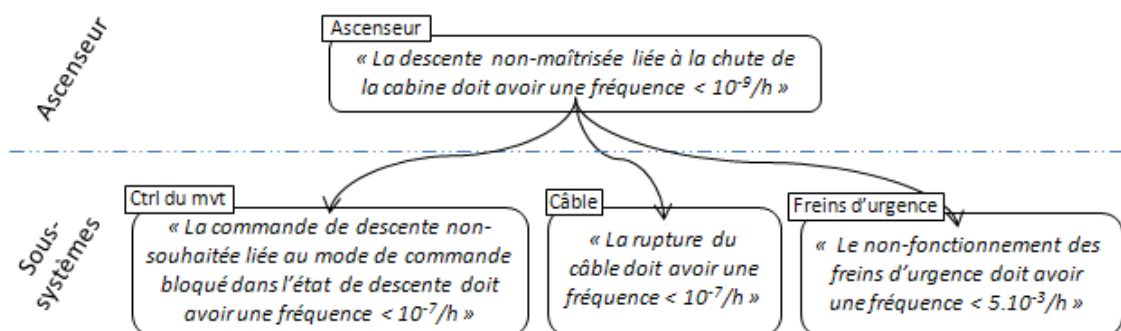
Figure III.20 : Synthèse de la déclinaison des exigences du système « ascenseur »
