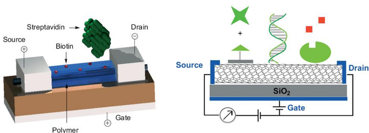
Figure 27 : Deux concepts de détecteur à base de NTC 322, 323, 320 .
