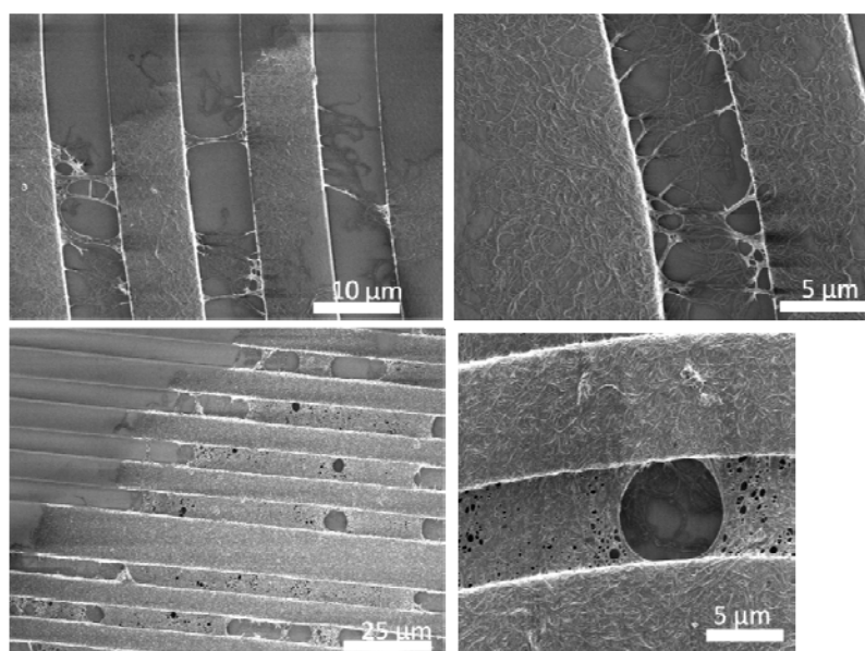
Figure 79 : Incubation d'un timbre de PDMS microstructuré avec des lignes de 10µm dans une suspension de NTC.
