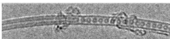
Figure 7 : Formation de la paroi interne d'un DWNT par coalescence d'endofullerènes (visible dans le SWNT sur la droite de l'image) 66 .
