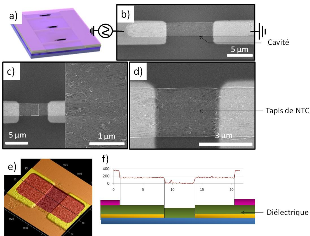
Figure 134 : Résultats obtenus grâce au protocole de DEP à électrodes enterrées et assemblage capillaire optimisé. a) Schéma de principe. b-d) Images MEB des cavités de résine remplies de NTC. e) Image AFM d'une de ces cavités. f) Schéma de la tranche et mesure AFM.
