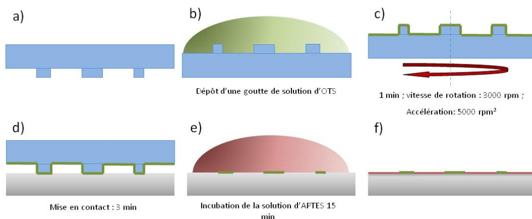
Figure 97 : Procédé de bifonctionnalisation par OTS et APTES d'un substrat. a) Préparation du timbre (voir chapitre 3). b) Encreage d'OTS sur le timbre. c) Séchage à la tournette puis par flux d'azote. d) Mise en contact du tampon avec le substrat. e) Incubation d'APTES. f) Dépôt final microstructuré d'OTS et d'APTES.
