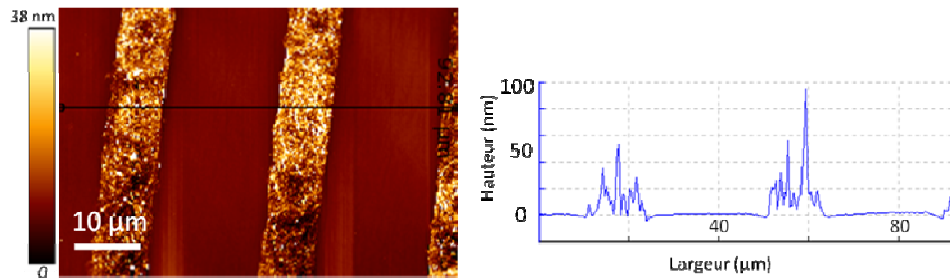
Figure 91 : Image AFM de motifs de NTC obtenus par impression microcontact et profil correspondant.
