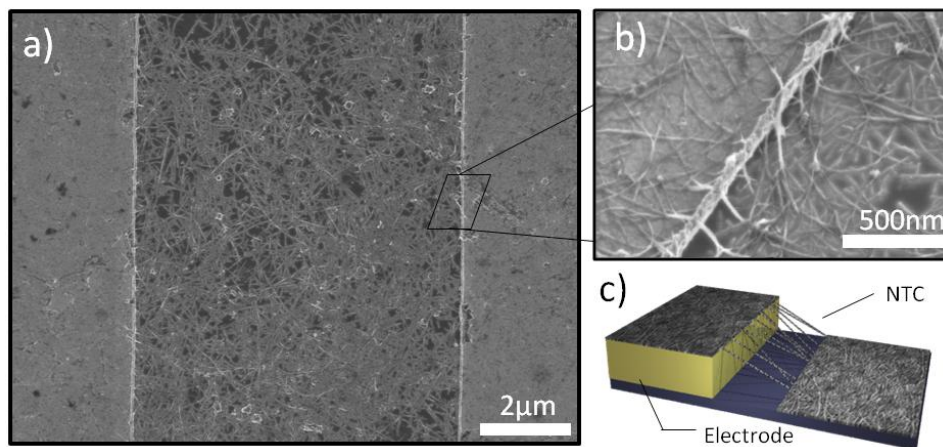
Figure 75 : Image MEB des contacts entre les tapis de NTC pulvérisés et les électrodes. a) Vue d'ensemble d'un gap entre 2 électrodes. b) Zoom et vue avec un angle de 40^\circ sur les contacts. c) Schéma d'interprétation.
