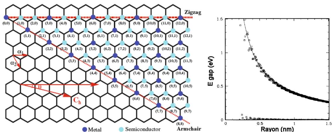
Figure 15 : A gauche, représentation graphique du comportement électrique d'un NTC en fonction de sa structure 9, 113 . A droite, taille du gap d'énergie théorique en fonction du diamètre d'un SWNT 110 .
