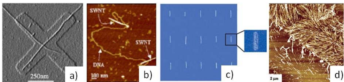
Figure 37 : a) NTC sélectivement déposés sur un motif en X d'APTES 406 b) Brin d'ADN accrochant sélectivement des NTC 404 . c) Réseau de NTC adsorbé sur des motifs d'APTES 405 . d) Les NTC sont sélectivement dirigés par l'interaction entre la suspension et des SAM, hydrophiles et hydrophobes 402 .
