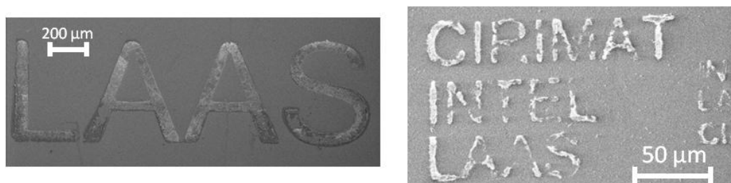
Figure 90 : Tapis de NTC microstructurés par \mu\text{CP} de motifs isolés.
