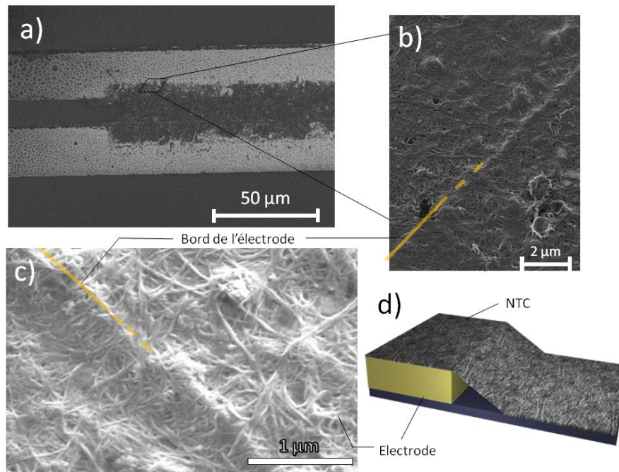
Figure 92 : a) Image MEB d'une connexion en NTC obtenue par \mu CP et encrage par pulvérisation. b) et c) Zoom sur le bord de l'électrode. d) Schéma d'interprétation.
