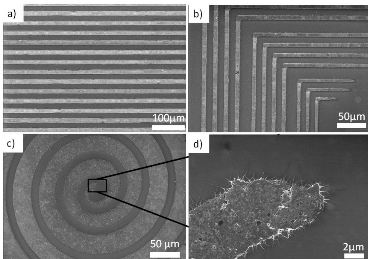
Figure 89 : Résultats obtenus pour l'impression par microcontact de différentes structures. a) Lignes de 10μm. b) Lignes avec angles droit de 5μm. c) Motif en spirale de 25μm à 2μm. d) Zoom sur le bout de la spirale.
