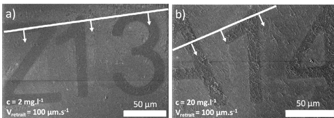
Figure 101 : Images MEB de deux expériences de trempage-retrait sur motifs chimiques pour deux concentrations différentes de NTC dans la NMP à 100\mu\text{m.s}^{-1} après 30s d'immersion. a) 2\text{mg.l}^{-1} b) 20\text{mg.l}^{-1} . La direction de balayage du solvant est représentée.
