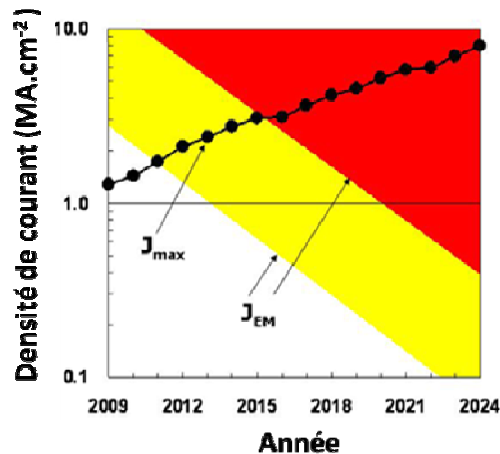
Figure 30 : Evolution de la densité maximum de courant ( J_{max} ) requise pour les années futures et de la densité de courant maximales que l'on peut atteindre avec les technologies actuelles limitées par l'électromigration ( J_{em} ) (Source ; rapport de l'ITRS)
