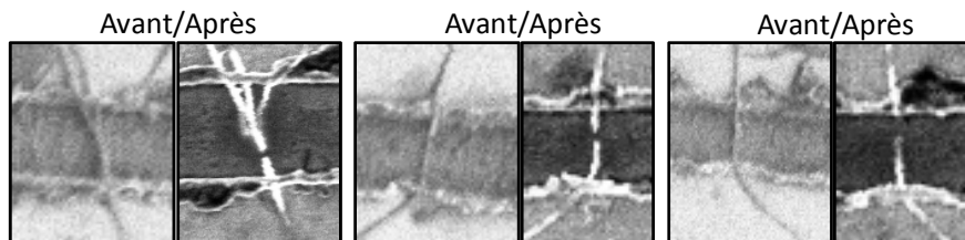
Figure 51: Observation de NTC entre 2 électrodes (gap 0.5μm) avant et après avoir été testés électriquement (premier cas faisceau, second cas, rupture de la connexion au centre et dernier cas, destruction au contact NTC/métal).
