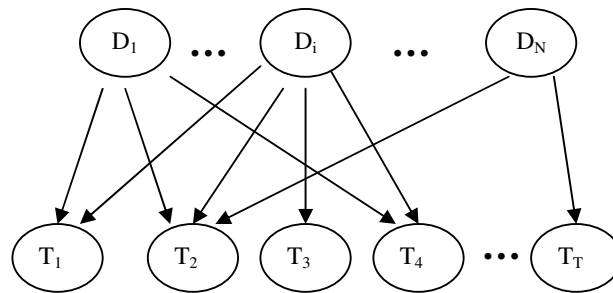
Figure 3.11 : Architecture générale du modèle possibiliste quantitatif
