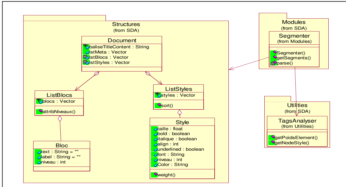
Figure 5.19 : Diagramme de classes du processus de segmentation
