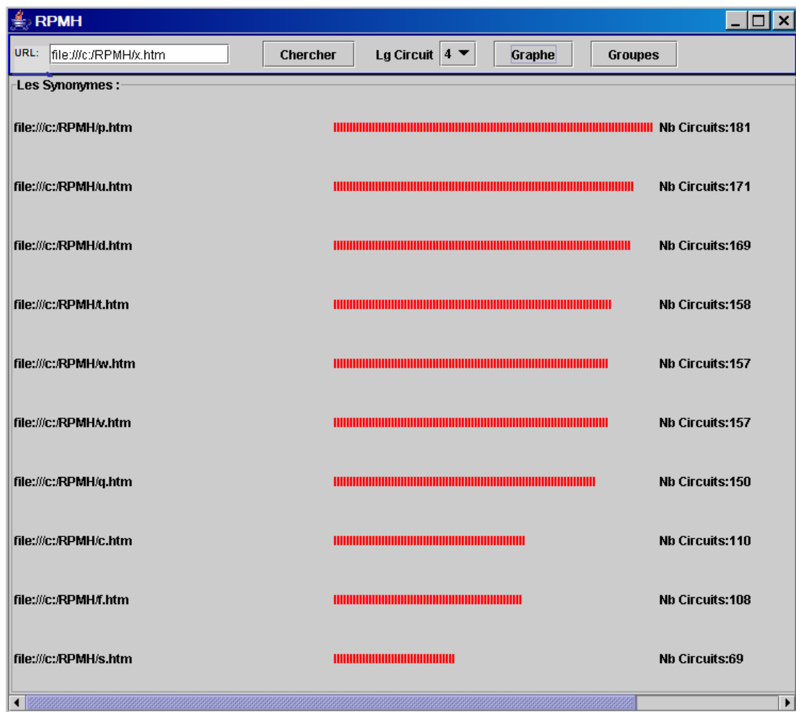
Figure 6.10 : Interface de calcul du nombre de circuits sélectionnés entre les pages Web
