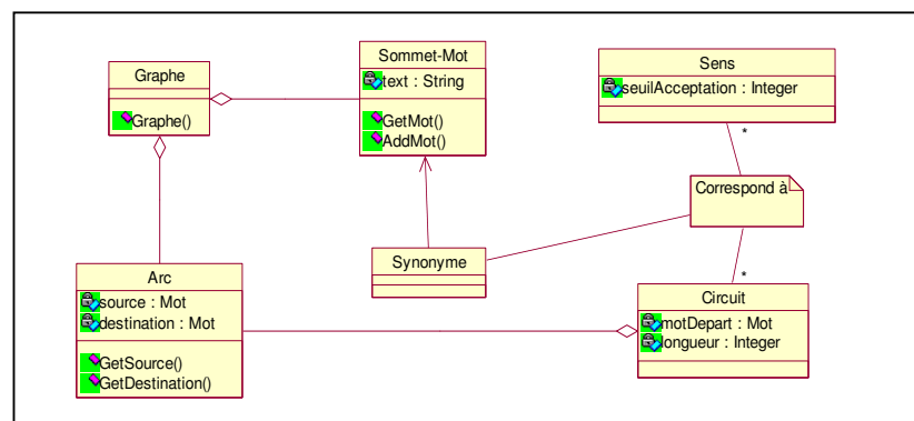
Figure 5.12: Diagramme de classes de la construction du RPMH de dictionnaire
