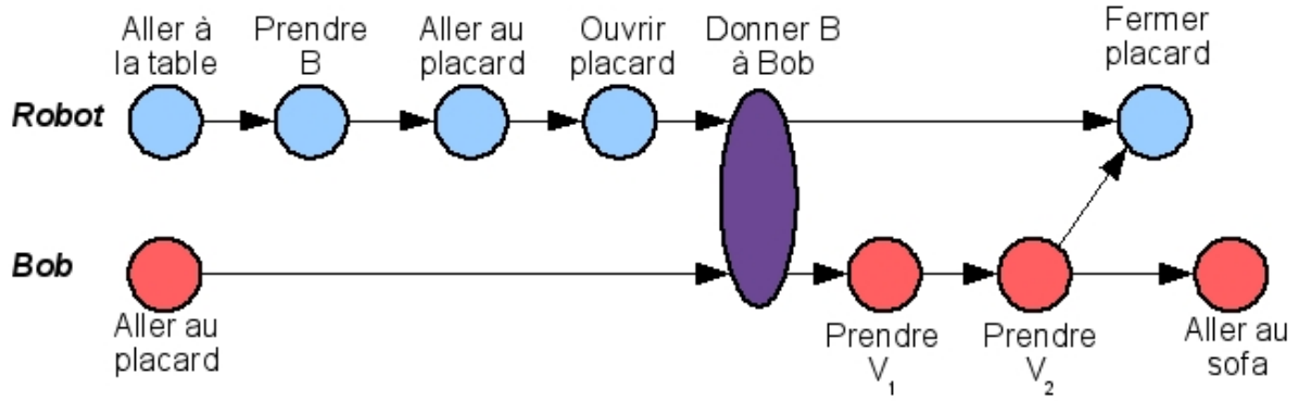
FIG. 3.7 – Exemple de plan solution : plan contenant des temps morts.
