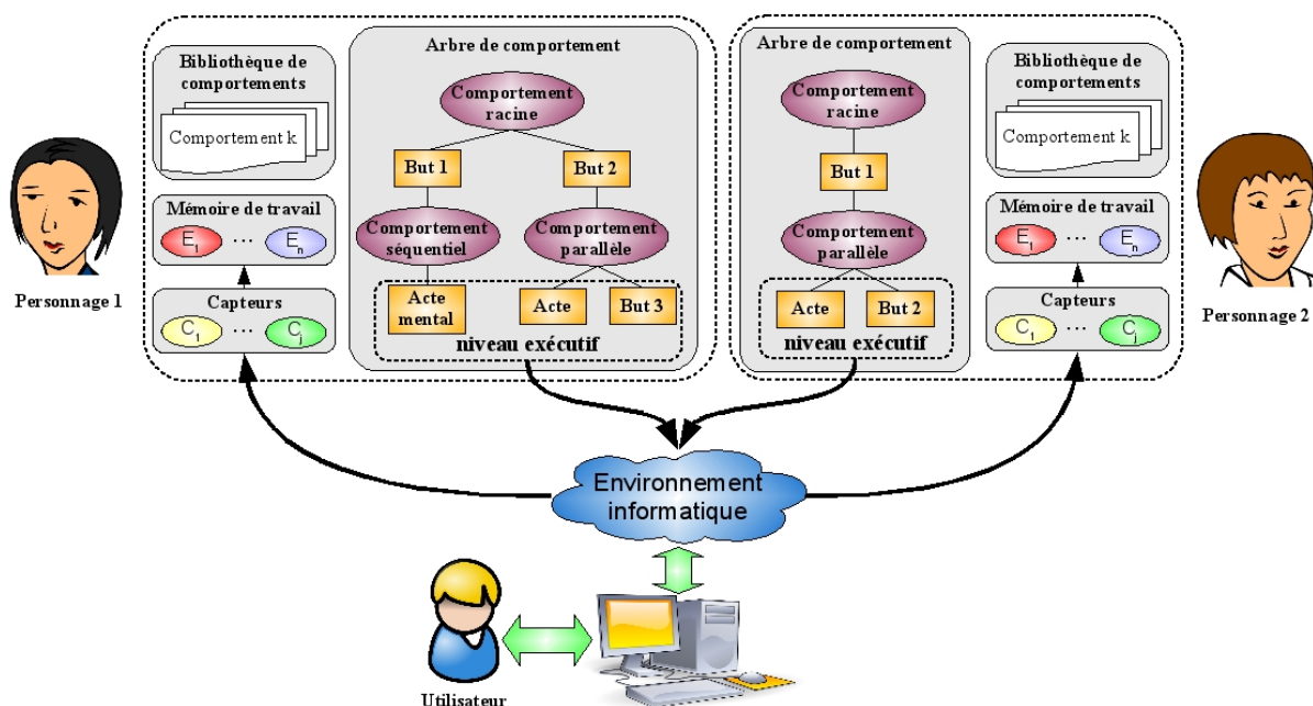
FIG. 1.7 – Structure de fonctionnement du langage ABL.
