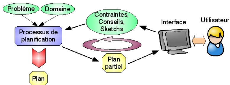
FIG. 1.10 – Planificateur à initiative mixte. Le planificateur prend en entrée un problème et un domaine. Pendant le processus de planification l'utilisateur peut influencer les choix du planificateur en imposant des contraintes ou en choisissant les branches de l'espace de recherche à explorer.
