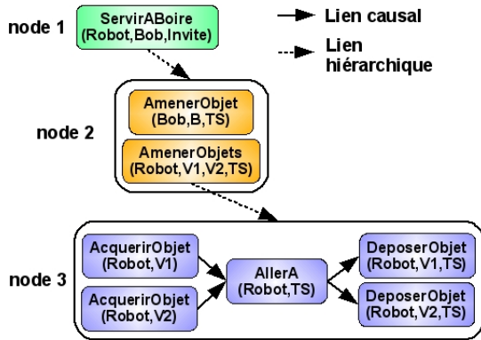
FIG. 4.17 – Problème HATP pour la tâche ServirABoire(Robot, Bob, Invite) avec contraintes du partenaire humain du robot.
