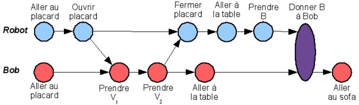
FIG. 3.8 – Exemple de plan solution : plan contenant des liens croisés.
