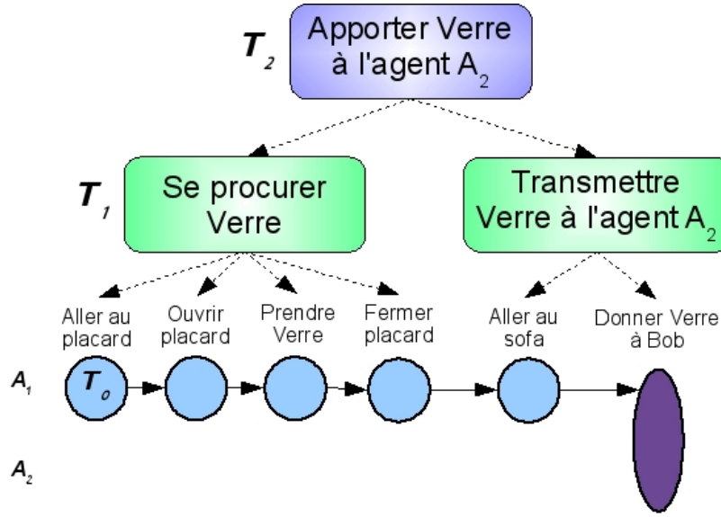
FIG. 3.9 – Exemple de graphe d'intentions.
