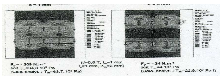
Figure III-13 : Simulation numérique en deux dimensions de la structure équipée de culasses
