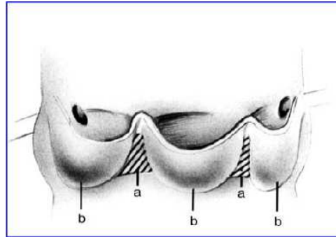
Figure III-3 : Triangles sous-commissuraux (a) et Sigmoïdes aortiques (b) (64)
