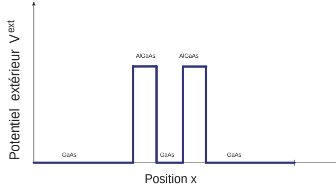
Figure 3: Double barrière de potentiel dans une diode à effet tunnel résonnant.
