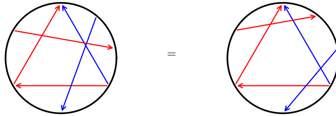
FIGURE A.1 – Exemple d'un Slide move
