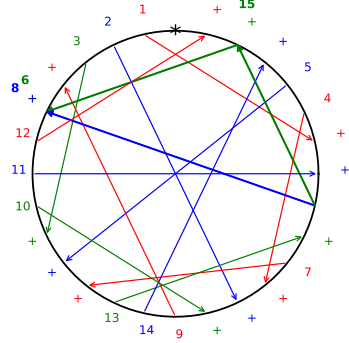
FIGURE 2.8 – Les 12 diagrammes de Gauss à point triple qui interviennent dans rot(S_{exemple}) (fin)
