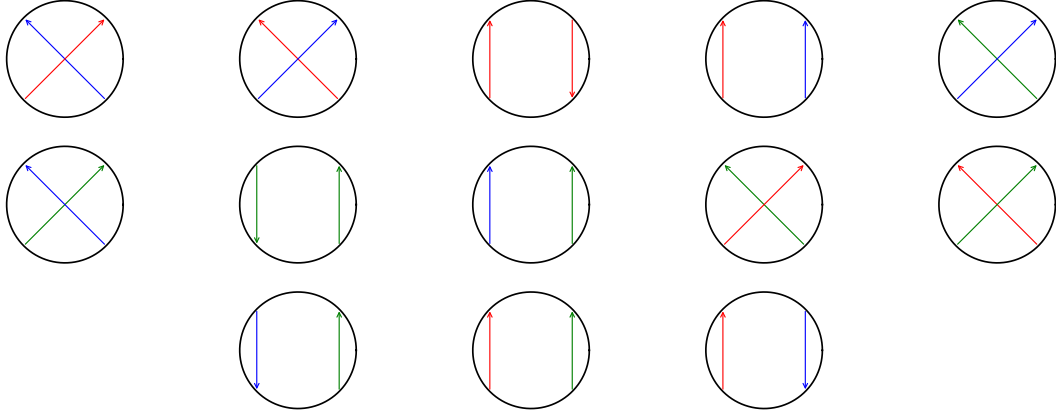
FIGURE 3.7 – Dans le sens de la lecture : C_{(2,1)}^c , C_{(1,2)}^c , C_{(1,1)}^o , C_{(1,2)}^p , C_{(3,2)}^c , C_{(2,3)}^c , C_{(3,3)}^o , C_{(2,3)}^p , C_{(3,1)}^c , C_{(1,3)}^c , C_{(2,3)}^o , C_{(1,3)}^p , C_{(1,2)}^o
