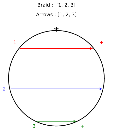
FIGURE 3.10 – Diagramme de Gauss pour la 4-tresse [1, 2, 3]
