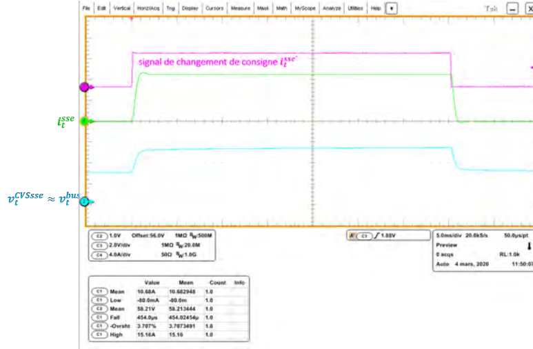
FIGURE 12 – Capture d'écran de l'oscilloscope lors du test permettant d'identifier R_{bus} et C_{bus} pour la BdT du bus
