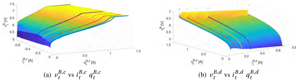
FIGURE III.22 – Interpolation et identification des paramètres de la fonction v_t^B = f(i_t^B, q_t^B) pour le modèle IVQ
