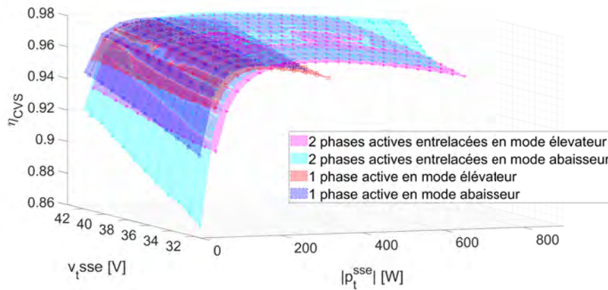
FIGURE 1 – Mesures du rendement de l'ISBC et interpolation linéaire, en mode abaisseur ( buck ) et élévateur ( boost ) avec une phase active et deux phases entrelacées actives
