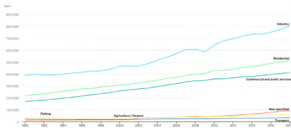
FIGURE I.4 – Consommation d'électricité finale par secteur dans le monde exprimée en ktoe ( kilo tonnes of oil equivalent ) [15]
