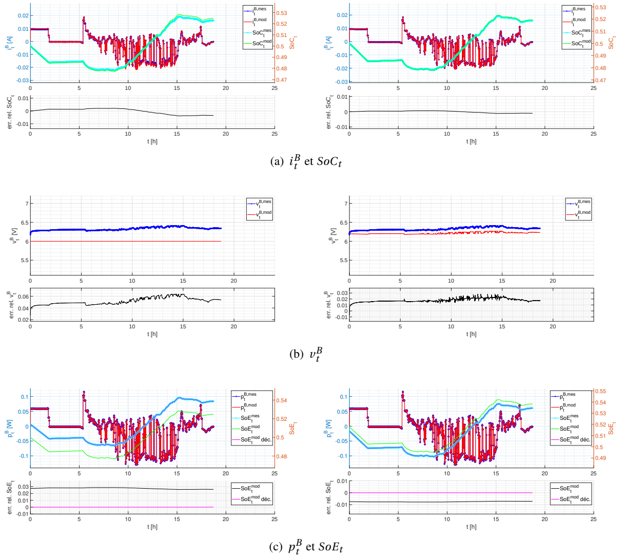
FIGURE 1 – Comparaison des mesures et des modèles PE (à gauche) et OCVR (à droite) pour la VRLAB BAT#3 et le profil de test n°1
