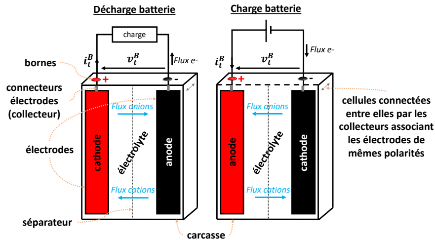
FIGURE III.5 – Schéma de principe du fonctionnement d'une batterie constitué d'une ou plusieurs cellules électrochimiques identiques
