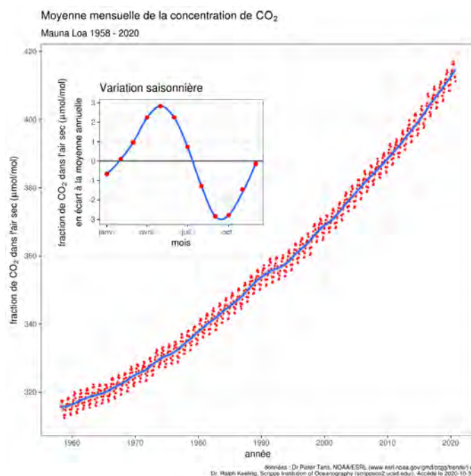
FIGURE I.5 – Évolution de la concentration du \text{CO}_2 dans l'atmosphère terrestre à l'observatoire de Mauna Loa depuis 1958 ou "courbe de Keeling" [21]
