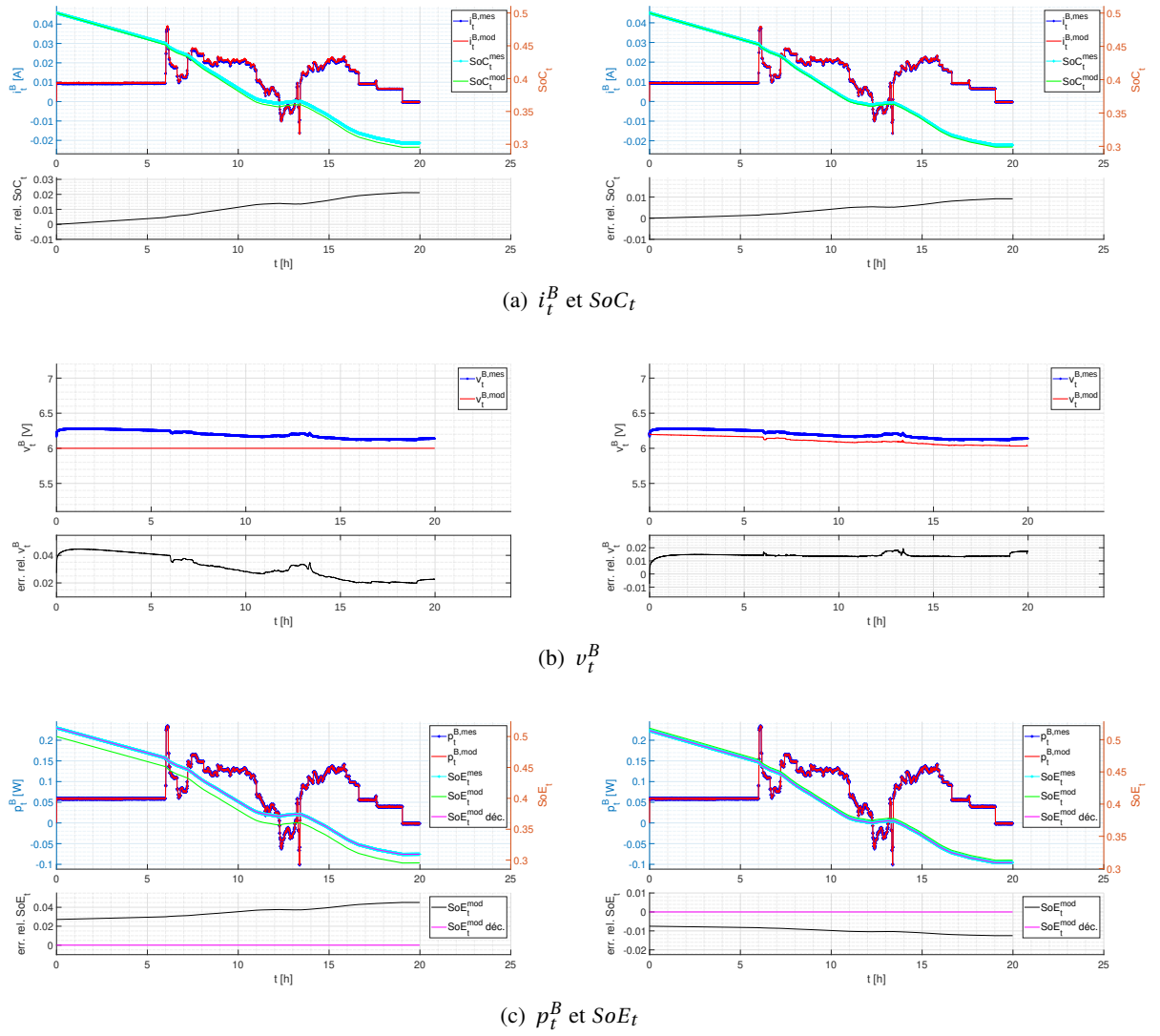
FIGURE 5 – Comparaison des mesures et des modèles PE (à gauche) et OCVR (à droite) pour la VRLAB BAT#3 et le profil de test n°5
