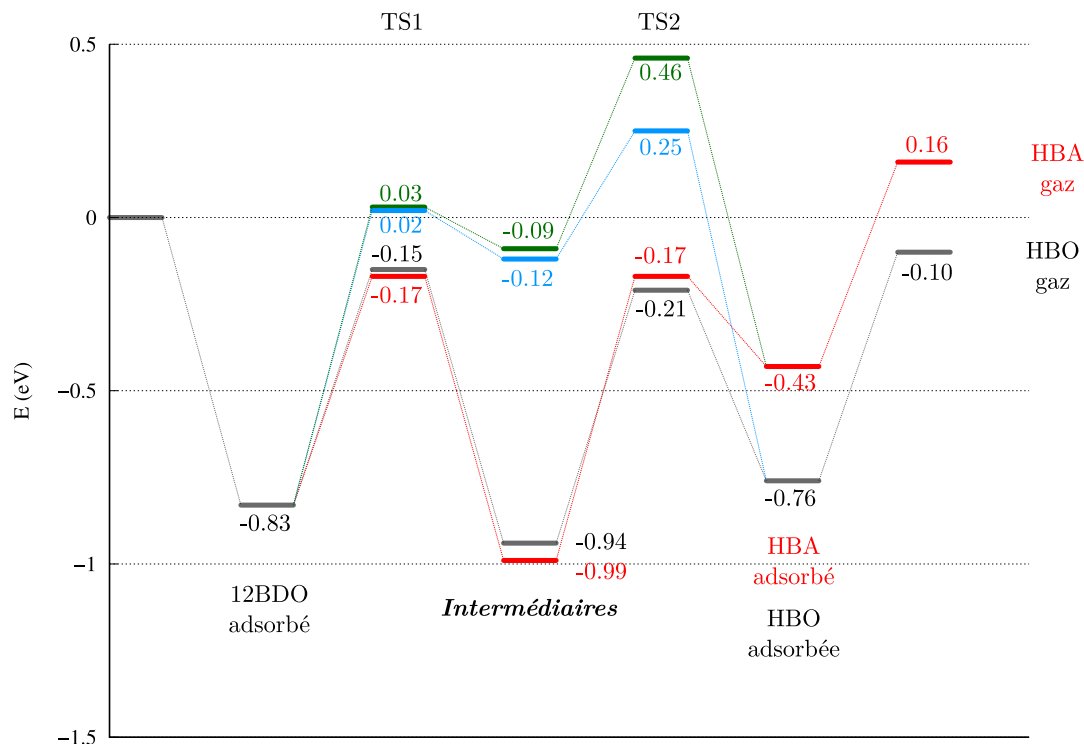
FIGURE 3.17 – Réactions de surface du 12BDO vers HBO ou HBA C-H_{\alpha} secondaire puis O-H secondaire en gris, C-H_{\alpha} primaire puis O-H primaire en rouge, O-H secondaire puis C-H_{\alpha} secondaire en bleu, O-H primaire puis C-H_{\alpha} primaire en vert
