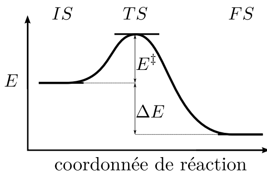
FIGURE 2.13 – Energie de réaction d'un réactif IS vers un produit FS par un état de transition TS
