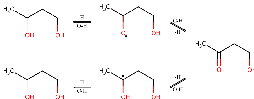
FIGURE 3.23 – 13BDO vers 4HBO
