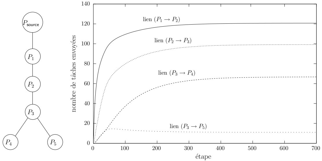
FIG. 6.5 – Simulation de l'algorithme de «multi-commodity flow» adapté au problème d'ordonnancement, sur une petite plate-forme.
