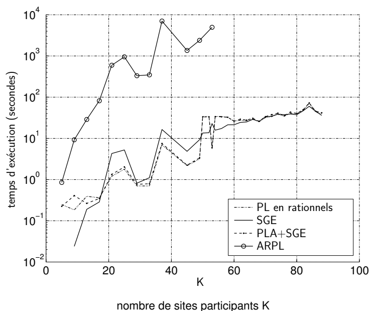
FIG. 7.7 – Temps d'exécution des heuristiques
