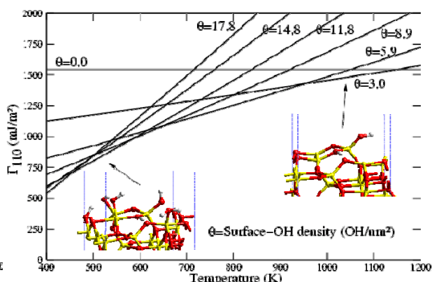
Figure 7 - Énergie de surface de l'alumine-γ (110) pour différents taux de recouvrement en hydroxyles \theta en fonction de la température pour une pression en eau de 1bar [30] (Hydrogène en blanc, aluminium en jaune et oxygène en rouge)
