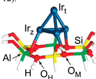
Figure 12 - Modèle d'agrégat supporté sur zéolite réalisé par l'équipe de Röscher [41,42]
