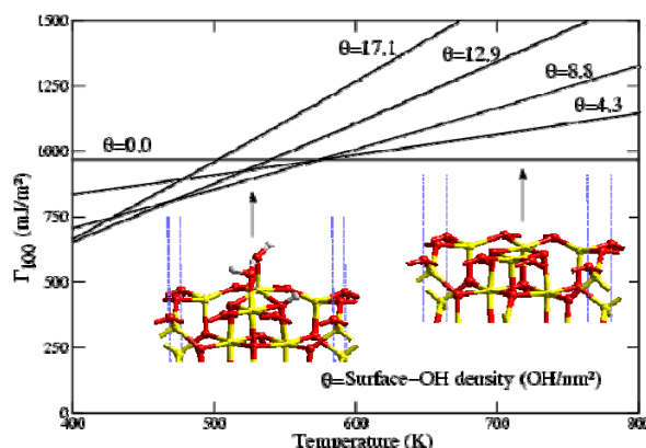
Figure 6 - Énergie de surface de l'alumine-γ (100) pour différents taux de recouvrement en hydroxyles \theta en fonction de la température pour une pression en eau de 1bar [30] (Hydrogène en blanc, aluminium en jaune et oxygène en rouge)
