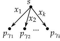
FIGURE 3.6 – Cas de base pour représenter un circuit asymétrique par un programme à branchements.
