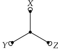
FIGURE 5.1 – Graphe représentant le polynôme XY + YZ + XZ .
