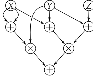
FIGURE 1.2 – Le polynôme 2XY + (X + Y)(Y + Z) représenté par un circuit arithmétique.
