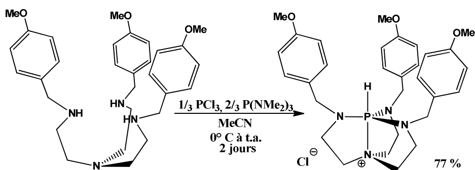
Schéma II. 20 : Conditions expérimentales de l'obtention de l'azaphosphatrane modèle
