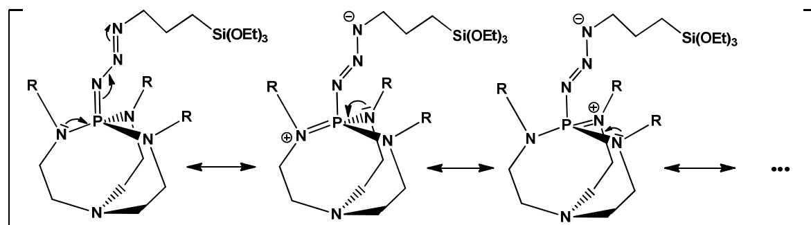
Figure III. 5 : Formes mésomères des azidoproazaphosphatranes
