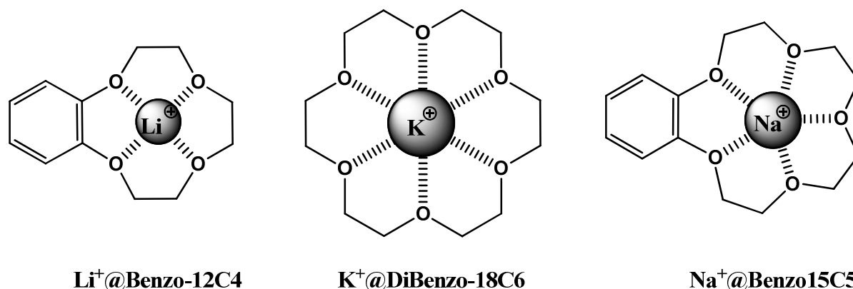
Figure II. 3 : Exemples d'éthers-couronnes synthétisés par Pedersen sous forme de complexes métalliques
