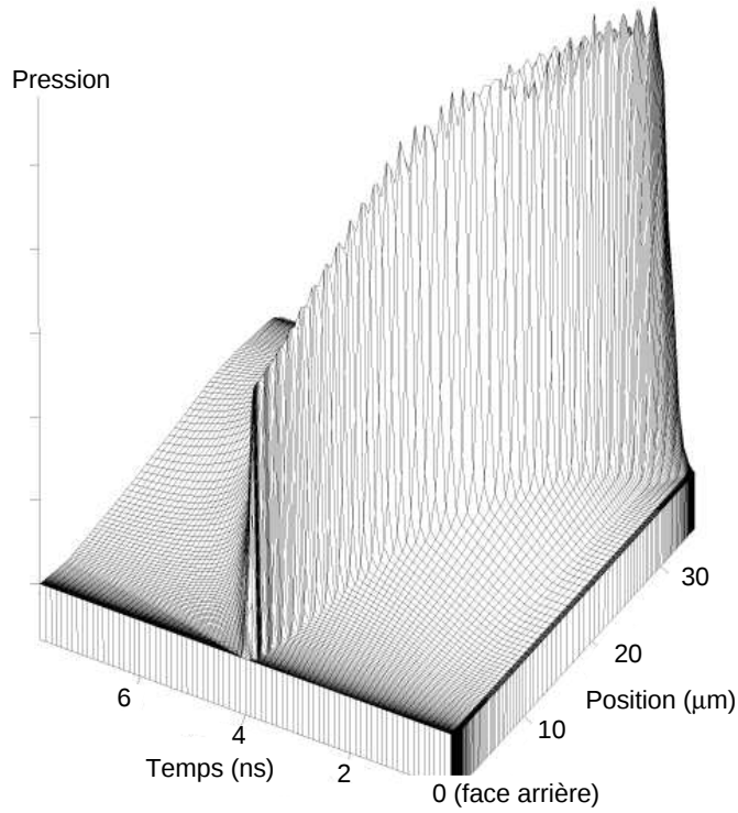
FIG. 3.25 – Simulation hydrodynamique du choc dû au piédestal ASE du laser (borne supérieure : 5 \times 10^{12} \text{Wcm}^{-2} ) pour une cible d'aluminium de 35 \mu\text{m} . La pression est tracée en fonction du temps et de la position dans la cible.
