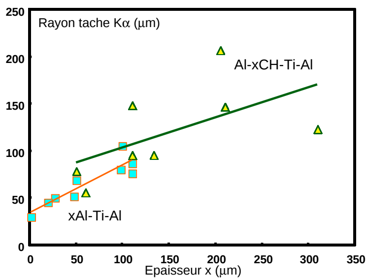
FIG. 4.26 – Rayon de la tache d'émission K\alpha en fonction de l'épaisseur de la couche de propagation de plastique, (cibles du type Al-CH-Ti-Al), ou d'aluminium (cibles du type Al-Ti-Al).
