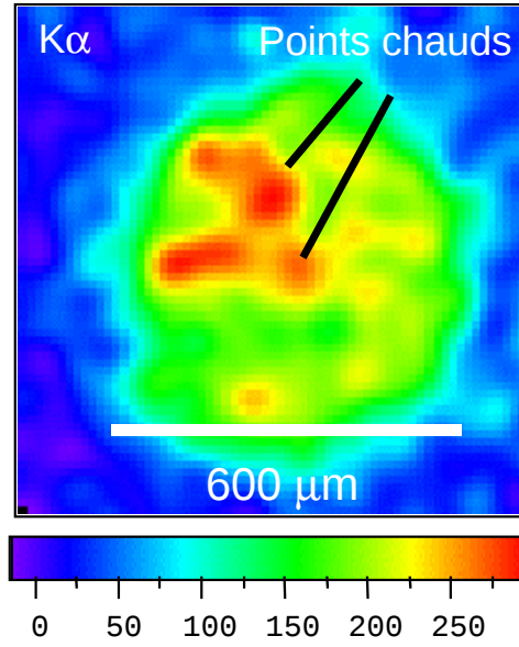
FIG. 4.31 – Image K\alpha d'une cible Al 11\mu\text{m} -CH 300\mu\text{m} -Cu 25\mu\text{m} -Al 16\mu\text{m} . Plusieurs points chauds sont visibles, témoignant d'une filamentation du faisceau d'électrons rapides traversant la couche fluorescente.
