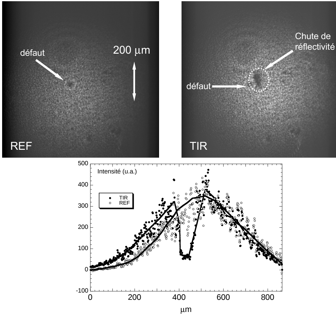
FIG. 3.12 – Images instantanées de la réflectivité de la face arrière d’une cible d’aluminium de 17\mu\text{m} d’épaisseur. A gauche, le tir de référence ; à droite le tir d’interaction ( 0.8J , 7.4 \times 10^{17} \text{Wcm}^{-2} ). L’image a été prise 25\text{ps} après l’interaction. Le chauffage est indiqué par une baisse de réflectivité (tache sombre). Un profil vertical passant par le centre de la tache est comparé avec le profil de référence correspondant.
