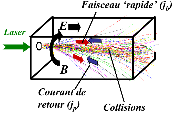
FIG. 2.6 – Schéma des effets des champs électriques et magnétiques sur la propagation du faisceau d'électrons rapides.
