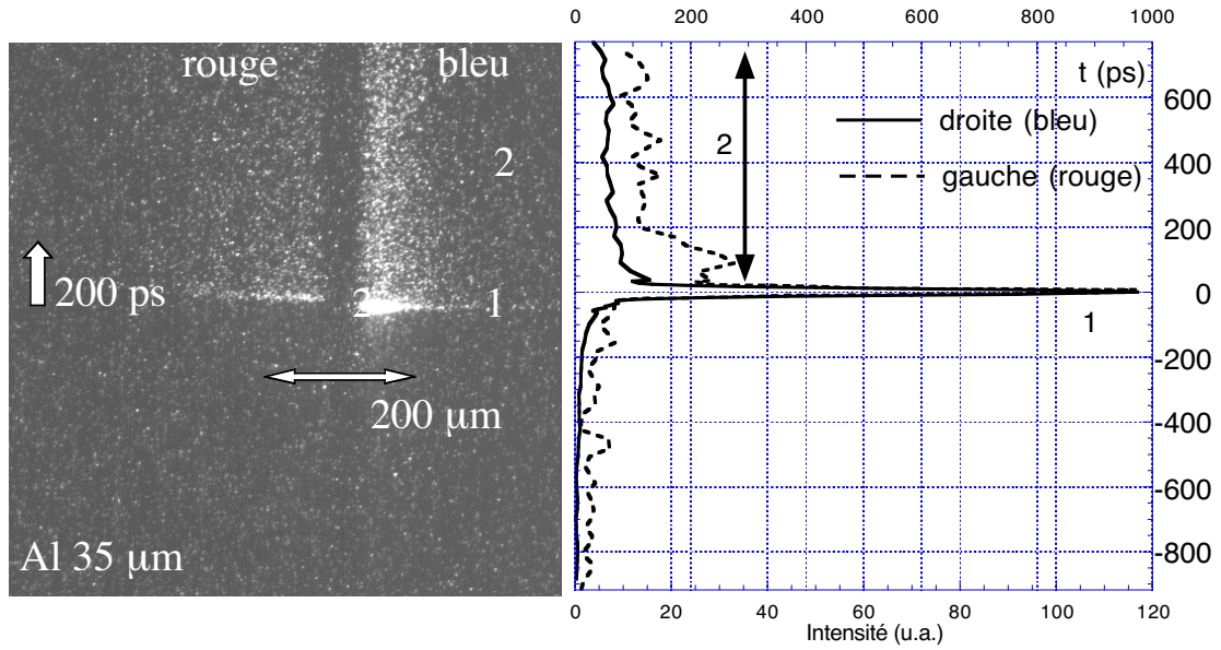
FIG. 3.36 – Images "rapides" d'émissivité d'une cible d'aluminium ( 35\mu m , 4J ), avec le double filtre rouge-bleu qui divise l'image en deux. A droite : profil rouge (pointillé) et bleu (continu).
