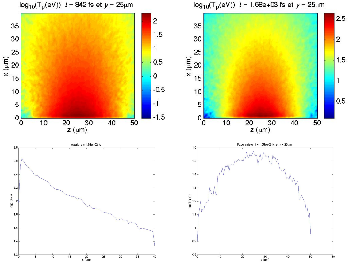
FIG. 5.24 – Simulation sans champs électromagnétiques, pour une cible d'aluminium de 40\mu\text{m} . Carte de température et profils axial et radial (en face arrière) correspondants. Mêmes paramètres que figure 5.15 et 5.16.
