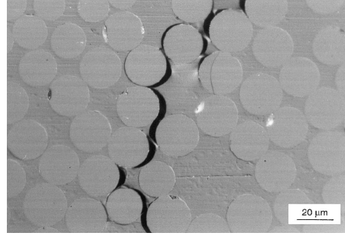
Fig. 1.7: Coalescence en une microfissure - source [Gamstedt et Sjogren, 1999]
