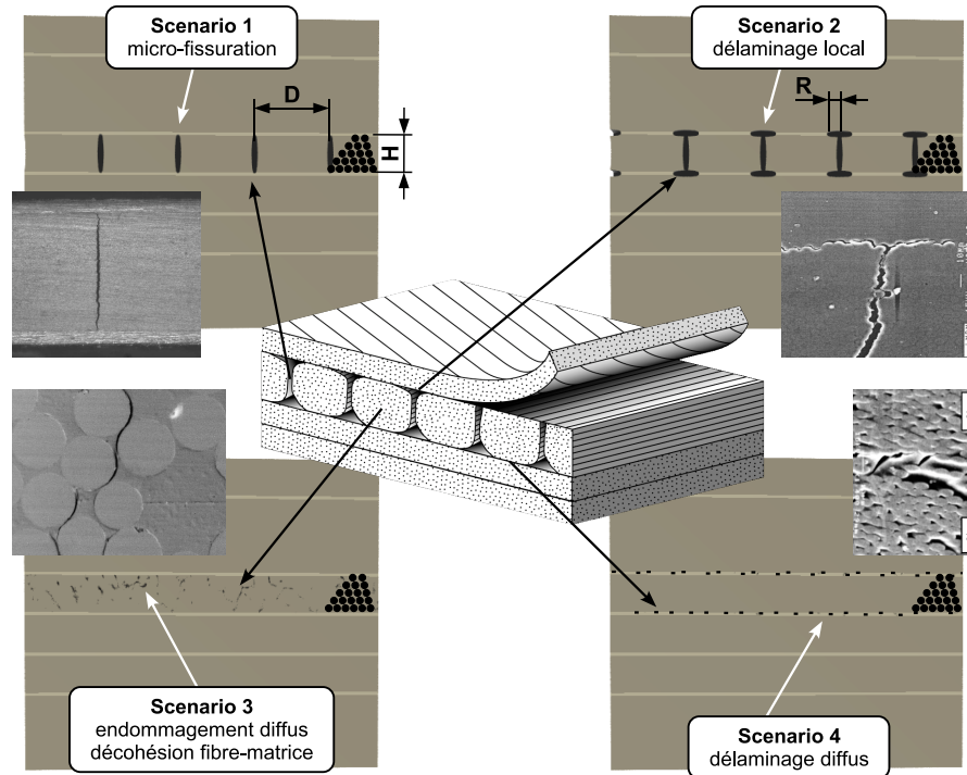
Fig. 2.2: Les quatre scénarios majeurs de dégradation pris en compte dans la procédure micro-méso
