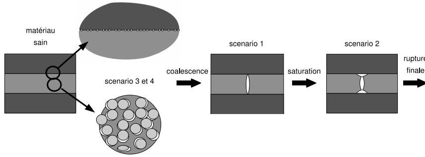
Fig. 2.3: Enchainement des quatre scénarios de dégradation
