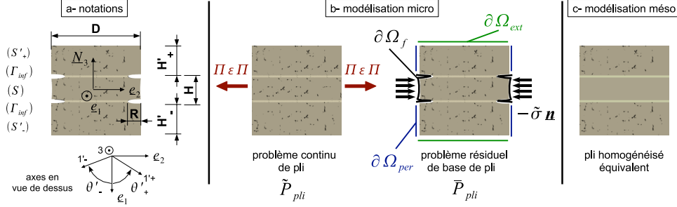
Fig. 5.1: Problème de base de pli \bar{P}_{pli}
