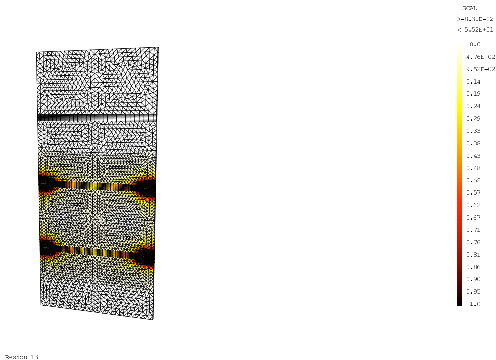
Fig. A.4: Localisation de l'énergie pour le résidu 13 ( \rho = 0.5, \tau = 0.23 )
