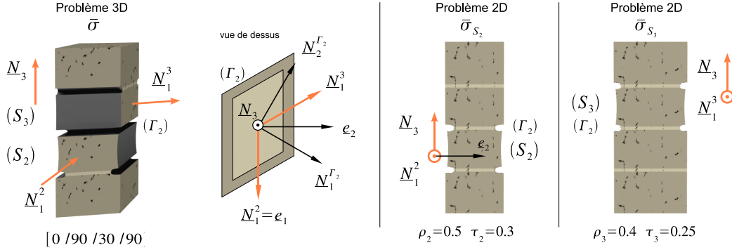
Fig. 3.2: Approximation de la solution résiduelle 3D par deux solutions 2D
