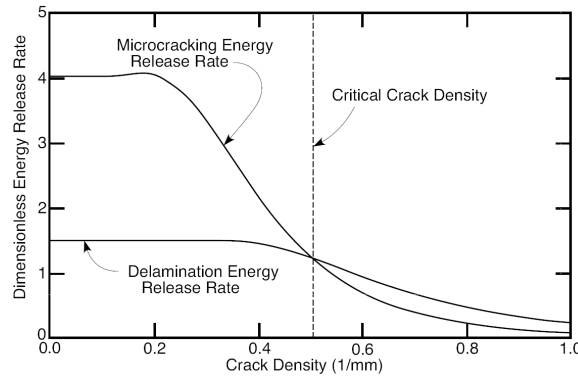
Fig. 1.16: Taux de restitution d'énergie adimensionné pour l'initiation du délaminage local et pour l'évolution de la micro-fissuration en fonction de la densité de micro-fissure - source Nairn, stratifié carbone/epoxy [0_2/90_4]_s
