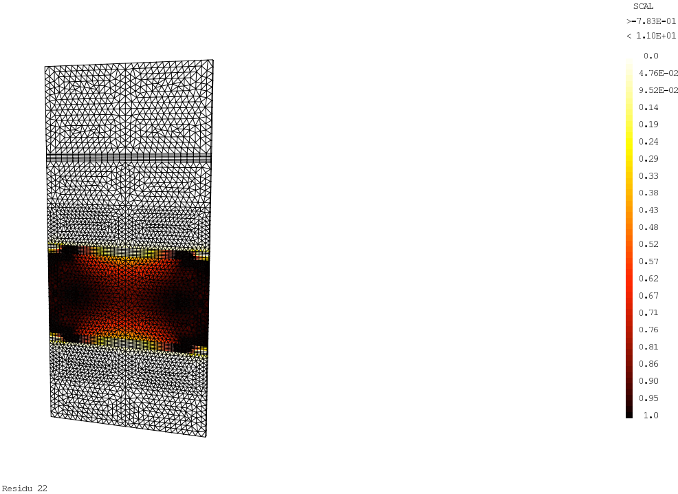
Fig. A.1: Localisation de l'énergie pour le résidu 22 ( \rho = 0.5, \tau = 0.23 )
