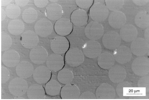
Fig. 1.6: Décohesions fibres-matrice dans un verre/epoxy - source [Gamstedt et Sjogren, 1999]
