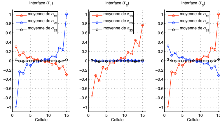
Fig. 4.9: Interfaces : moyenne des composantes hors-plan de la contraintes
