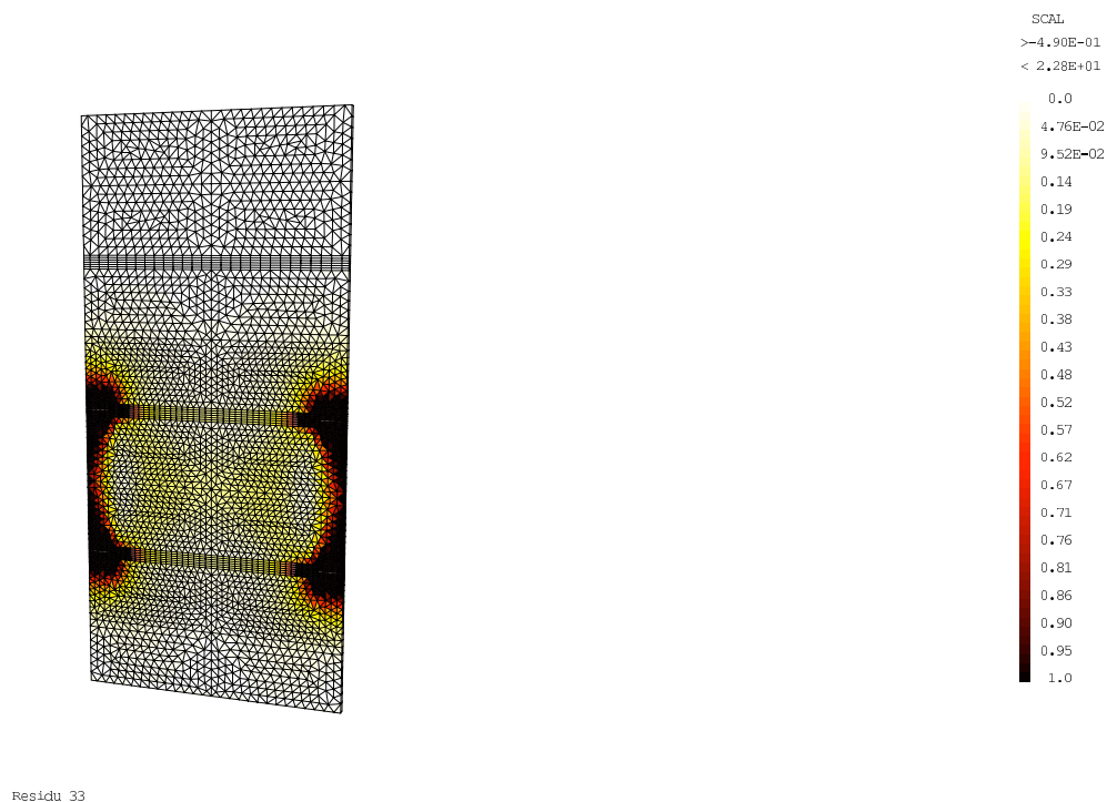
Fig. A.5: Localisation de l'énergie pour le résidu 33 ( \rho = 0.5, \tau = 0.23 )
