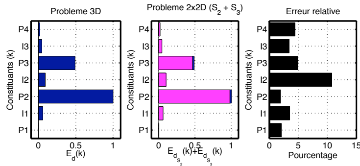
Fig. 3.7: Chargement plan – comparaison entre le calcul 3D et l'approximation 3D \approx 2 \times 2D de l'énergie de déformation résiduelle pour les quatres plis et les trois interfaces de la cellule élémentaire
