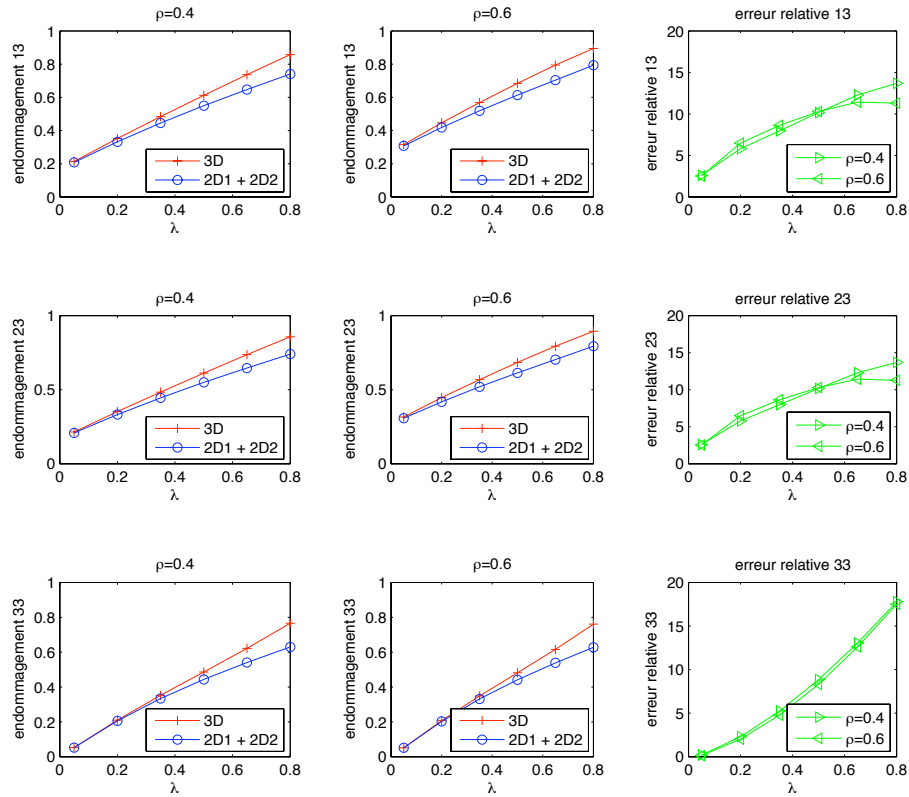
Fig. C.2: Comparaison entre solution 3D et approximation 2 \times 2D en fonction de l'état de dégradation de la cellule
