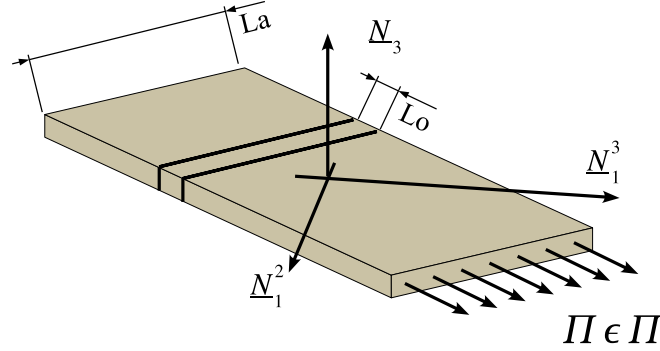
Fig. 4.1: Eprouvette [67, 5/ - 45/45/ - 67, 5]_s soumise à un essai de traction – notations
