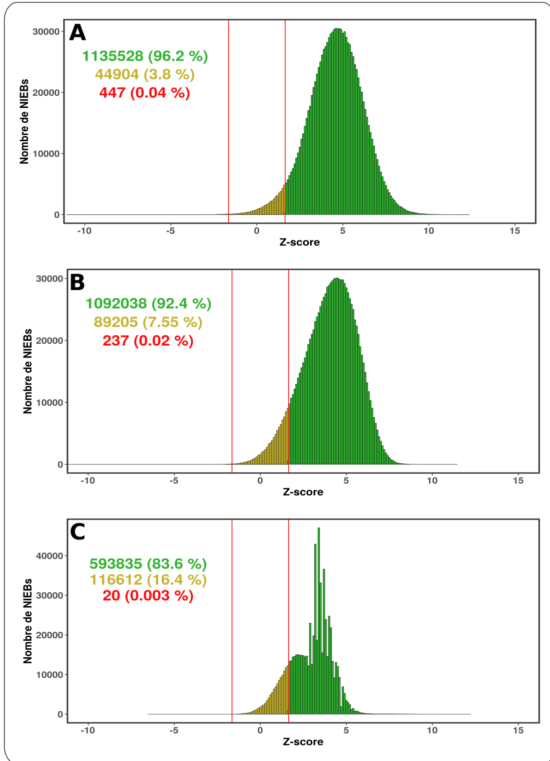
FIGURE 3.2 – Distributions des z-scores des barrières nucléosomales chez l'humain obtenues à partir des données expérimentales de Valouev et Mieczkowski. Les z-scores ont été obtenus selon la méthode détaillée en Partie 3.2.1 . Les figure A, B et C représentent respectivement les résultats obtenus avec les données de Valouev in vivo , Valouev in vitro et Mieczkowski. La couleur verte représente les z-scores traduisant une déplétion significative en nucléosomes à l'intérieur des barrières par rapport à leurs bords. La couleur rouge représente les z-scores traduisant un enrichissement significatif des nucléosomes à l'intérieur des barrières. La couleur jaune représente les z-scores ne traduisant pas d'enrichissement significatif ni à l'intérieur ni à l'extérieur des barrières. Les barres verticales rouges représentent les seuils de significativité au risque 5 % (−1.645 et 1.645). Les NIEBs utilisés pour le calcul sont distant d'au moins 300 pb de leurs deux voisins et ne sont considérées que les régions (NIEB + régions flanquantes) avec au moins 10 lectures alignées. Le nombre et la proportion de barrières dans chaque catégorie sont indiqués en suivant le même code de couleur.
